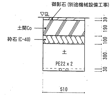
施工前 管路撤去掘削断面図① 1:20
