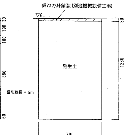
施工後 管路撤去掘削断面図③ 1:20
