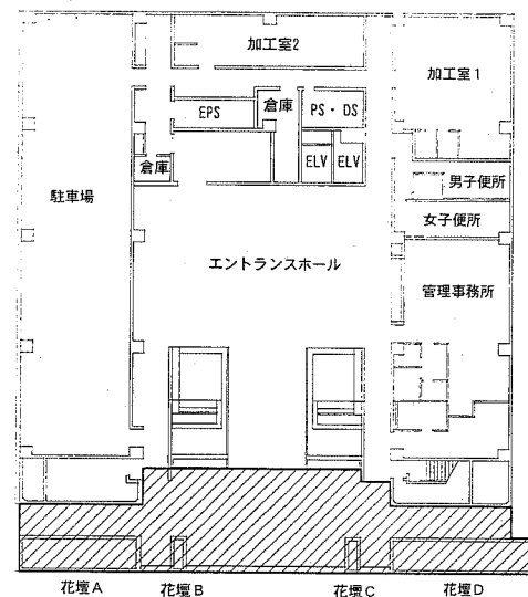
2階 配置図 1:400
