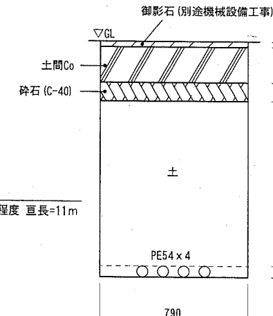
施工前 管路撤去掘削断面図③ 1:20
