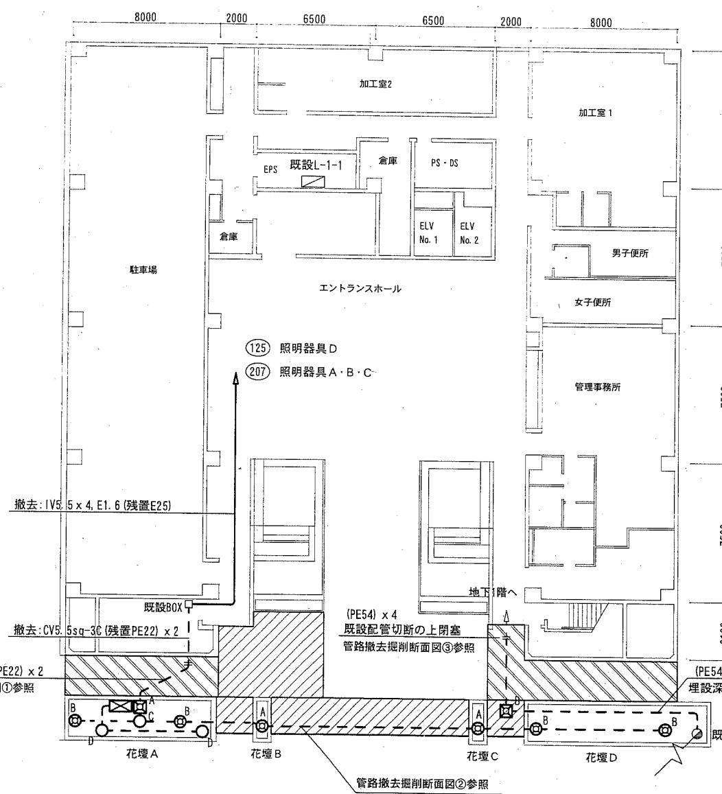
1階 撤去図 1:200
