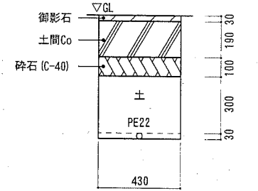
施工前 管路撤去掘削断面図② 1:20
