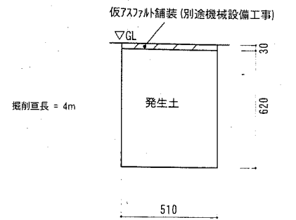
施工後 管路撤去掘削断面図① 1:20
