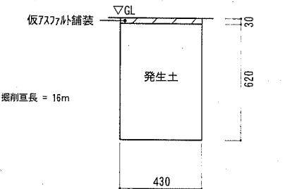
施工後 管路撤去掘削断面図② 1:20
