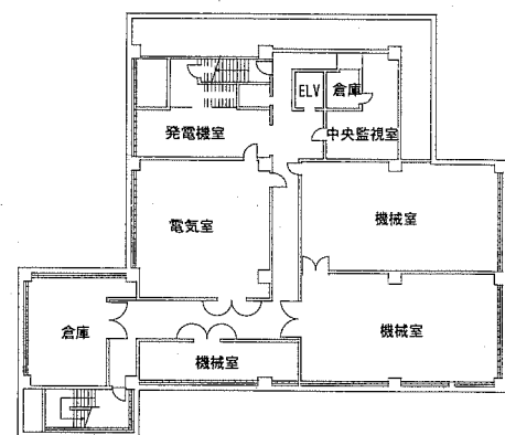
地下1階 配置図 1:400
