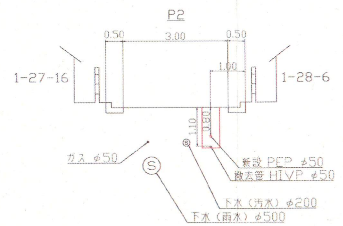
断面図 S=1/50
