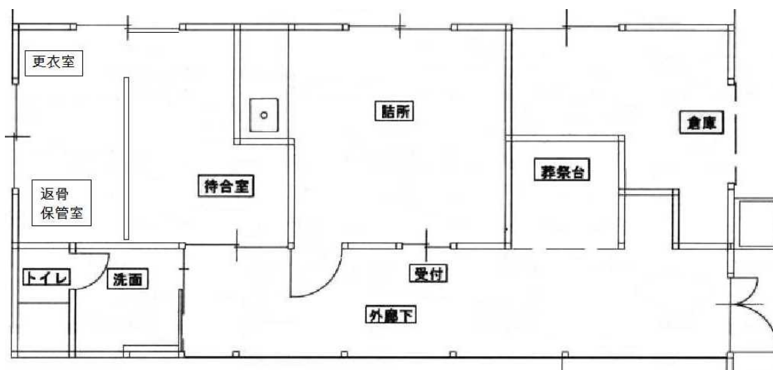
小動物焼却施設平面図
