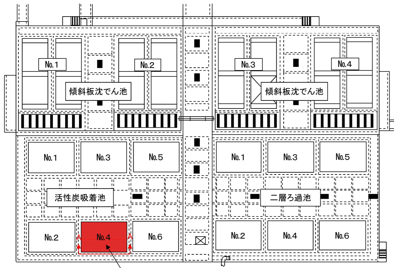
作業対象池 平面図
