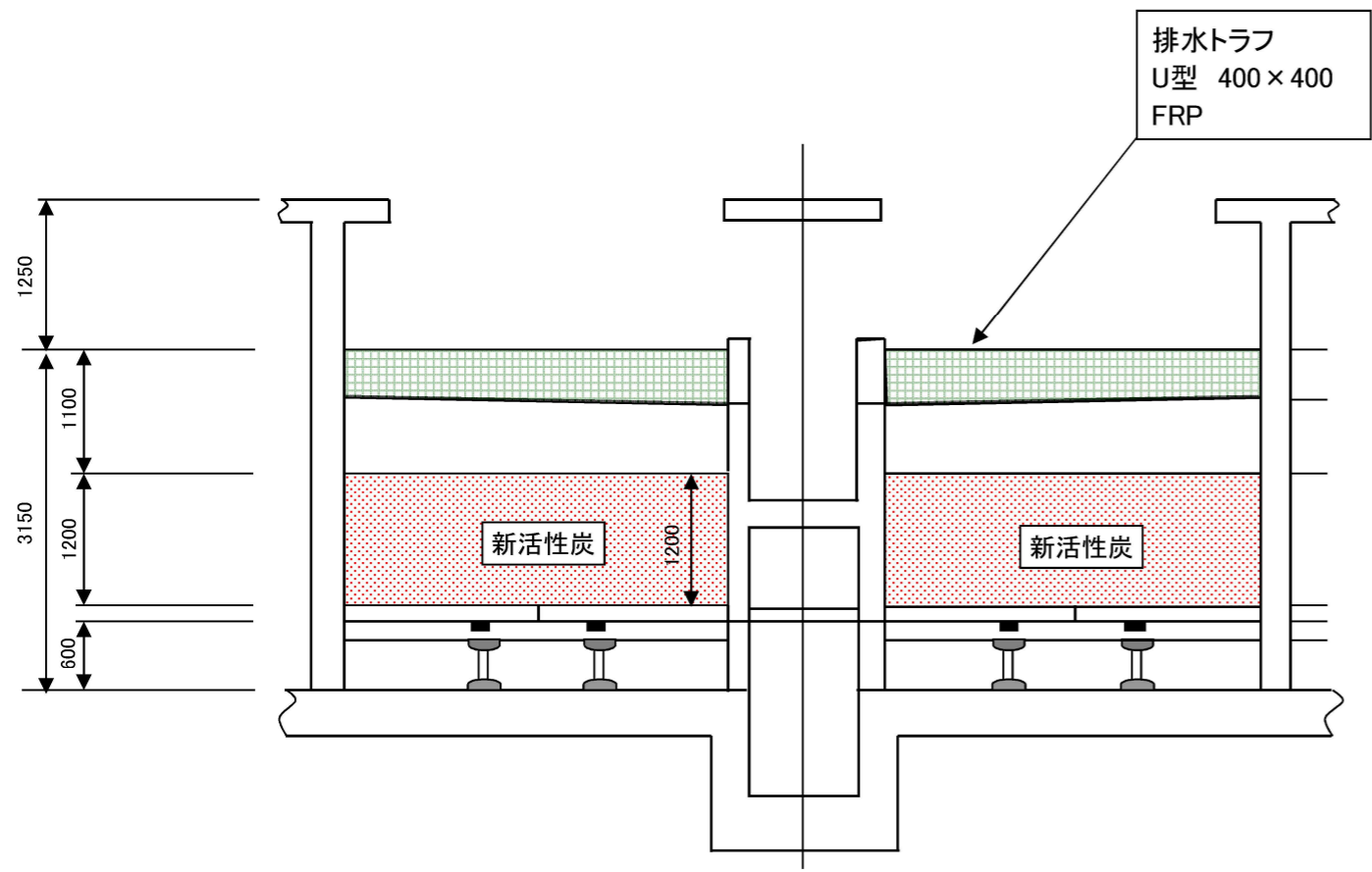
A-A 断面図
