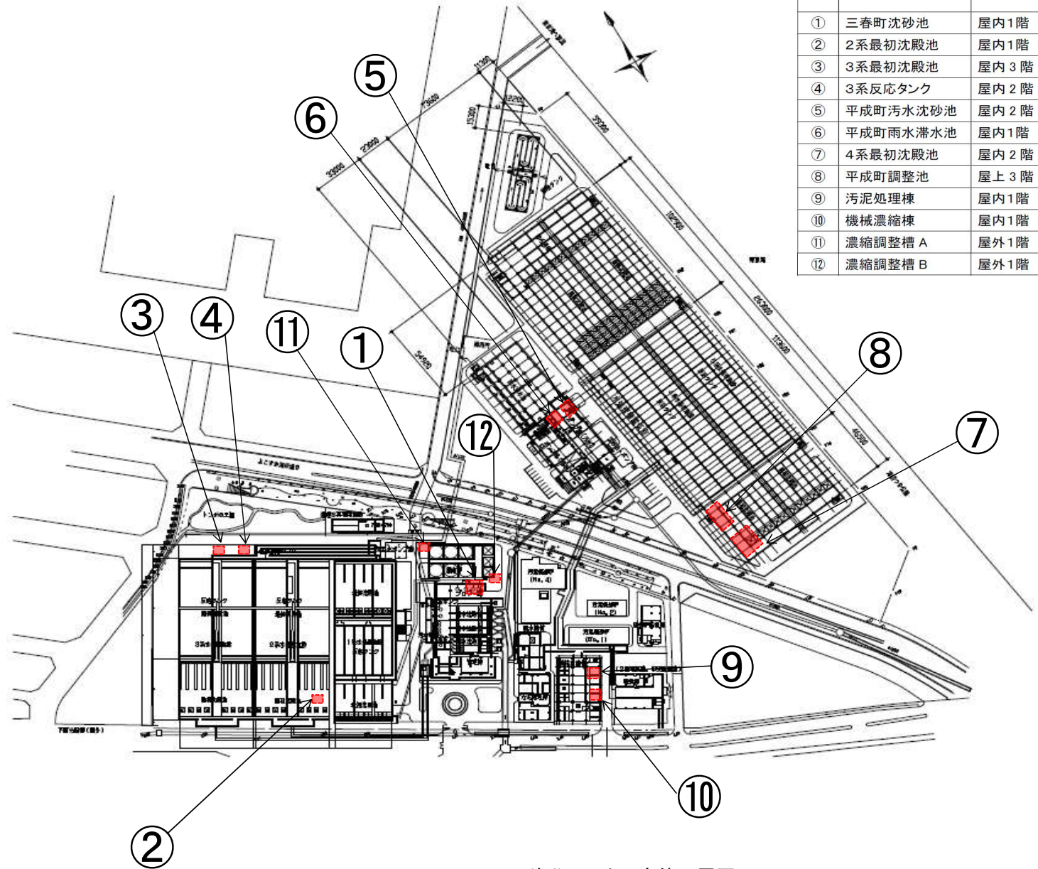
下町浄化センター全体配置図
