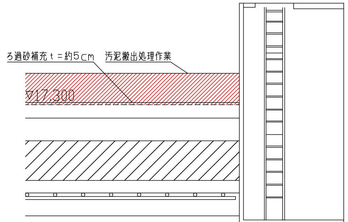
断面図 S=NON
