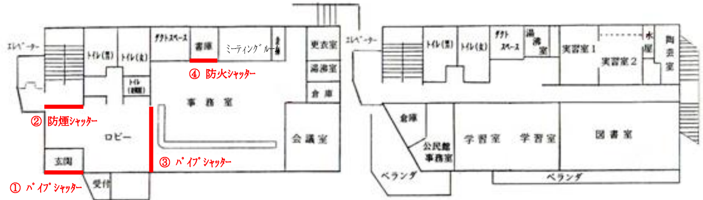
1階 (334.62㎡)
