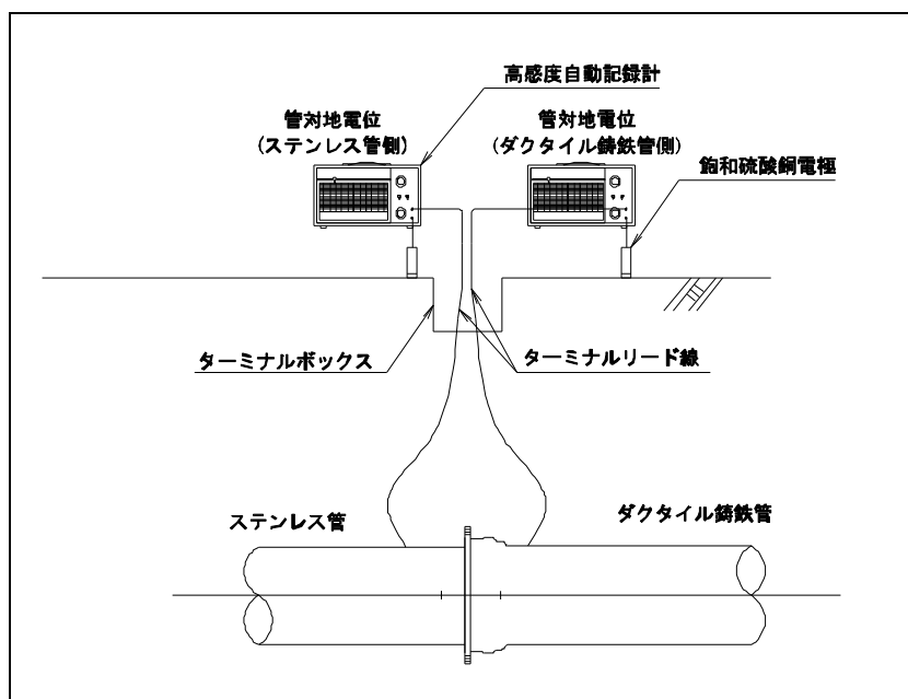
図 絶縁状態確認作業概要図
