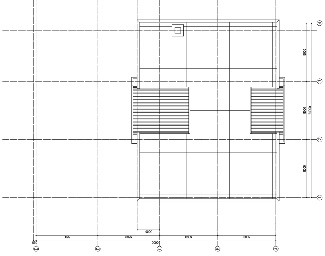
R階平面図 S=non
