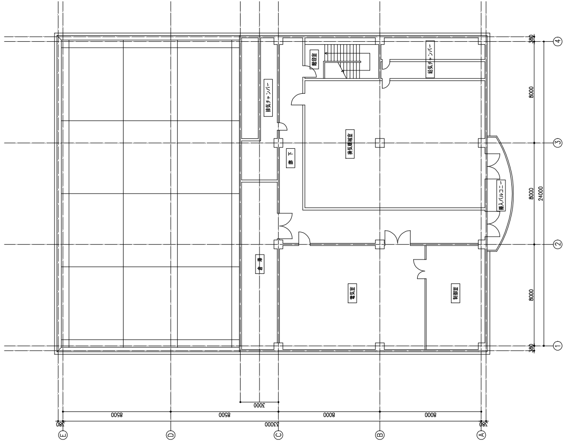
2階平面図 S=non
