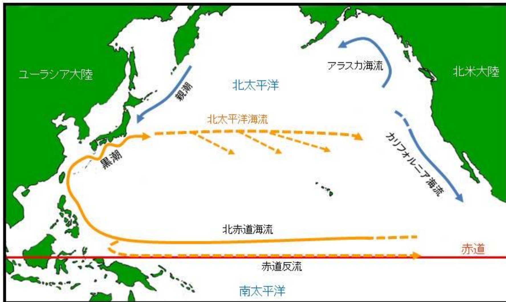
黒潮の源と北太平洋の海流
