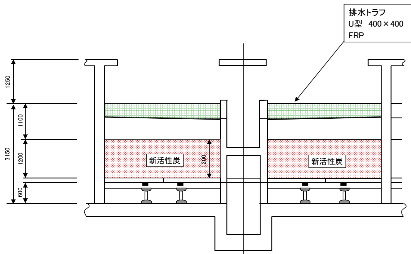
A-A 断面図
