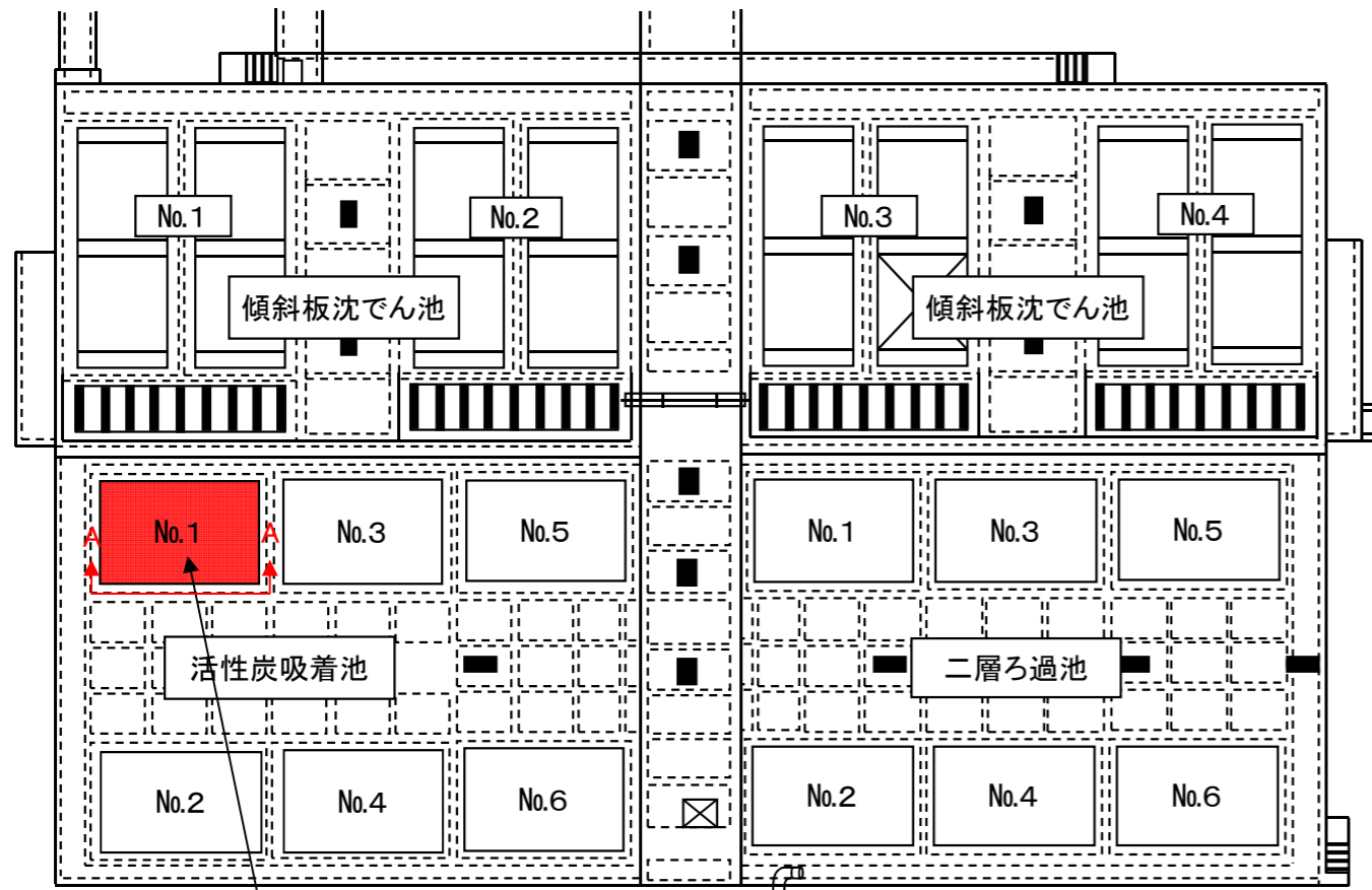
平面図
