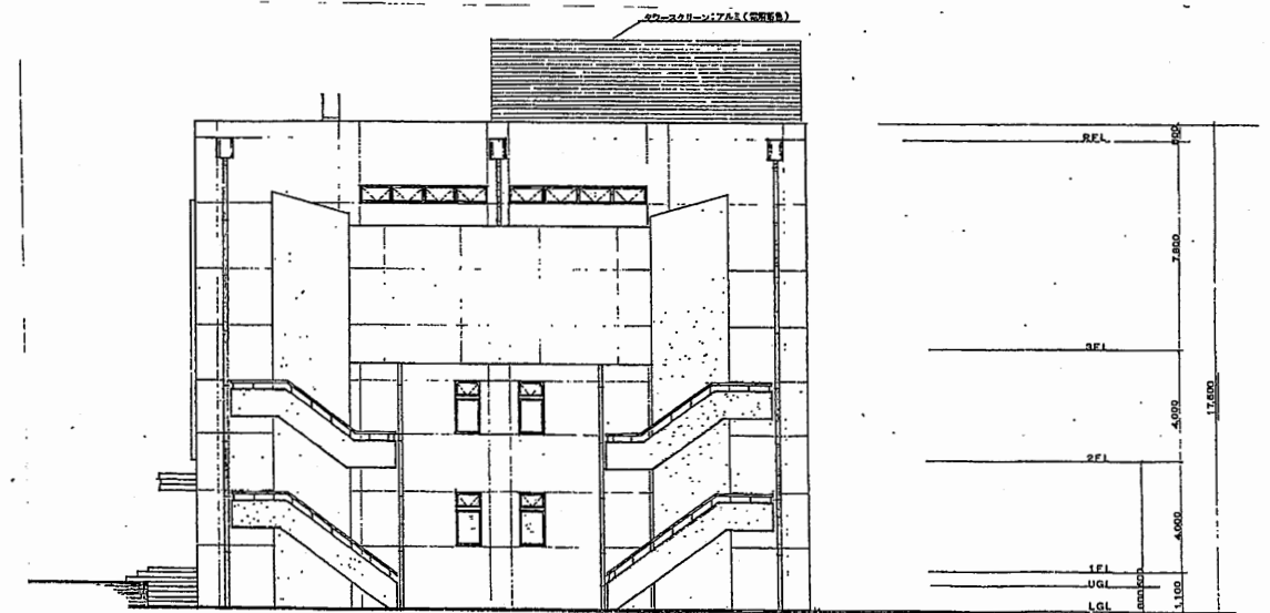
東側立面図 S1:1/100
