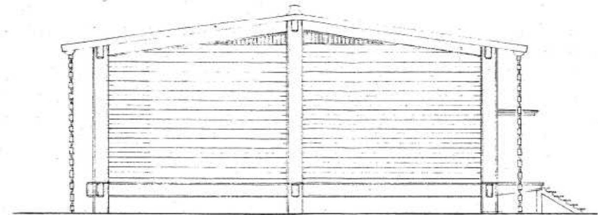
南立面図 1:100
