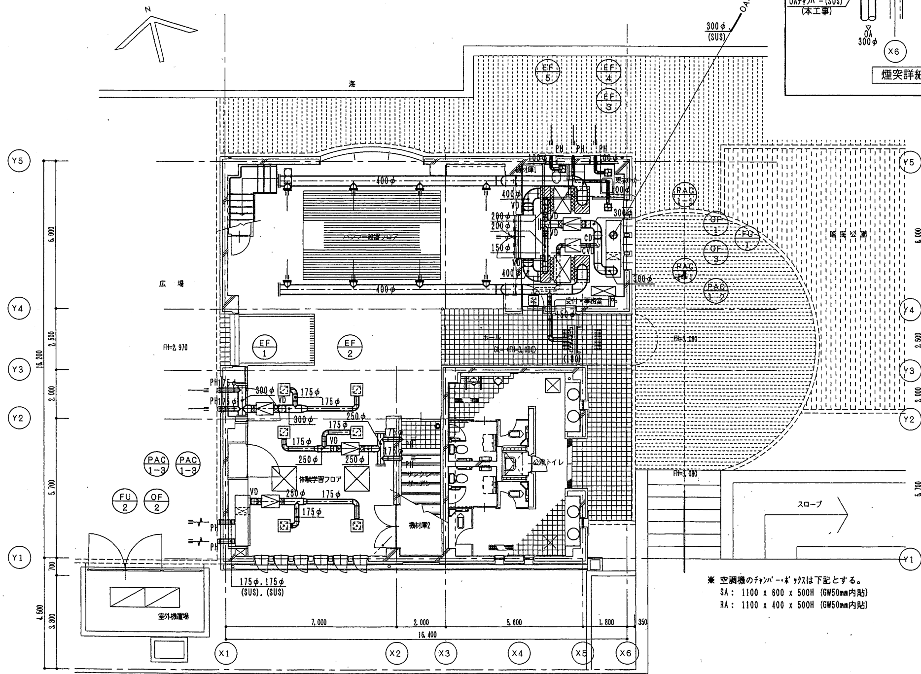
1階平面図
