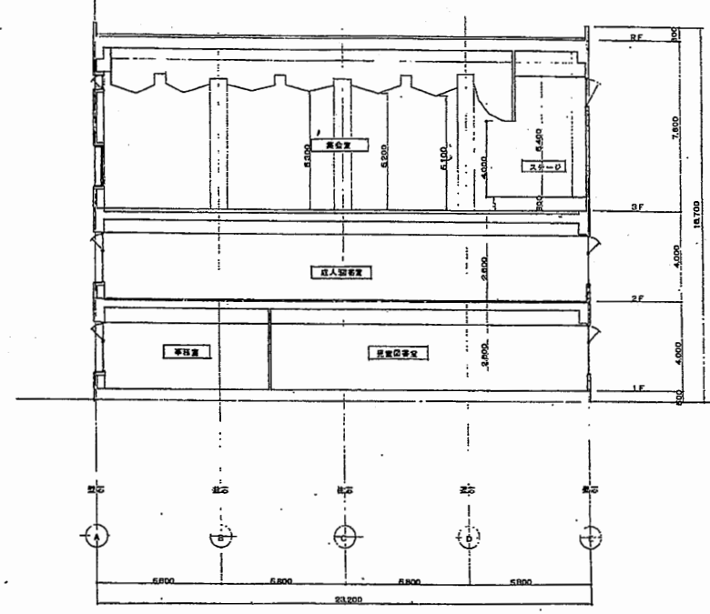
Y1-Y1断面図 1/100
