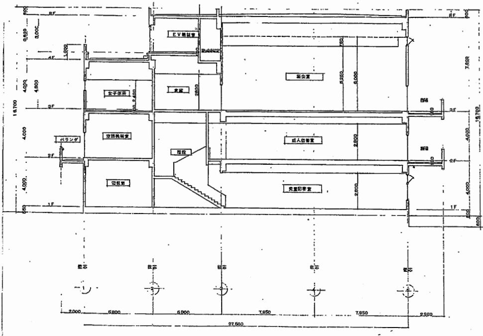
X1-X2断面図 1/100
