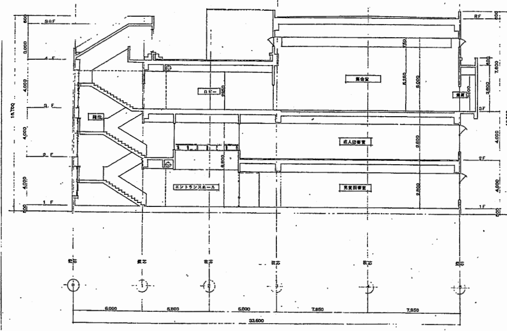
X1-X1断面図 1/100
