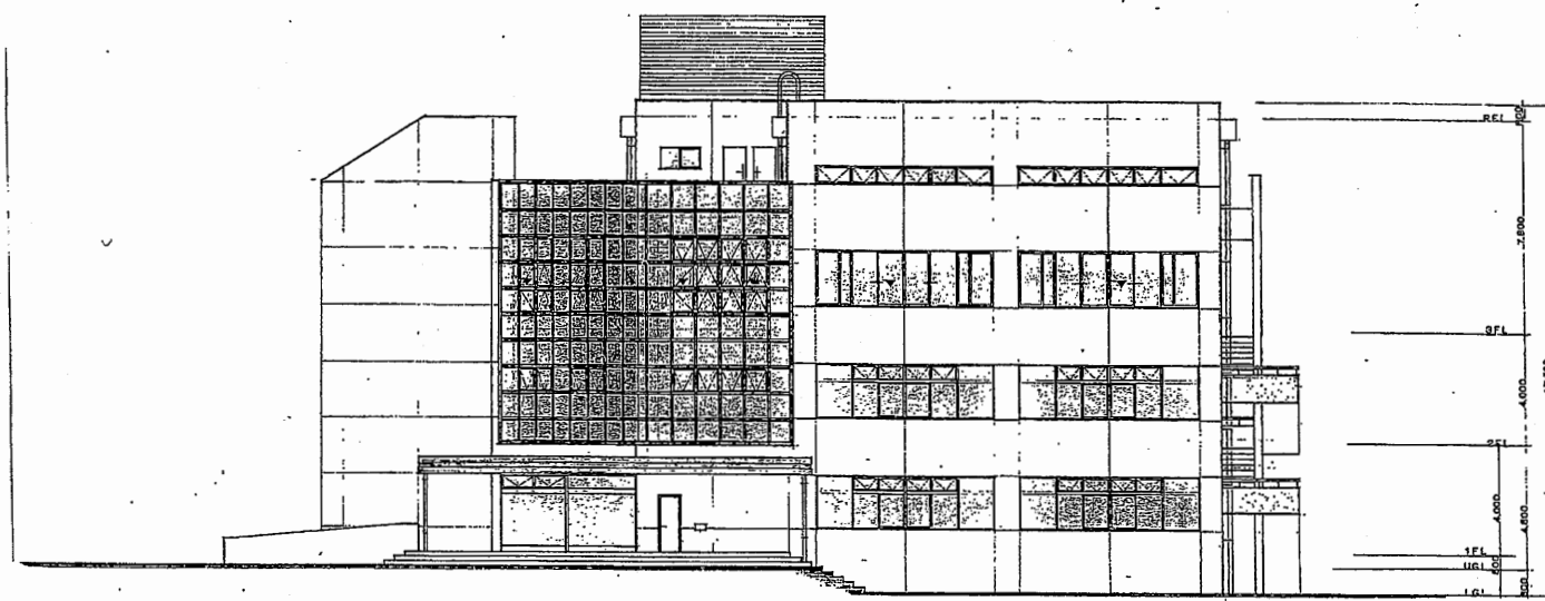
南側立面図 S1:1/100
