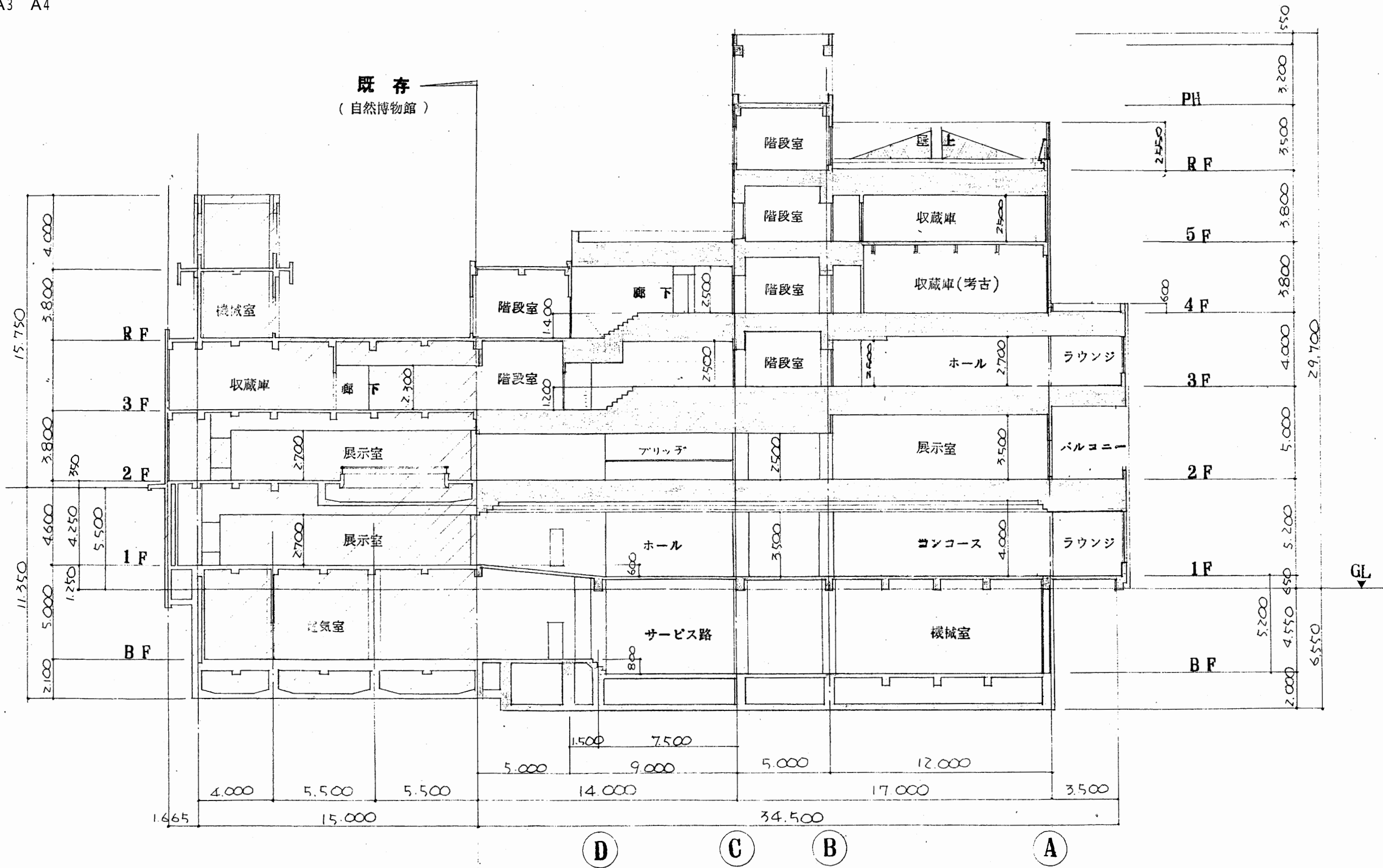
断面図 S 1:200
