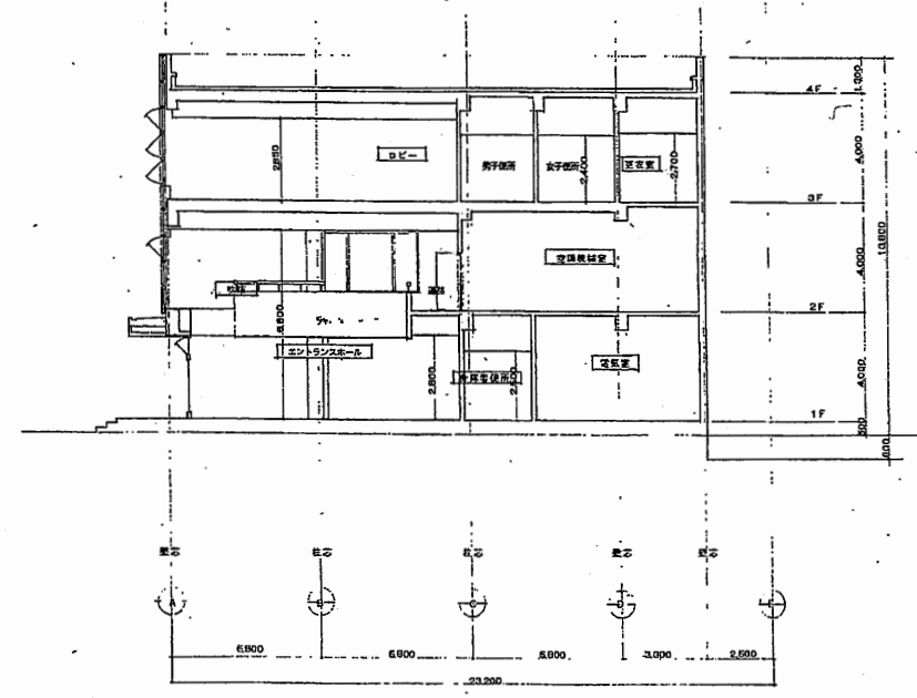
Y1-Y2断面図 1/100
