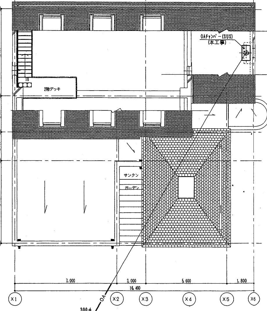
2階平面図
