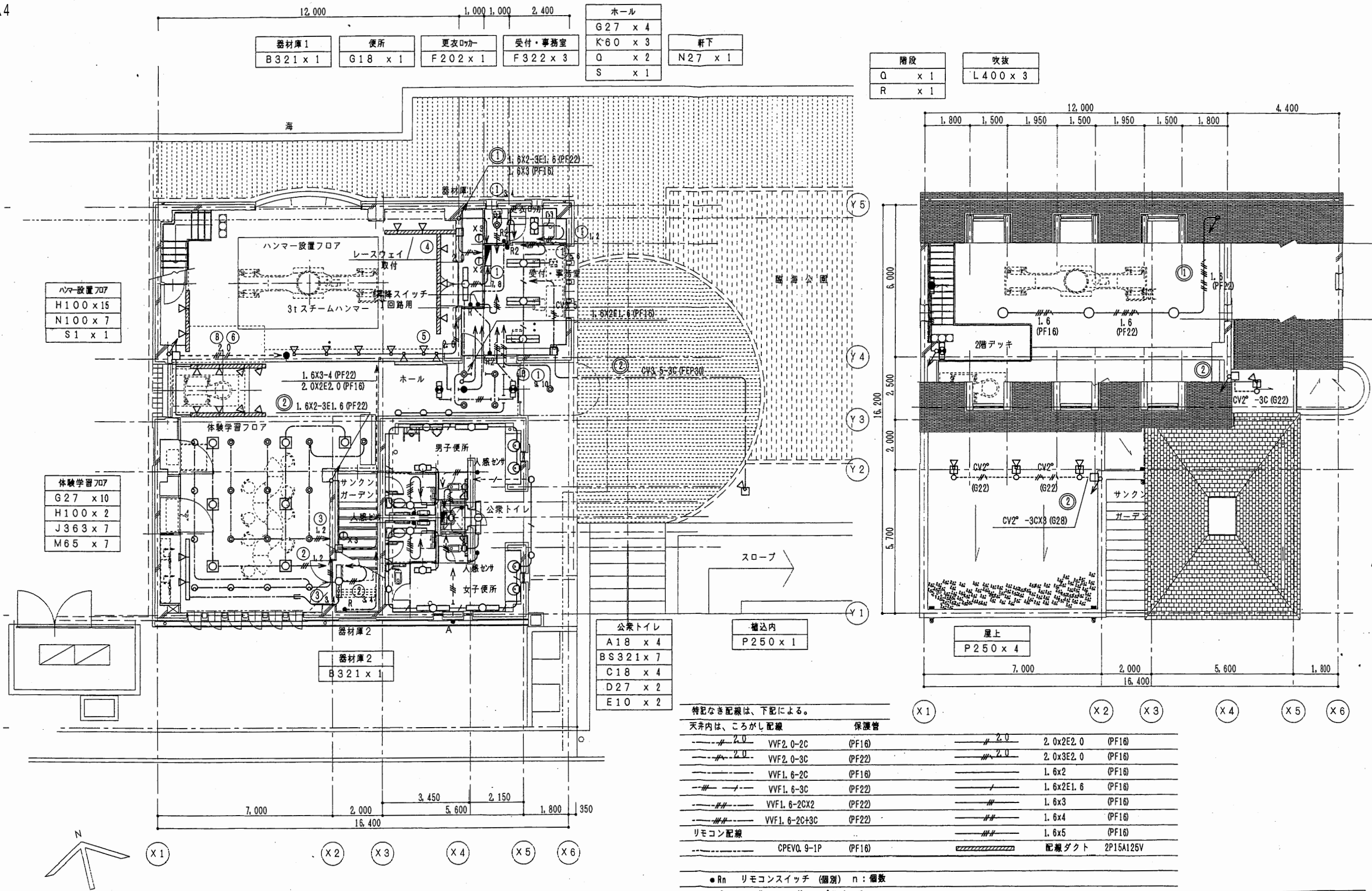
1階平面図
