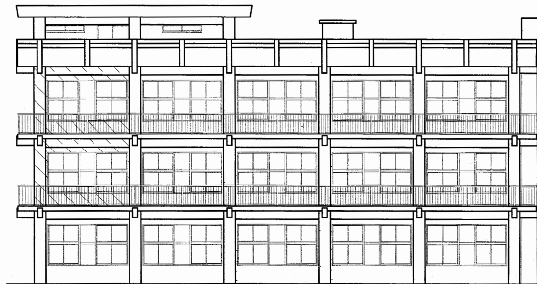
南側立面図
