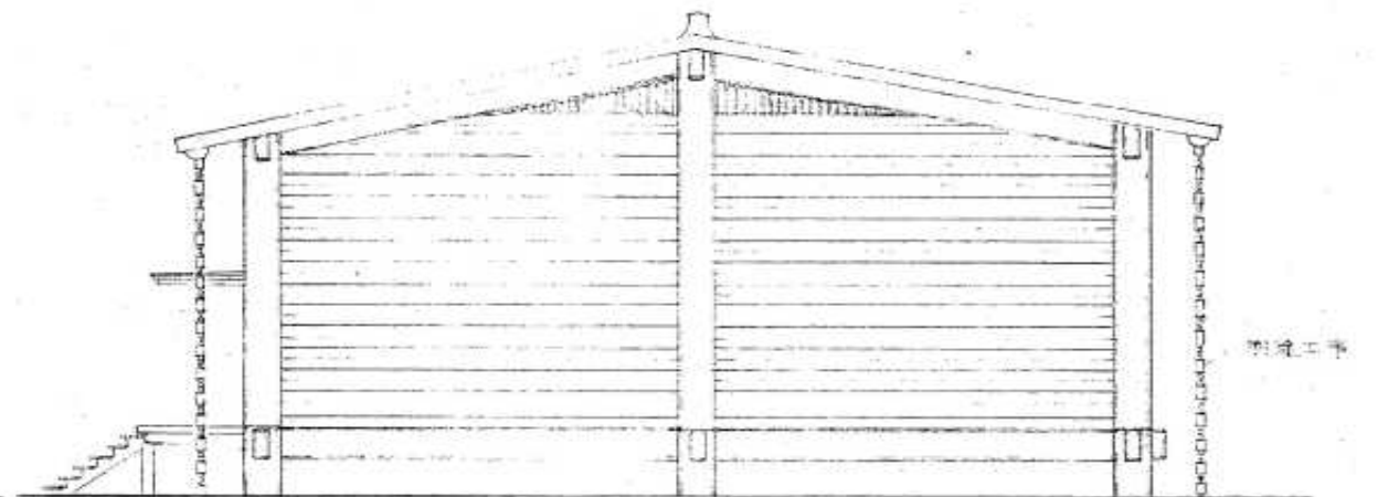
北立面図 1:100
