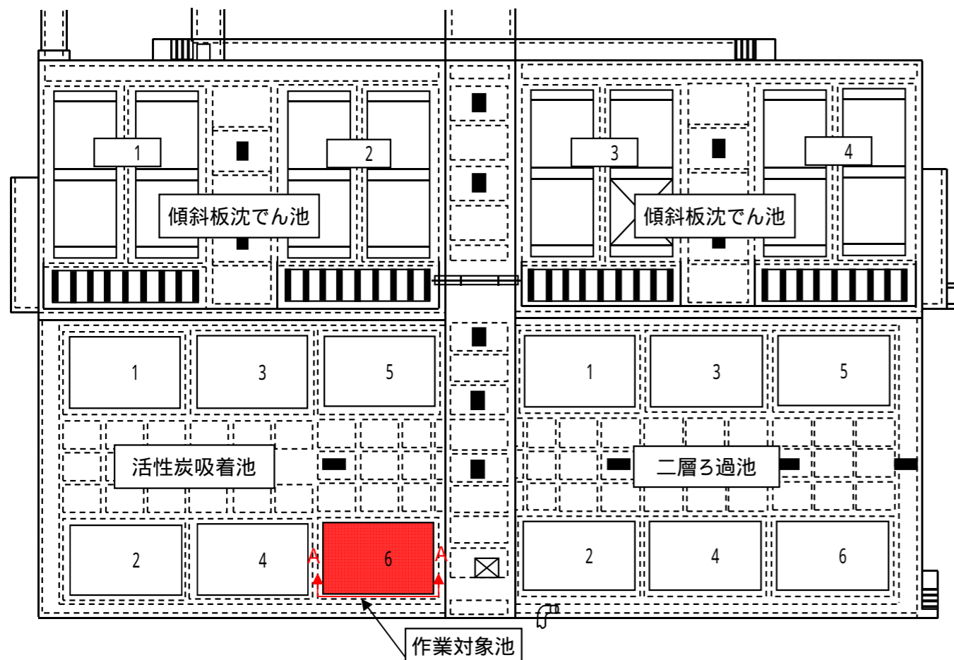
平面図
