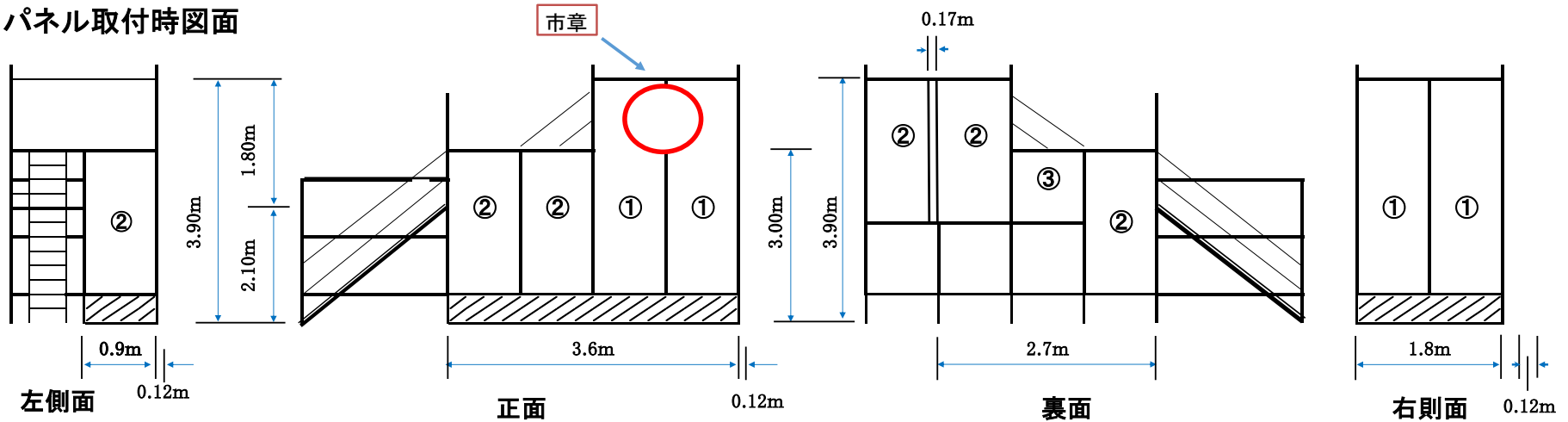
左側面図
