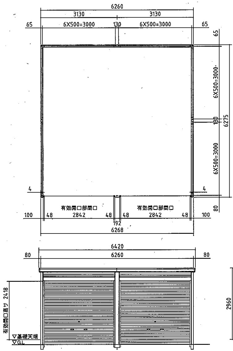
外形図 S=1/60(A3版)
