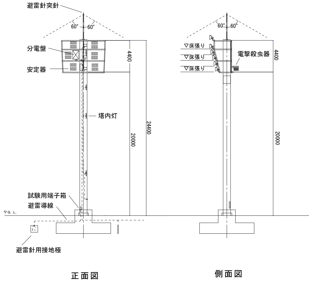
照明塔姿図
