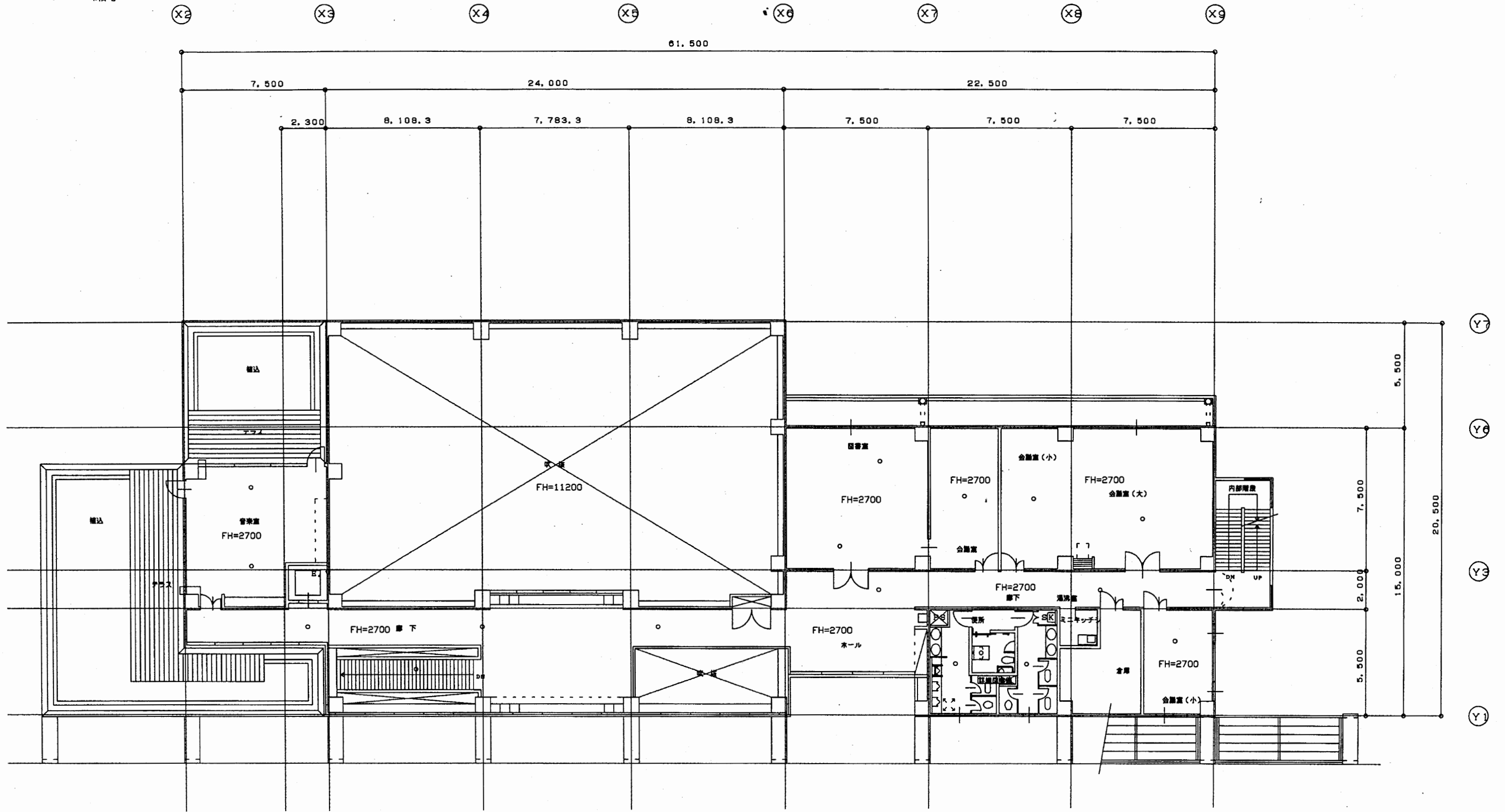
2階平面図 1:200
