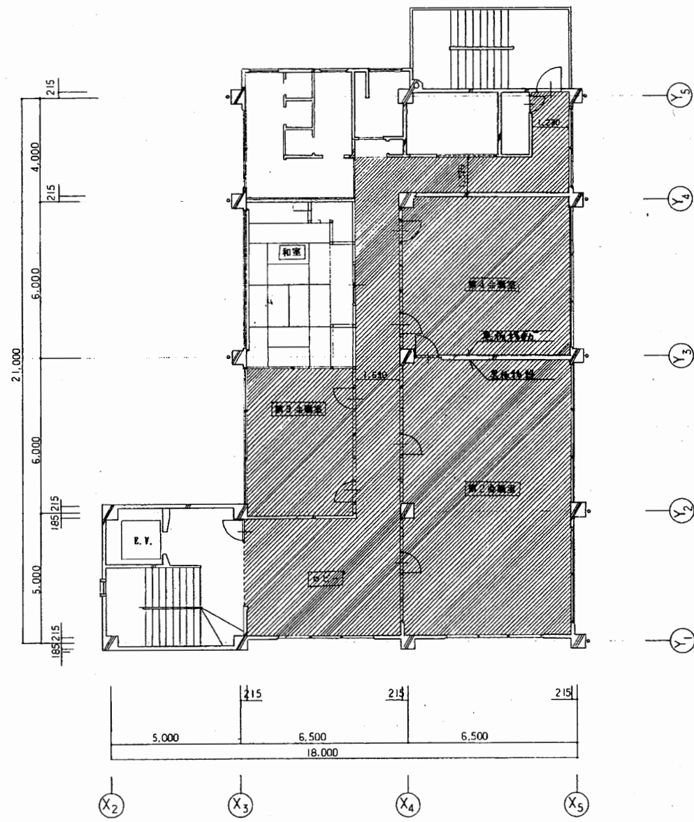
3階平面図 S 1:200
