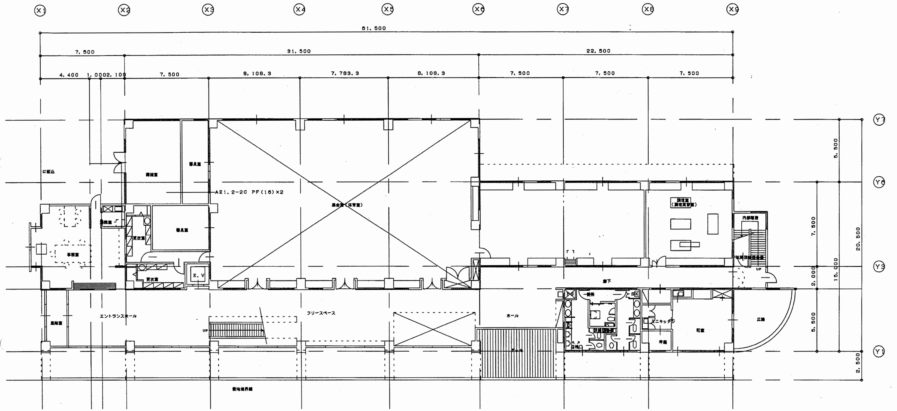
1階平面図 1:200
