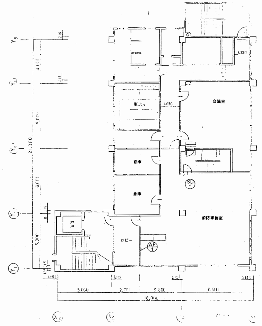
2階平面図 S 1:200
