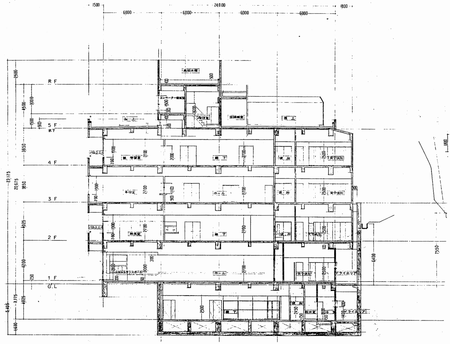
断面図 S 1:200
