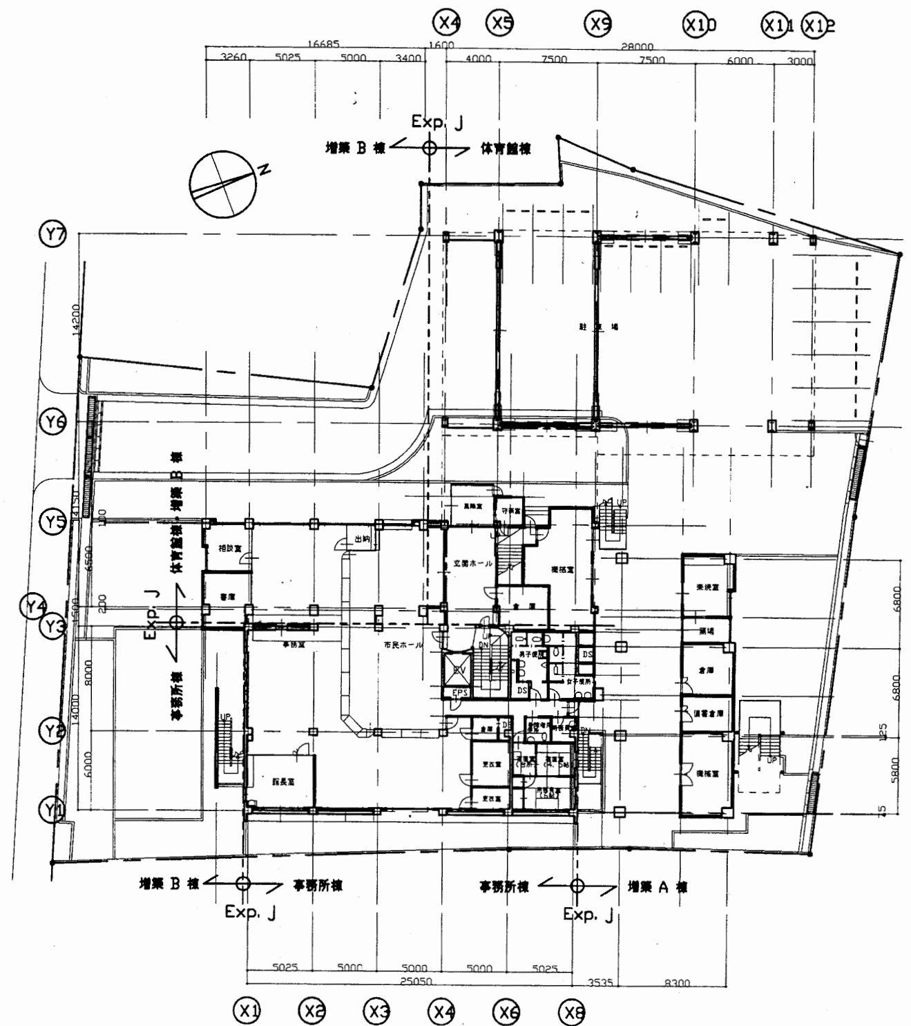
地下1階平面図 S1:400
