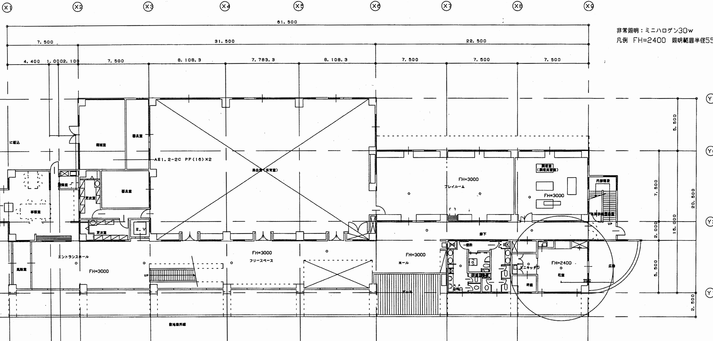
1階平面図 1:200
