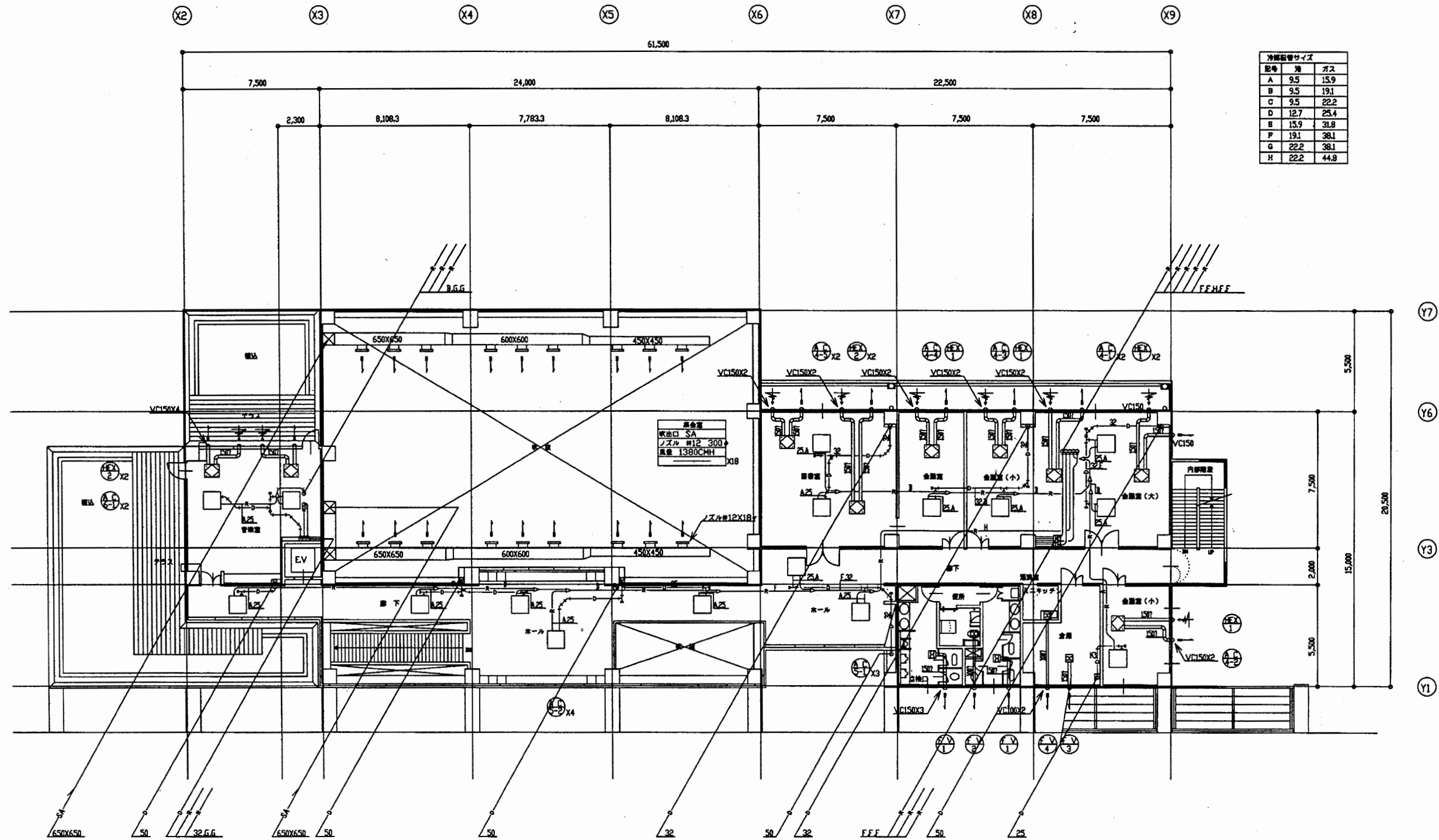
空調設備 2階平面図
