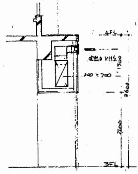
A-A断面詳細図 S=1/40
