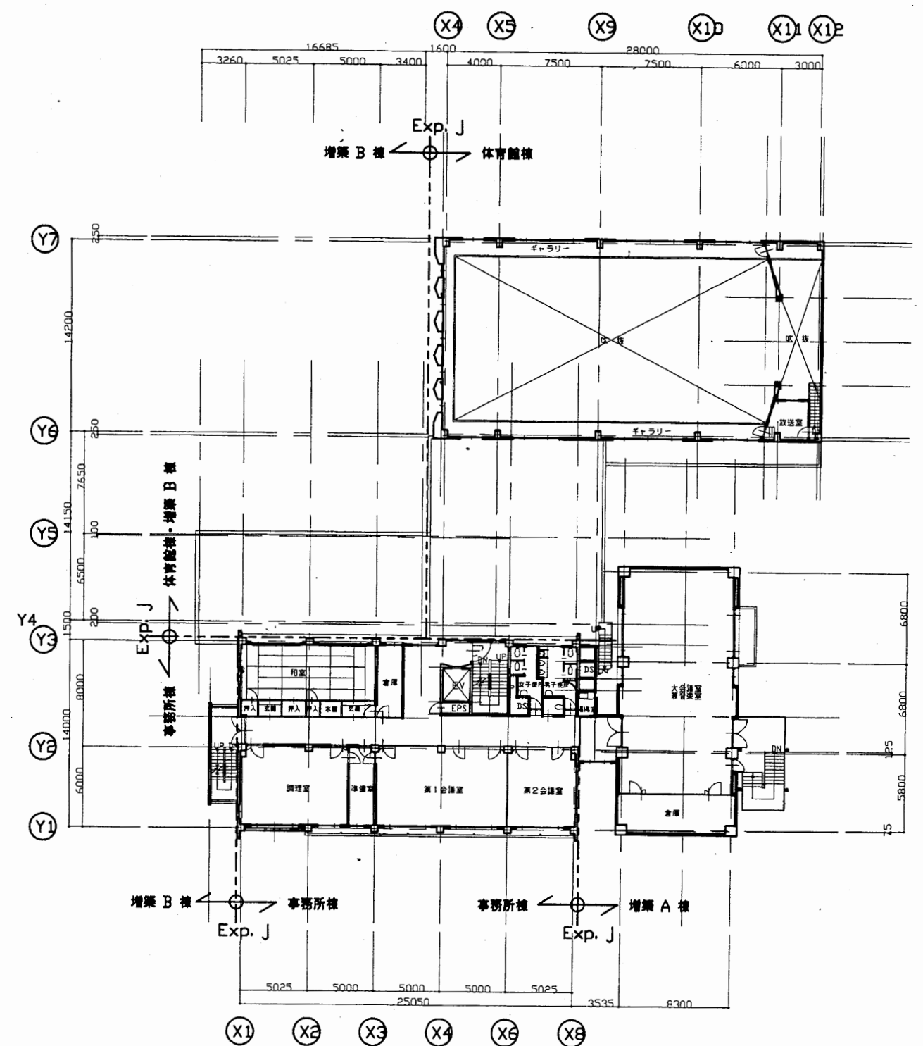
3階平面図 S1:400
