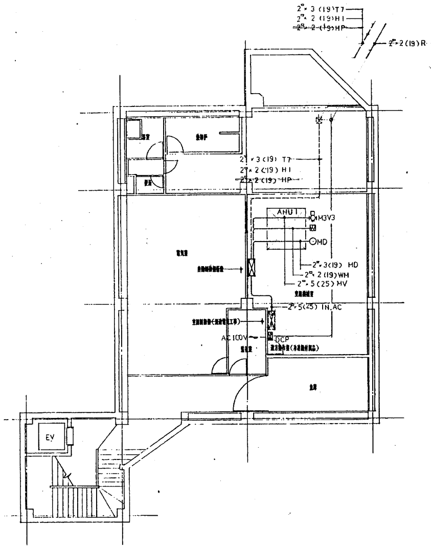
地層計装平面図 1:200
