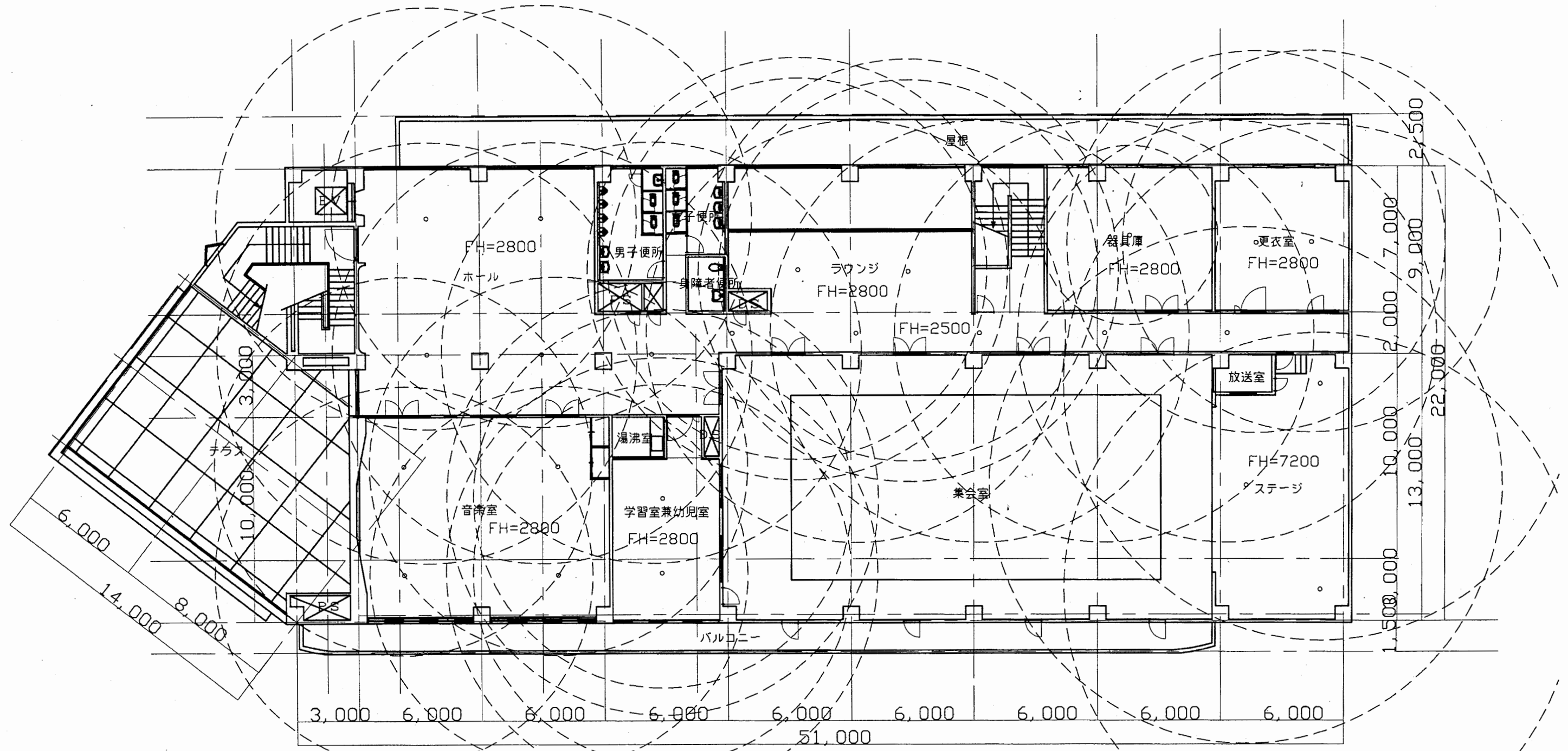
3階平面図 1:200
