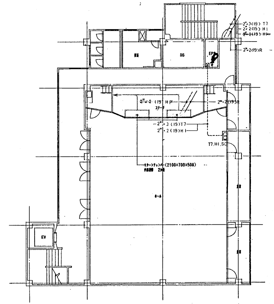
4層計装平面図 1:200
