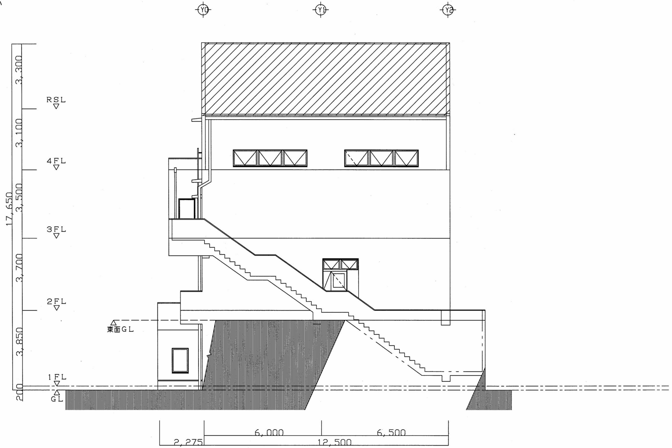
東側立面図 S=1/100
