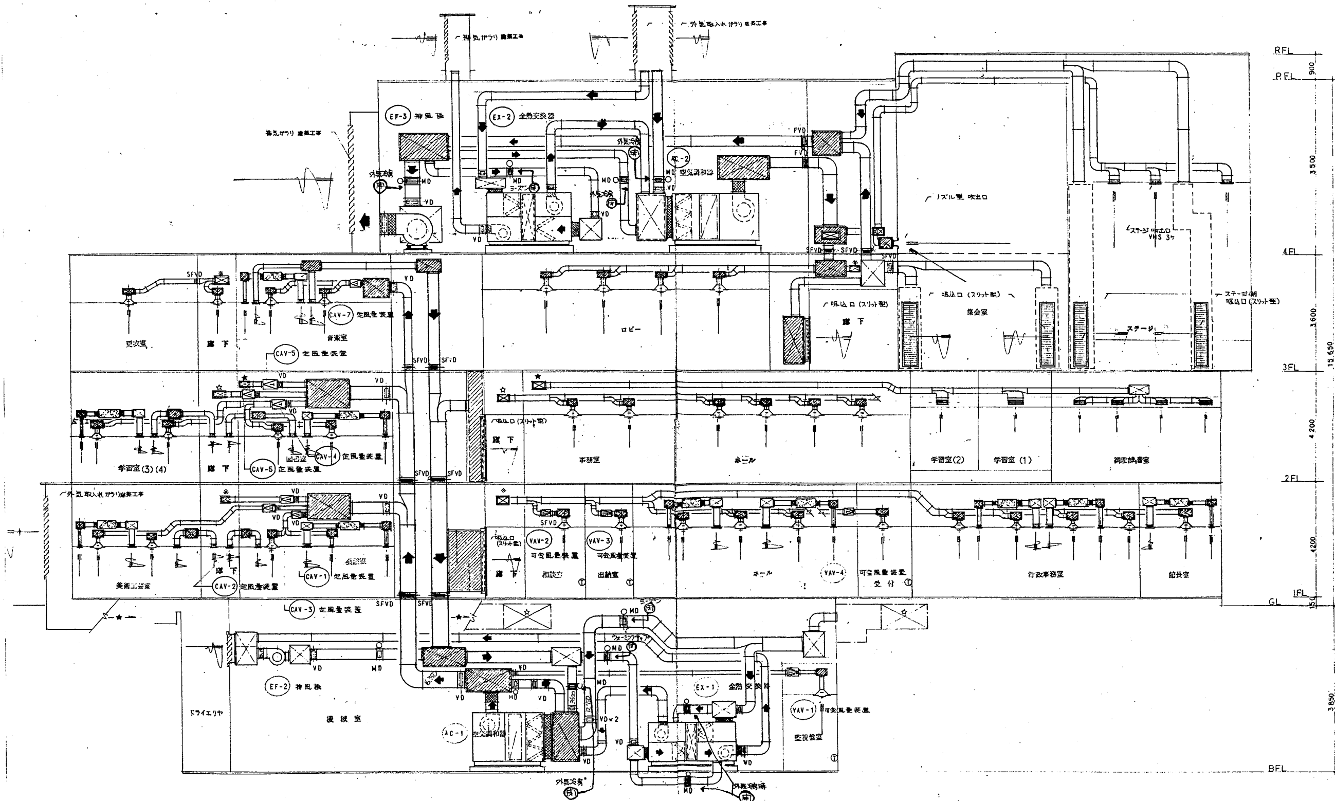
空調ダクト系統図
