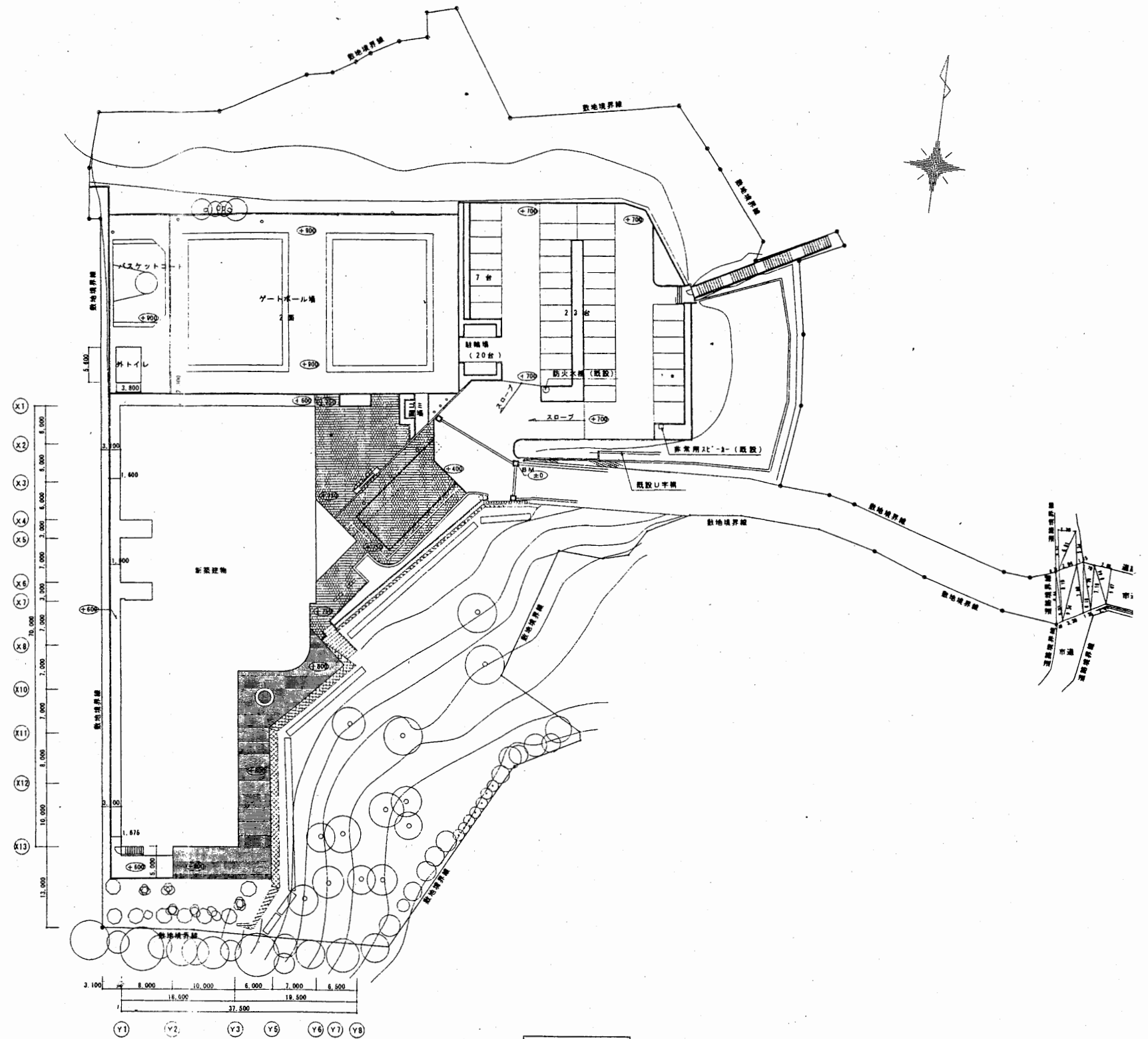
配置図
