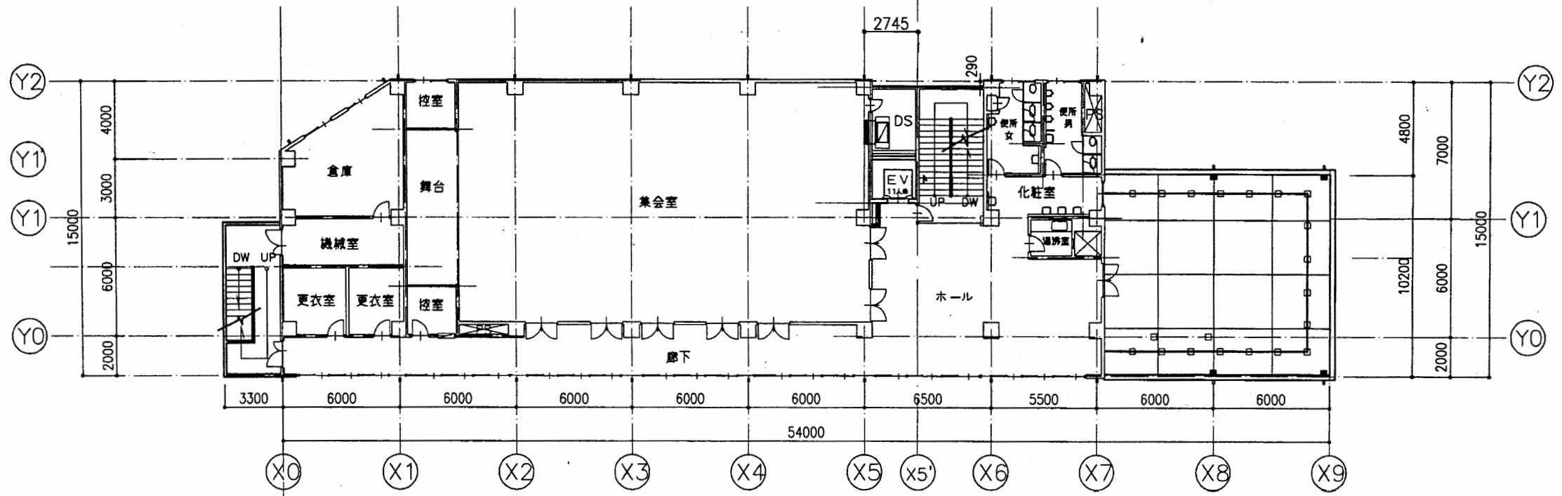
3階平面図 1:200
