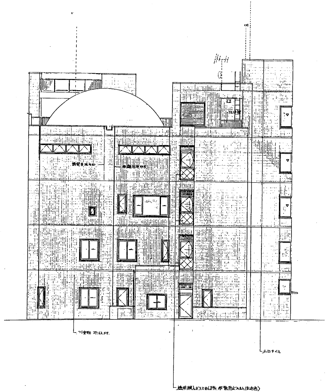
東側立面図 S 1:200
