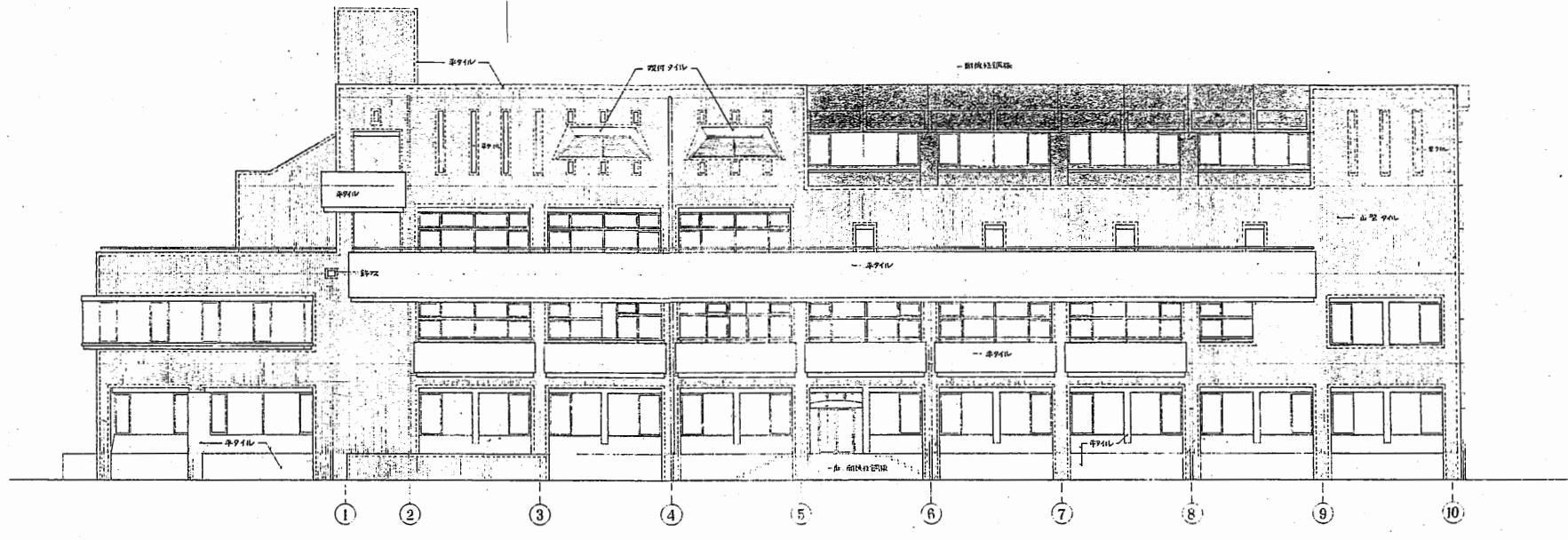
用立断面 1/100
