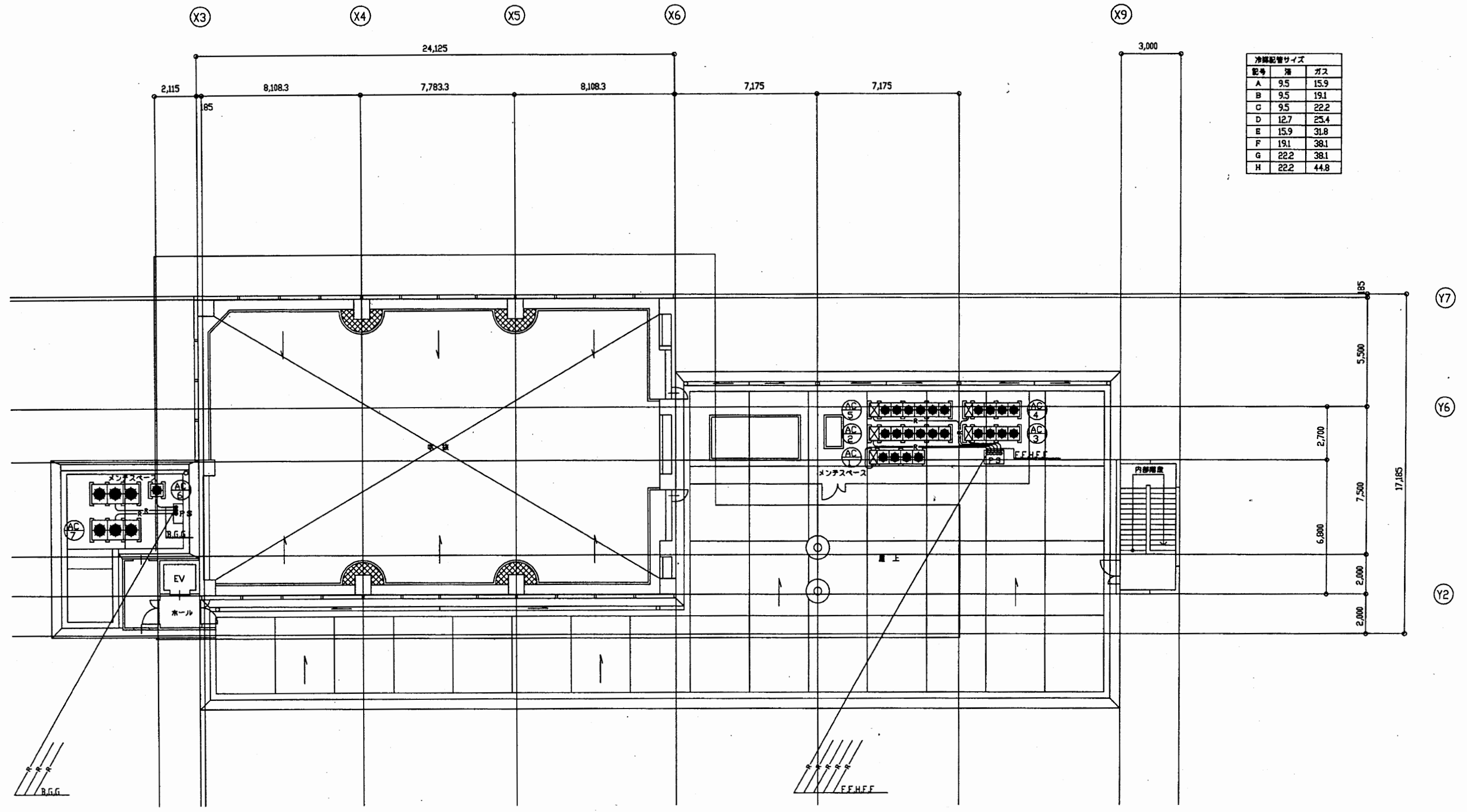
空調設備 R階平面図
