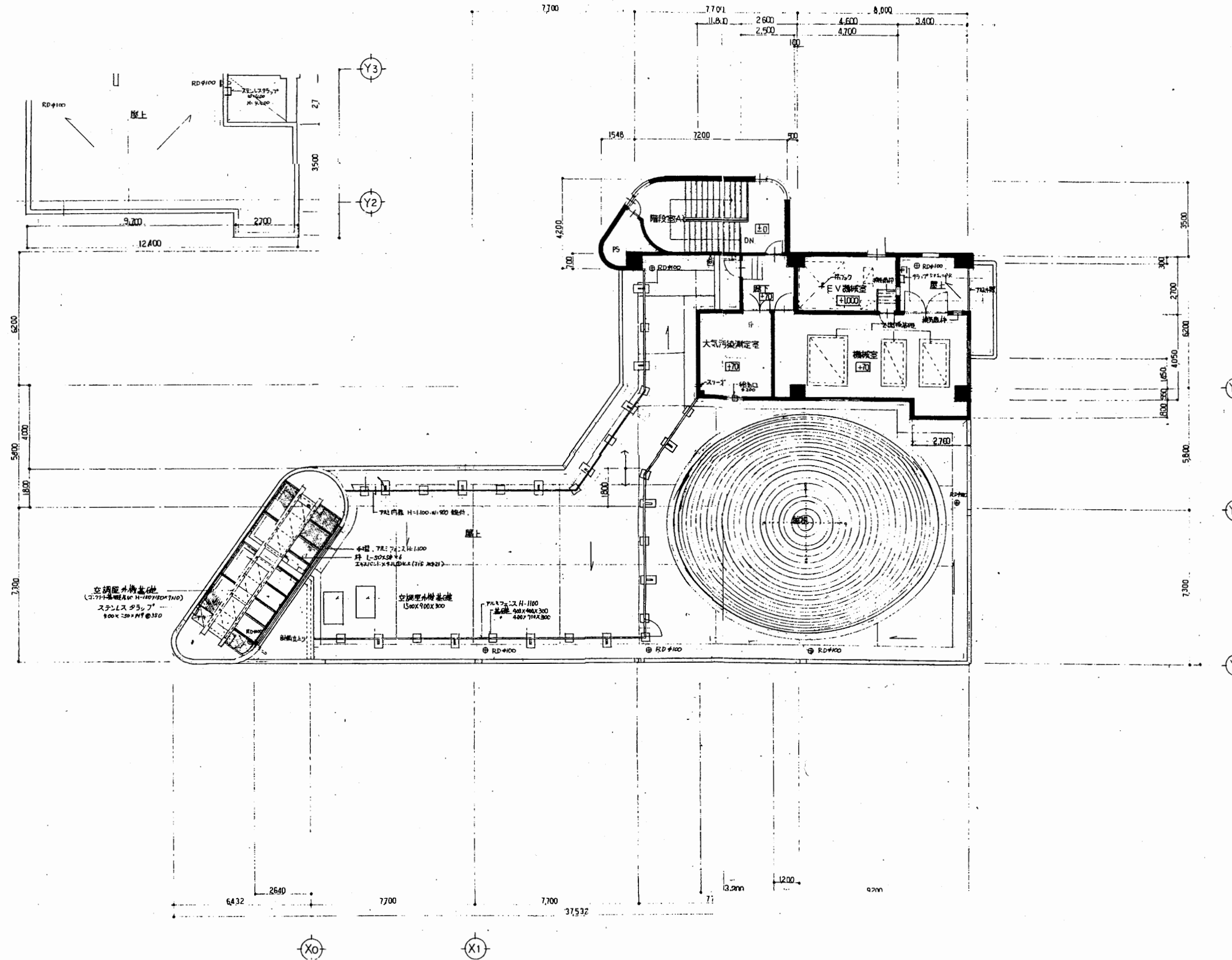
5階平面図 S 1:200
