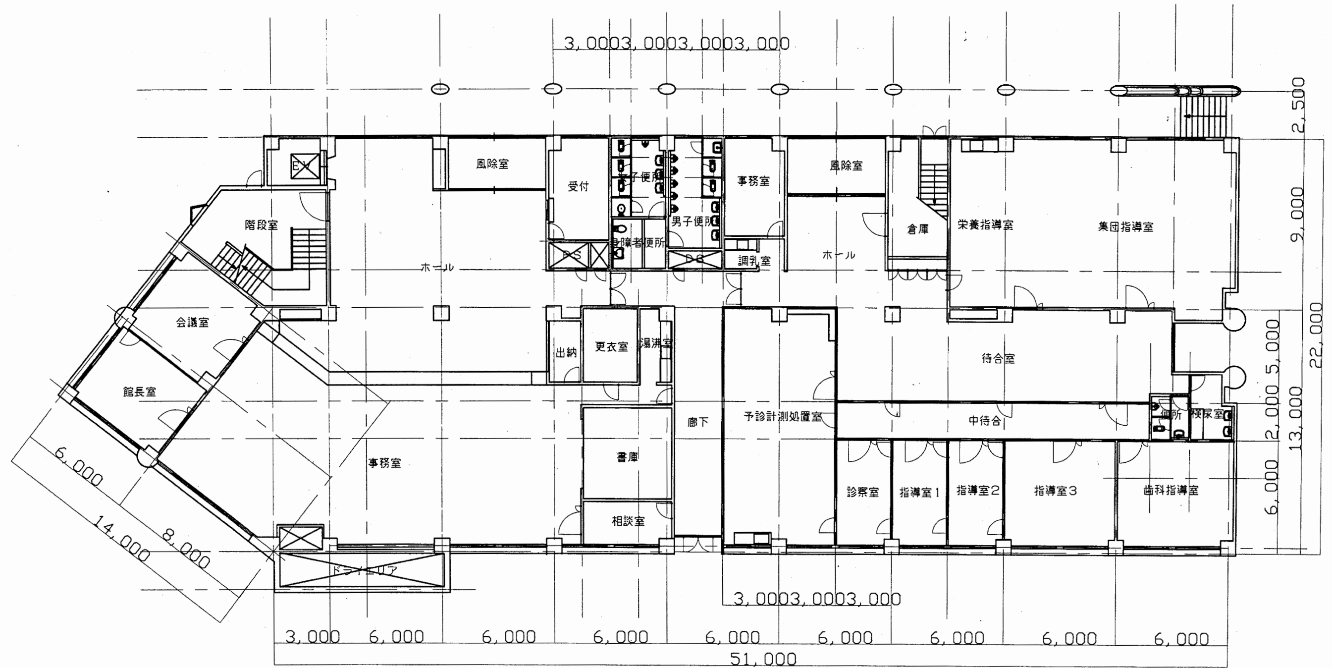
1階平面図 1:200
