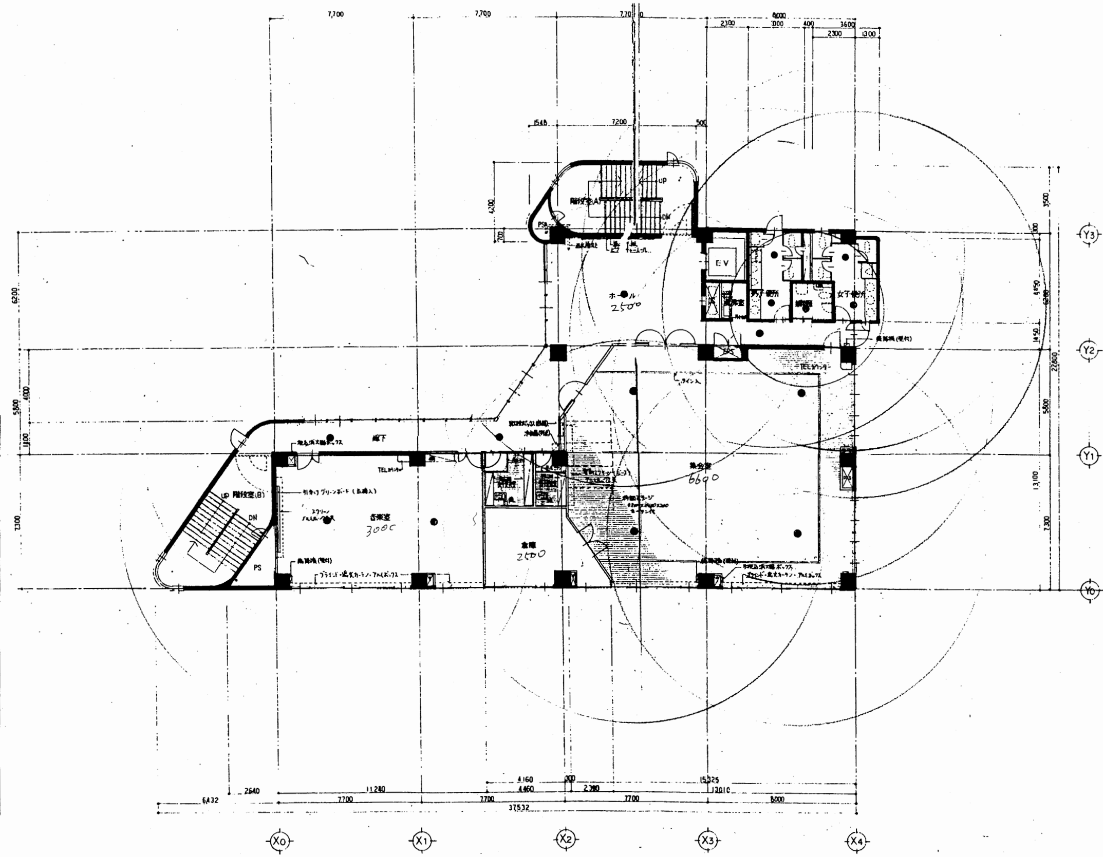
4階平面図 S 1:200
