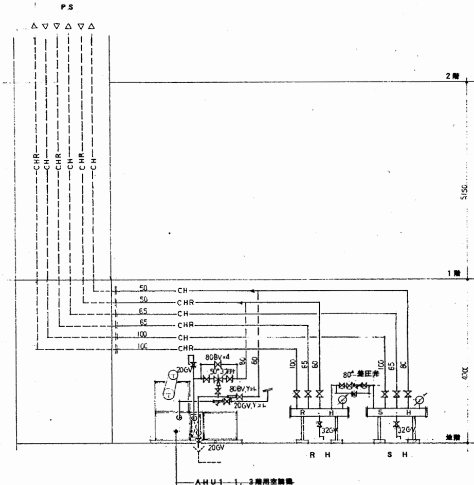
系統図 (新設)
