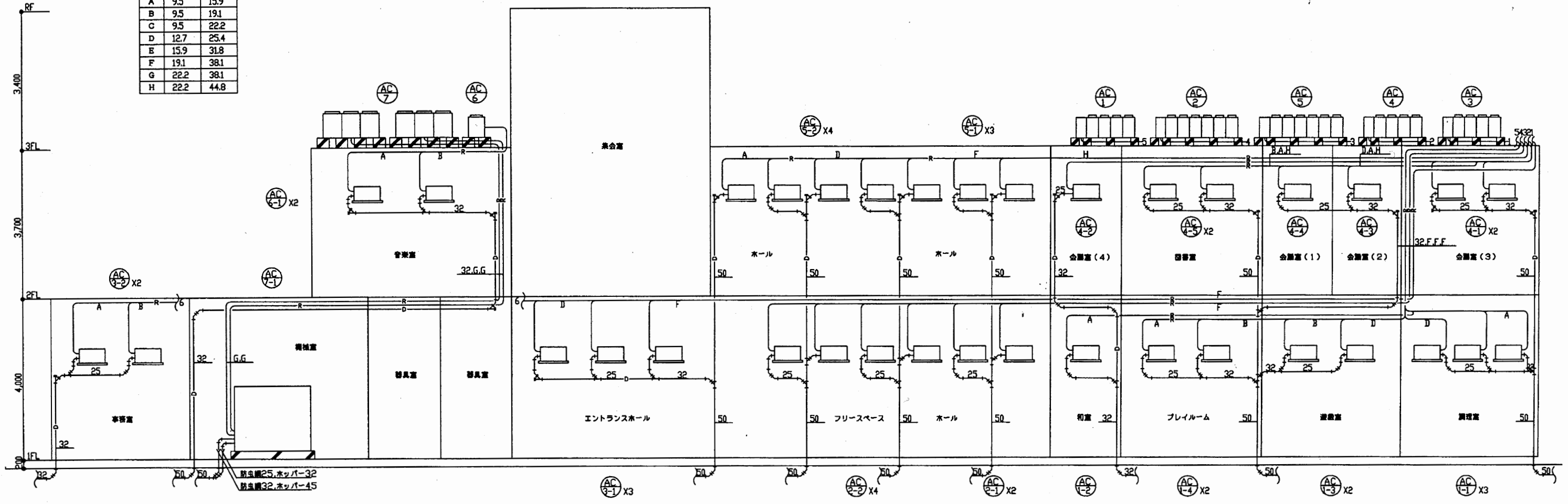
空調設備 配管系統図
