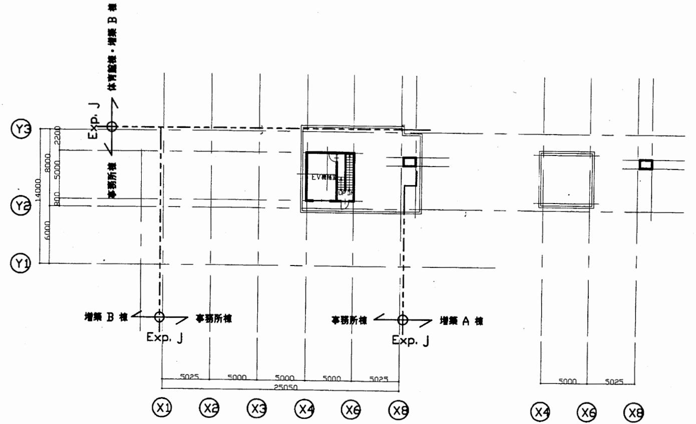
屋階平面図 S1:400
