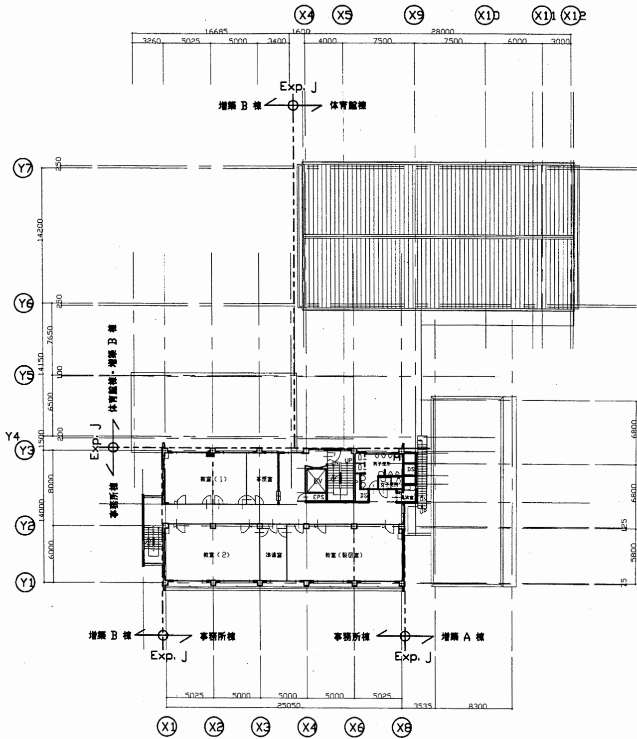
4階平面図 S1:400
