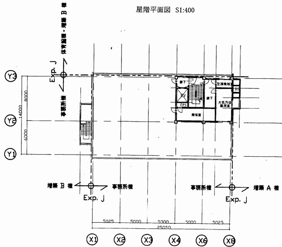
5階平面図 S1:400
