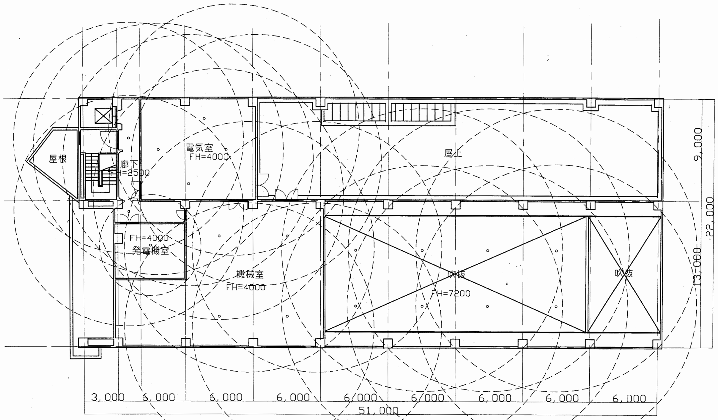
4階平面図 1:200
