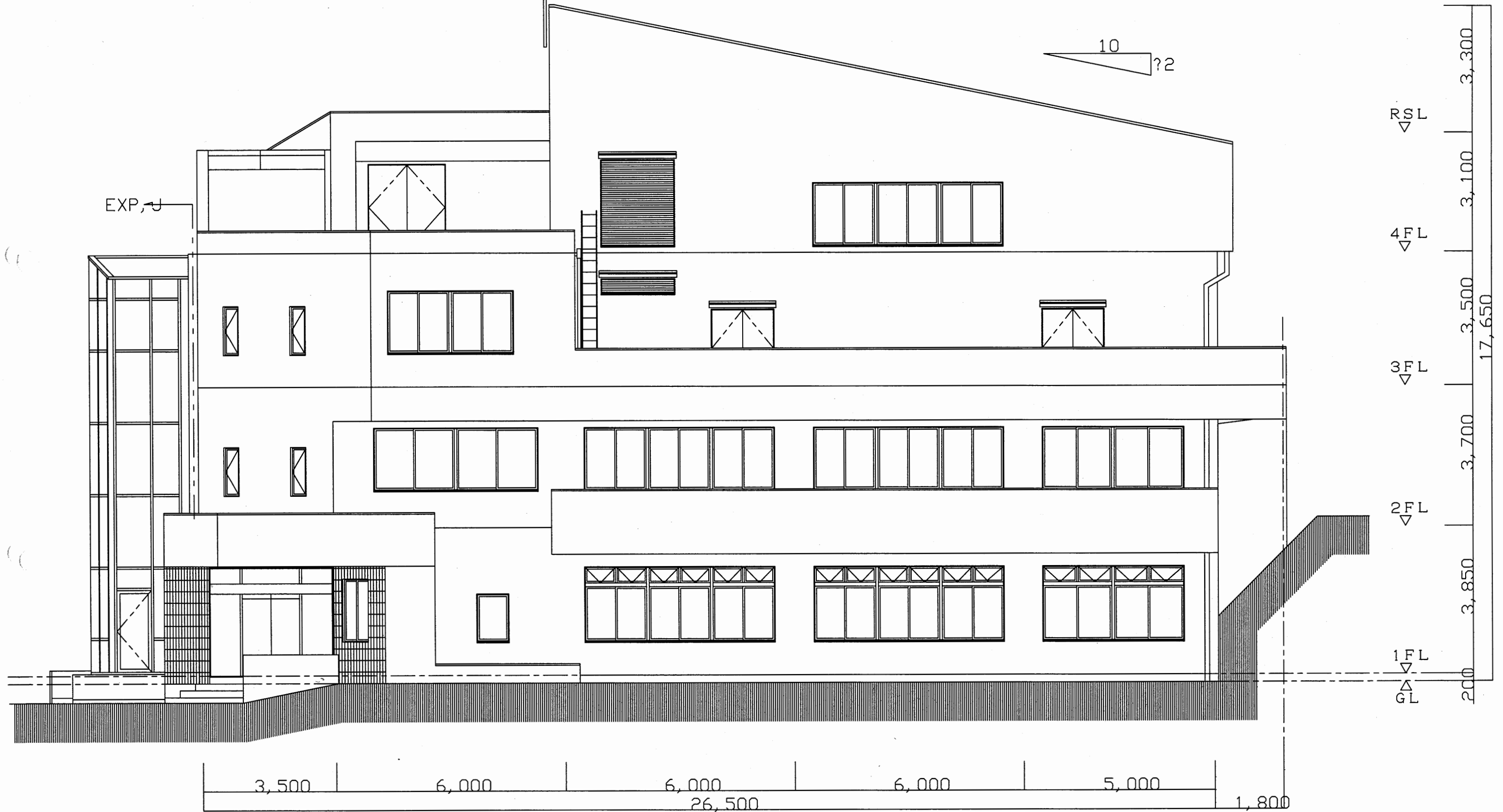
南側立面図 S=1/100
