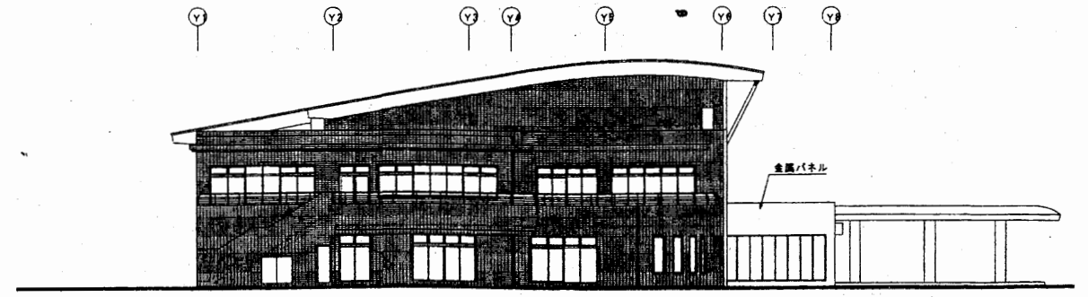
南側立面図
