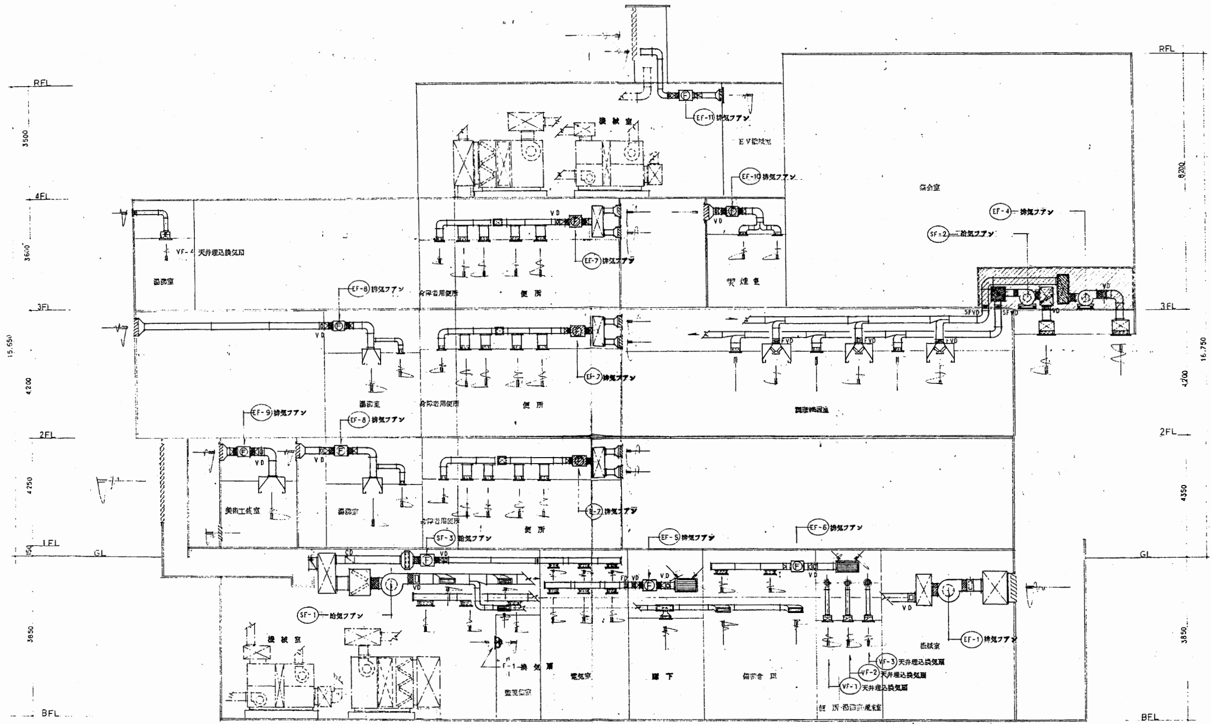
換気ダクト系統図
