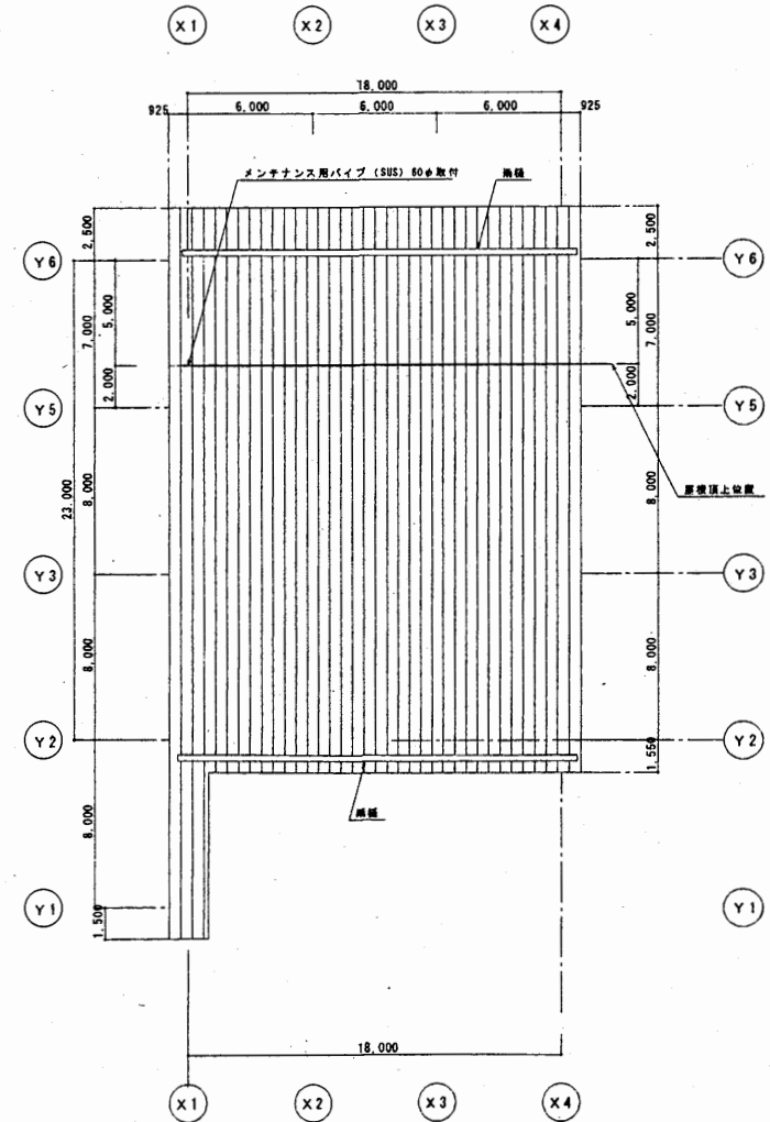
体育館屋根伏図
