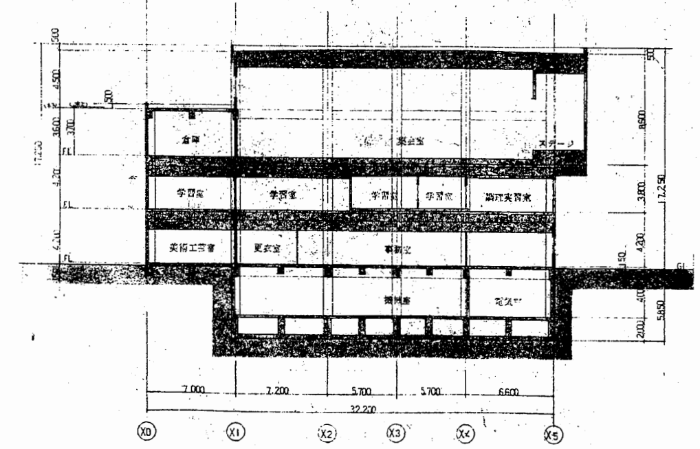
断面図 S 1:300
