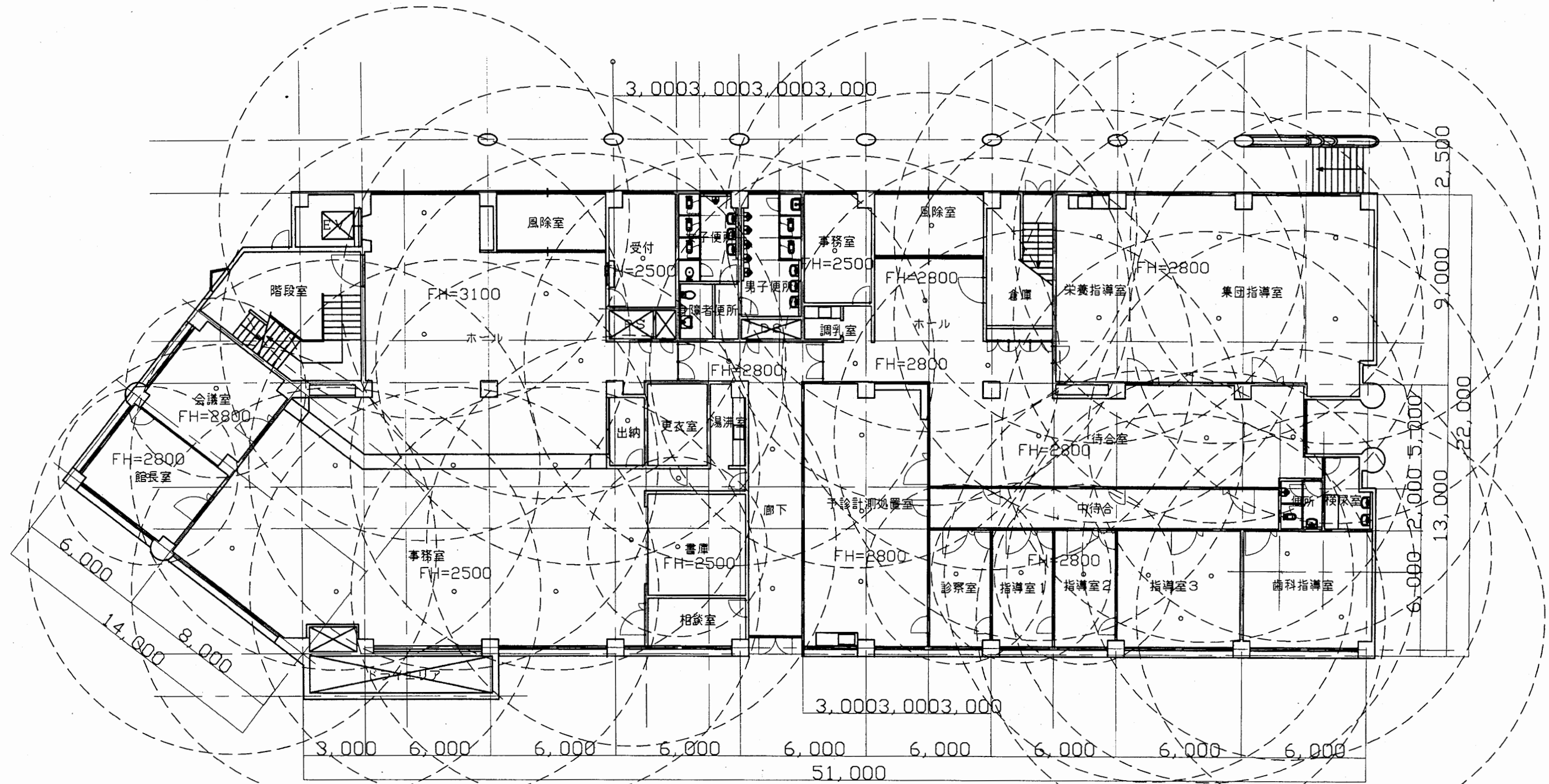
1階平面図 1:200
