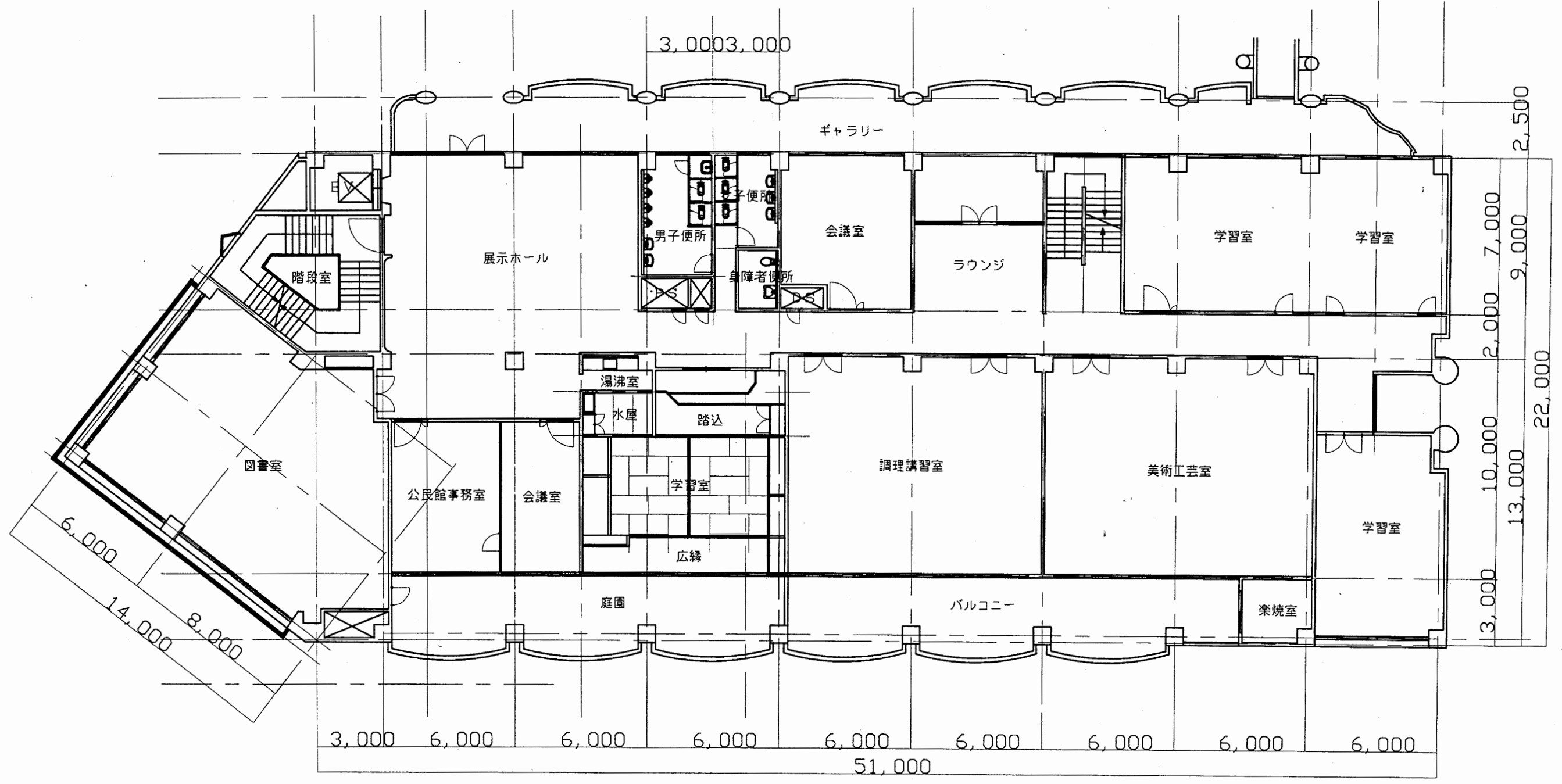
2階平面図 1:200
