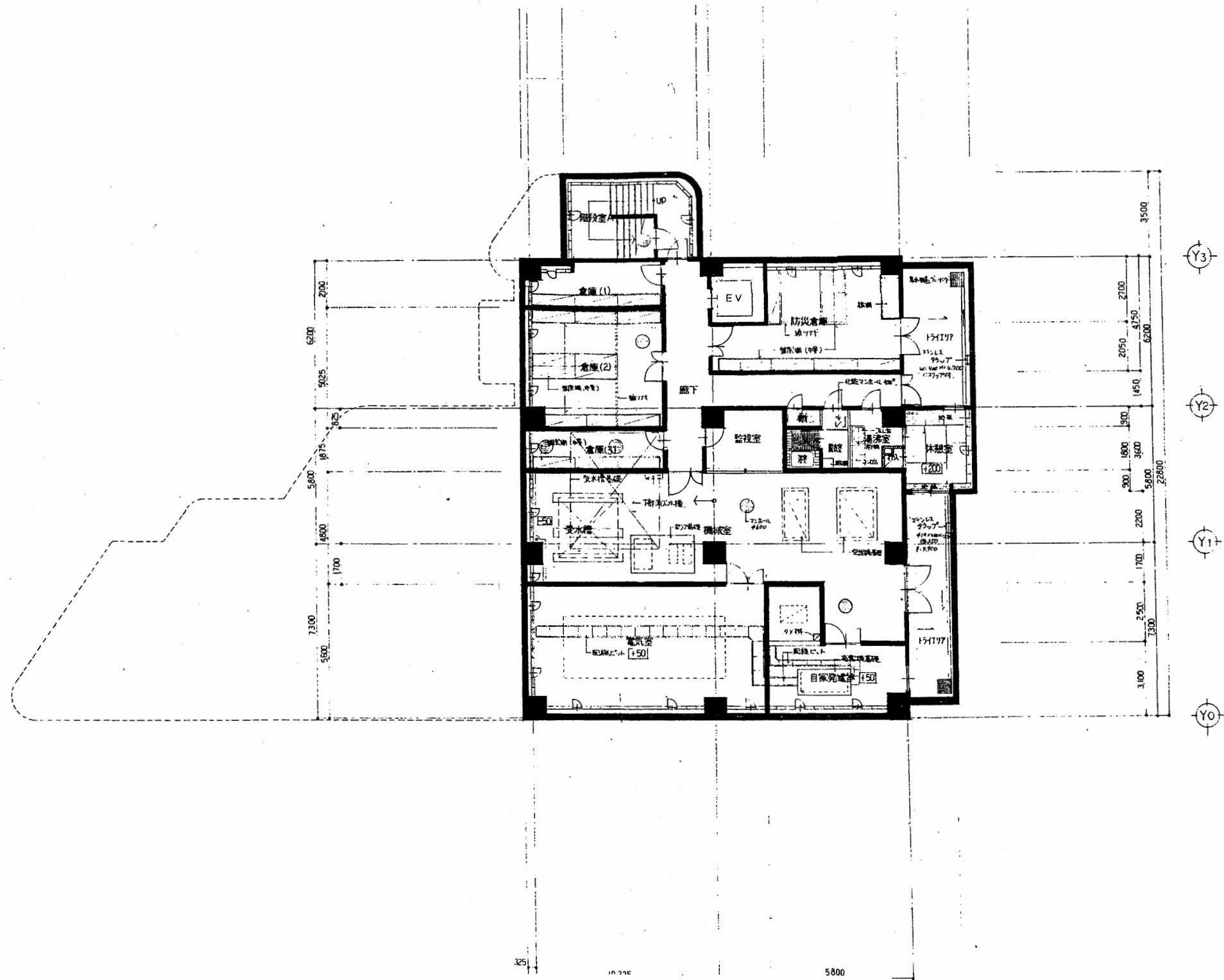
地階平面図 S 1:200
