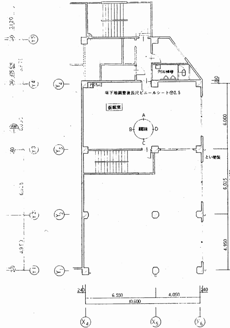
中2階平面図 S 1:200
