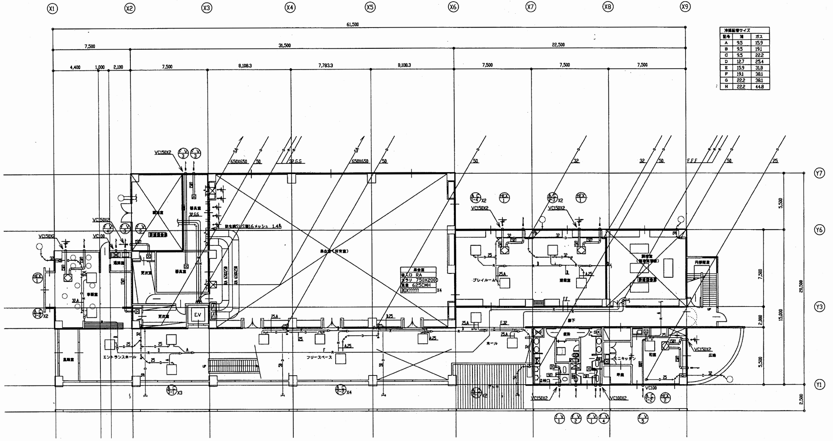
空調設備 1階平面図
