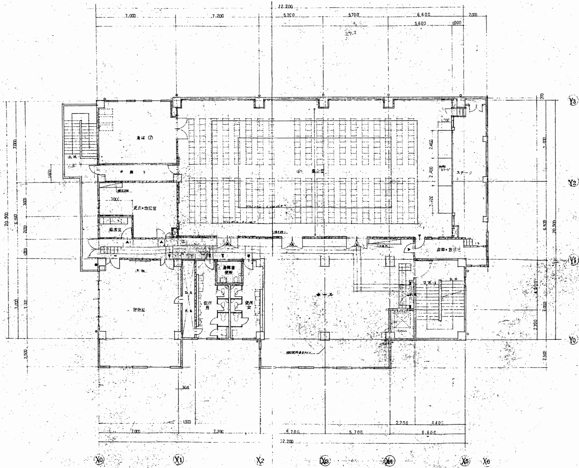
3階平面図 S 1:200
