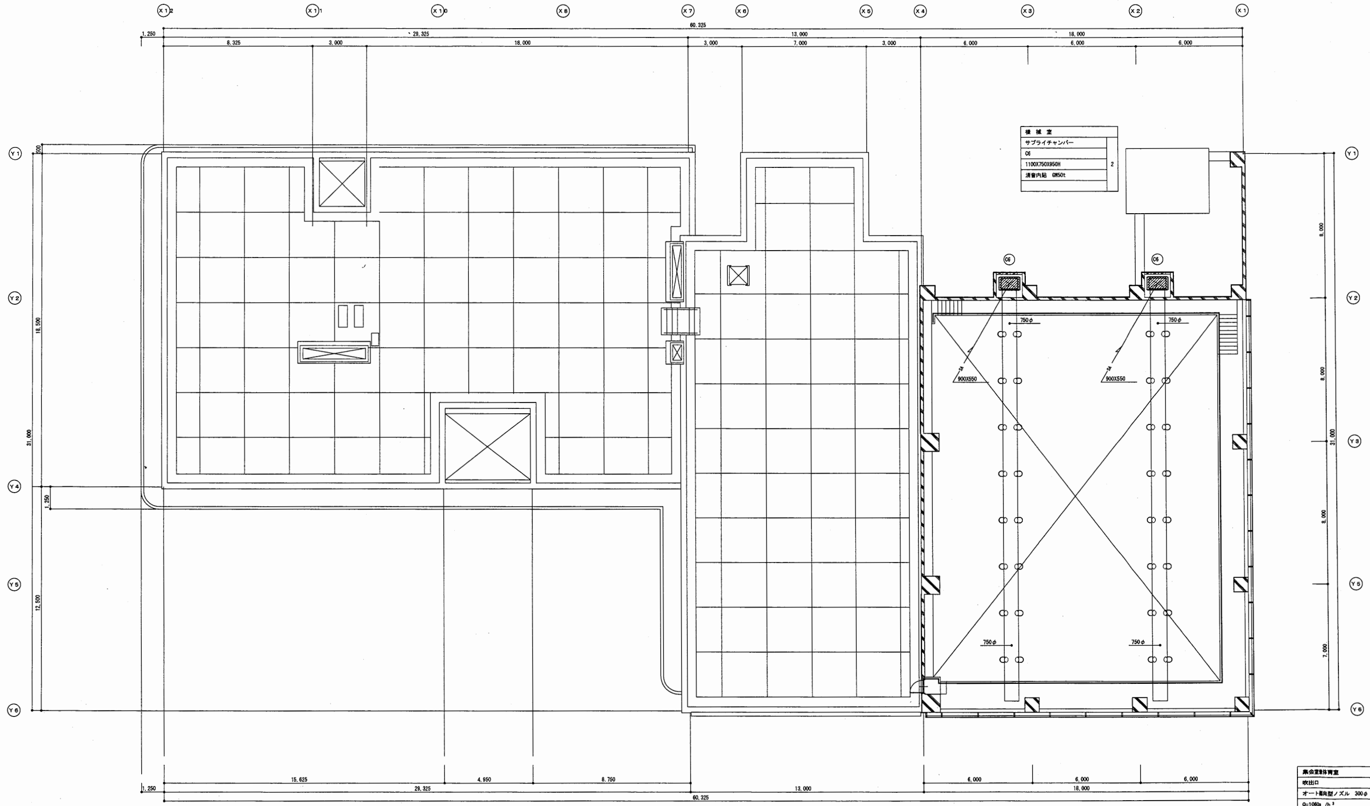
R階空調ダクト図
