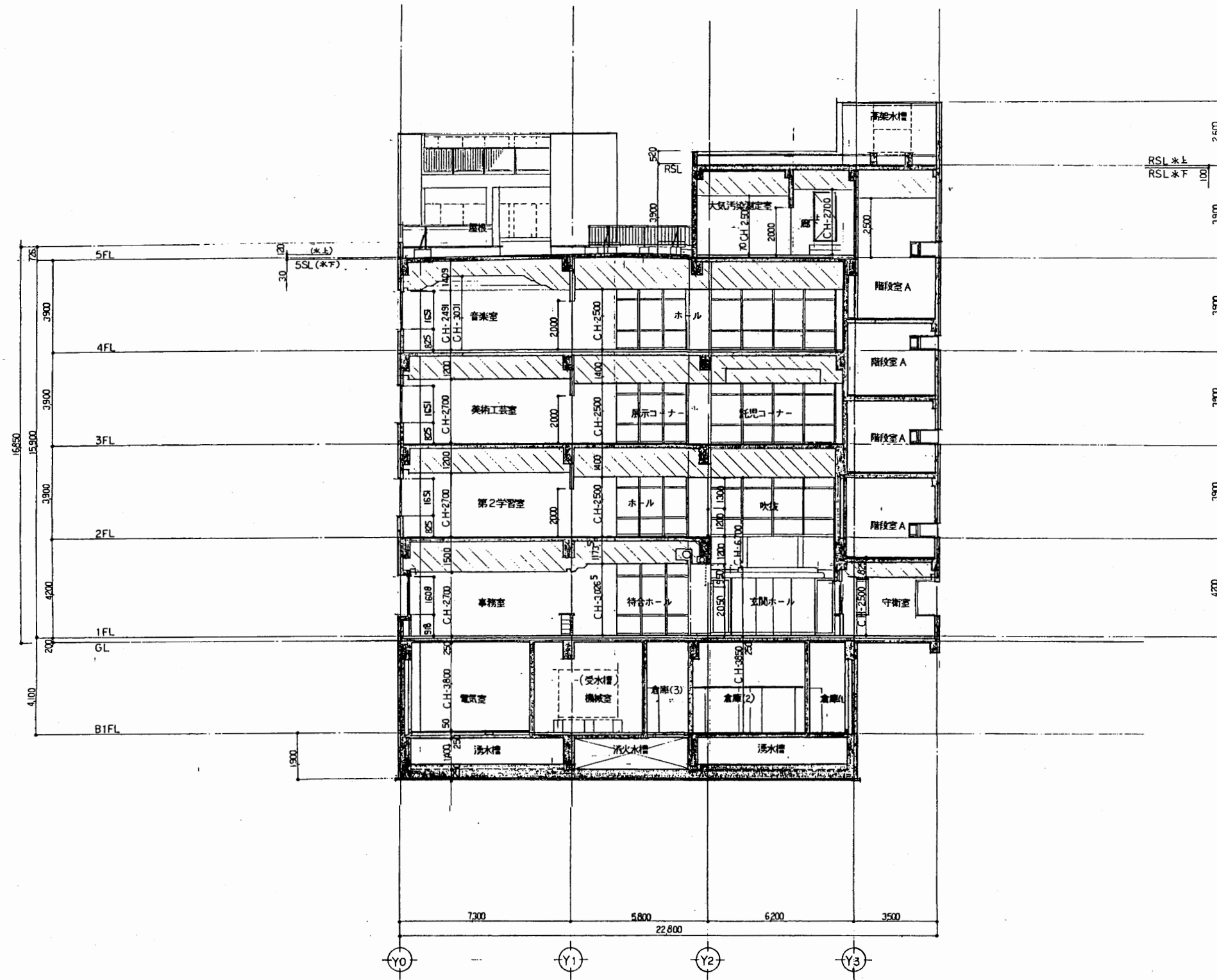
断面図 S 1:200
