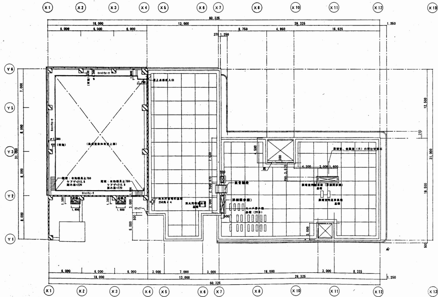
体育館屋根伏図
