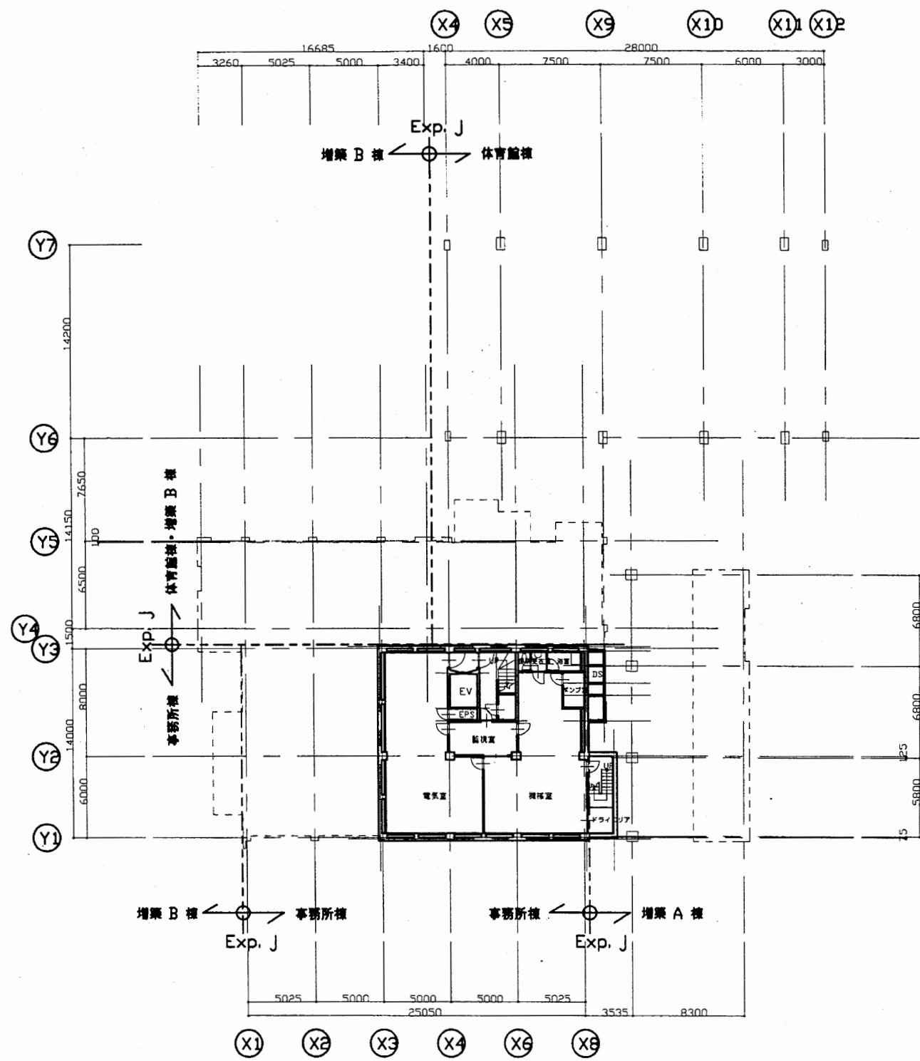
地下1階平面図 S1:400
