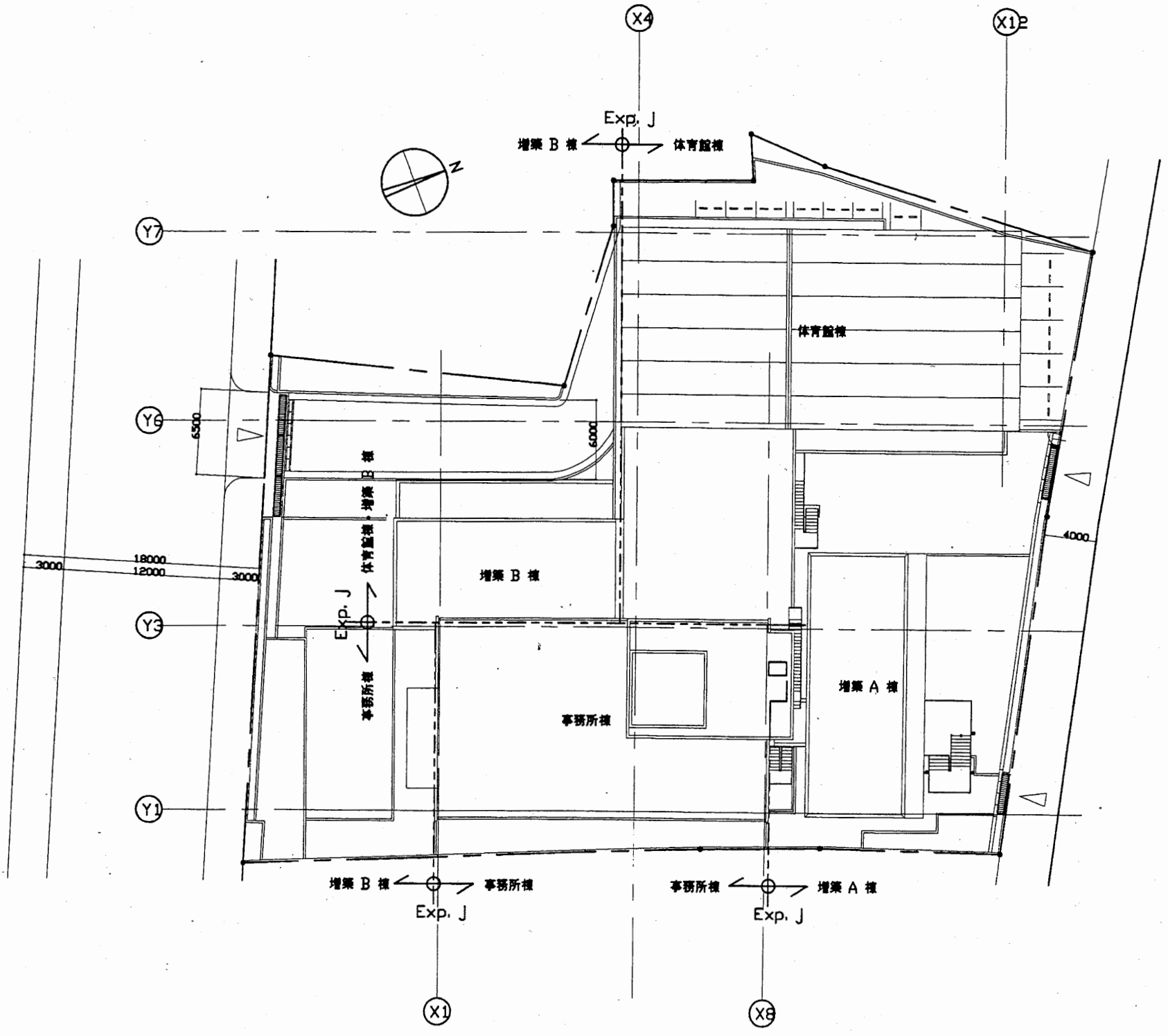
配置図 S 1:400
