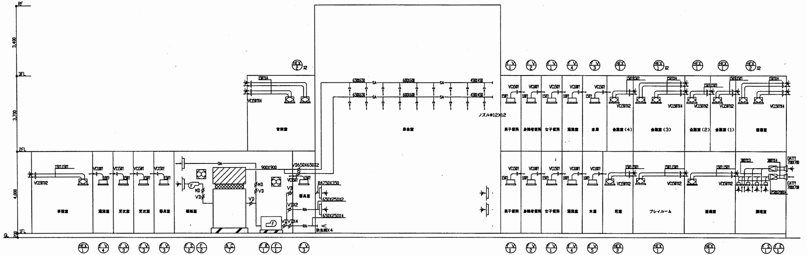
空調設備 ダクト系統図
