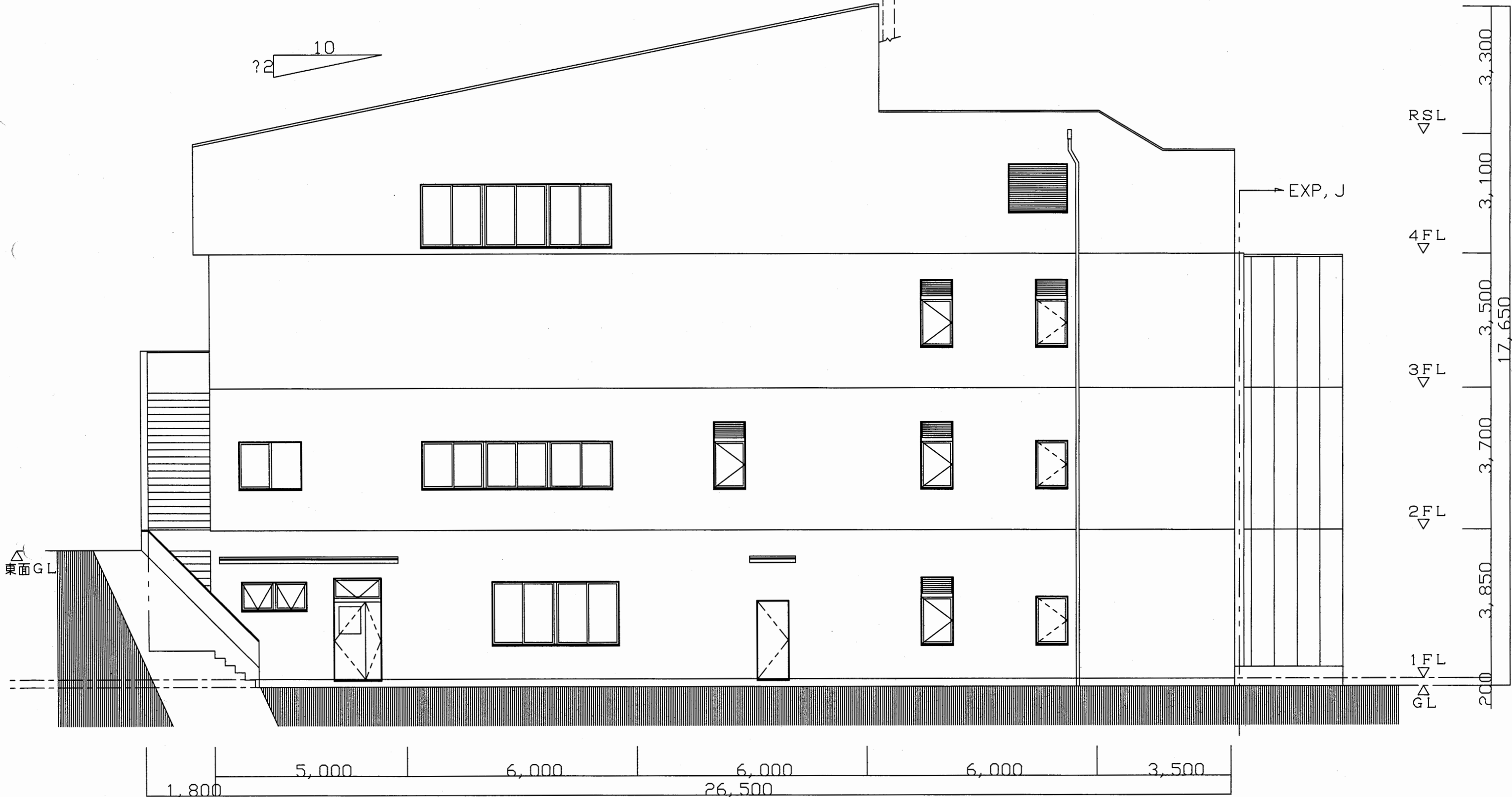
北側立面図 S=1/100
