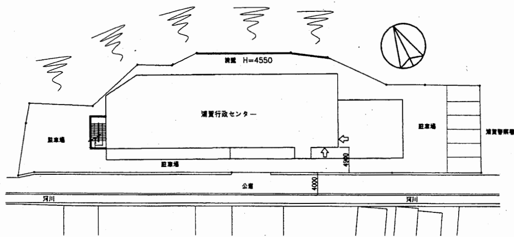
配置図 1:500
