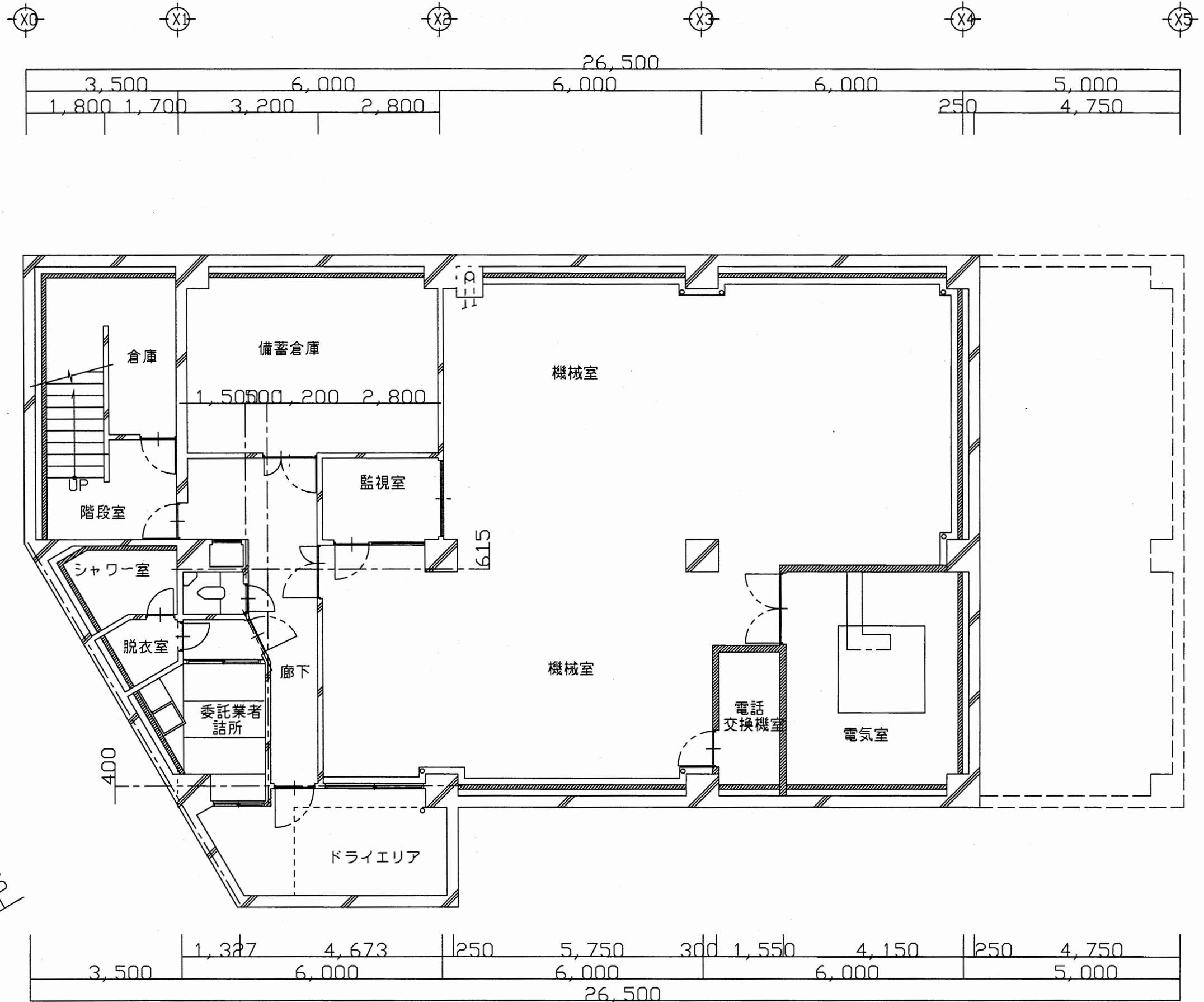
B1階平面図 S=1/100
