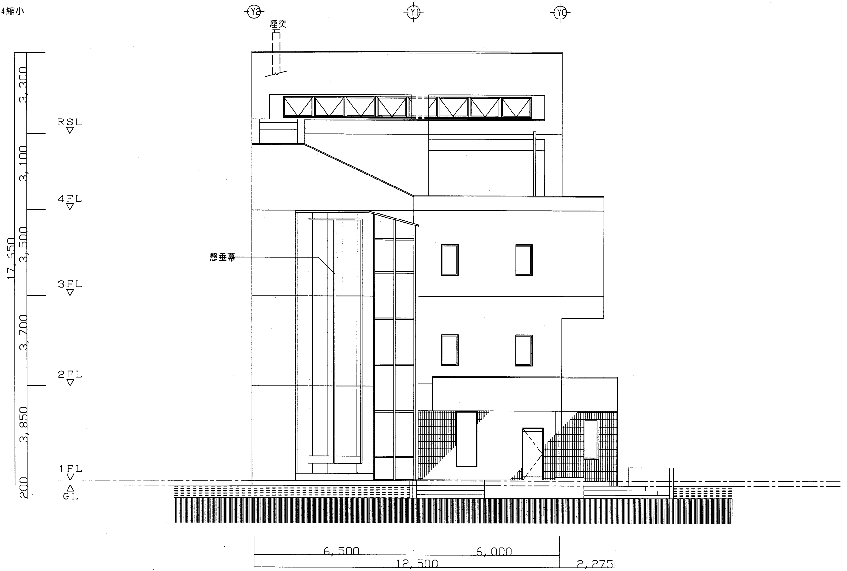
西側立面図 S=1/100
