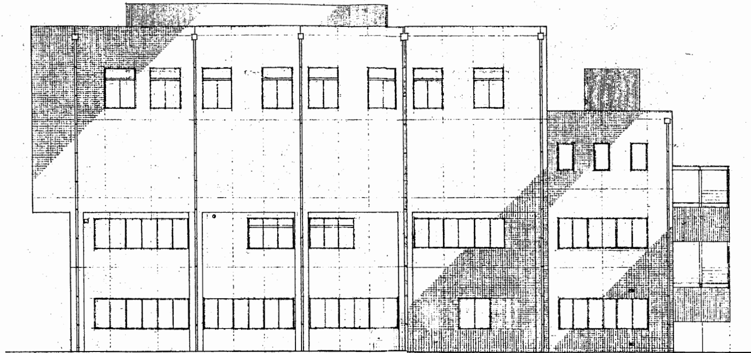
東側立面図 S 1:200
