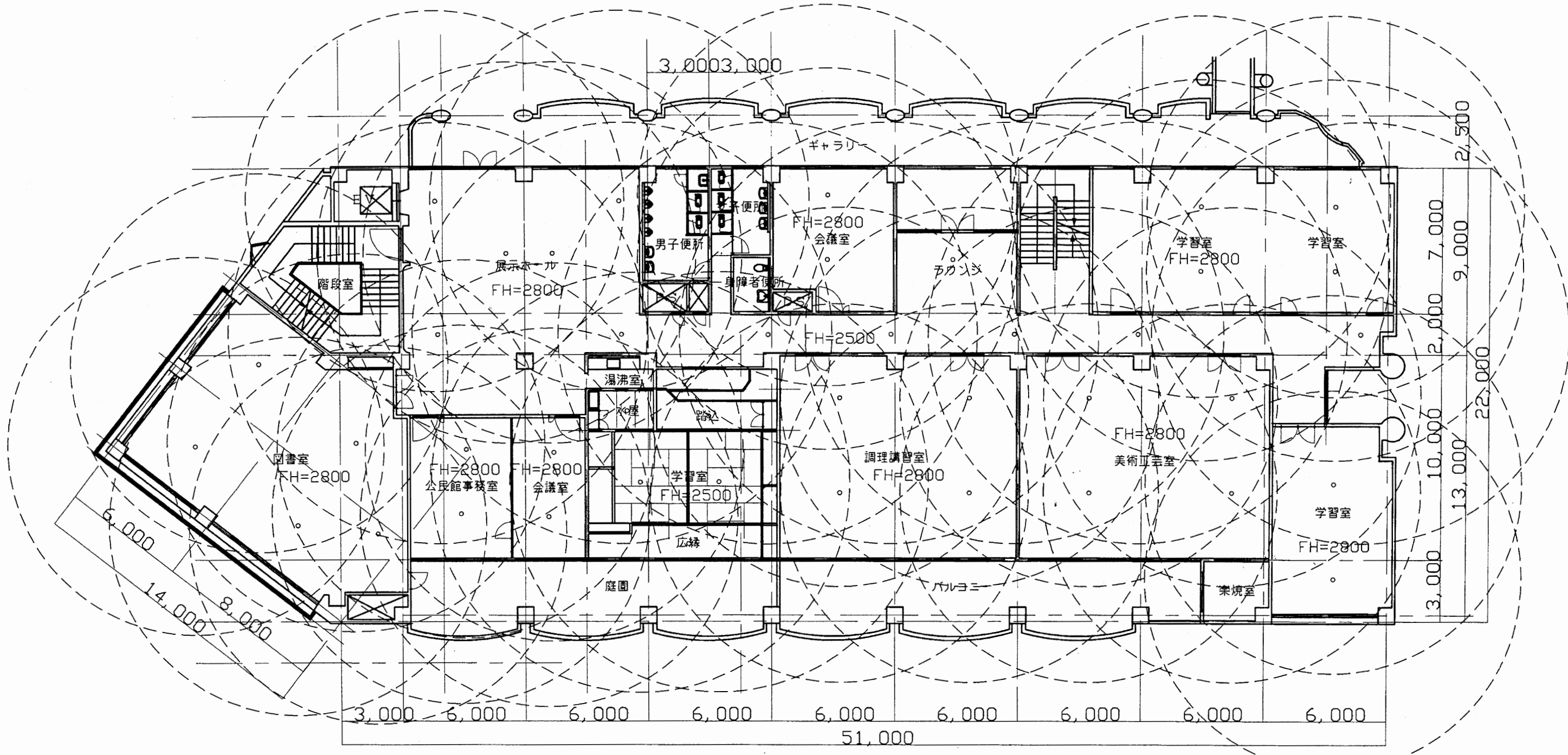
2階平面図 1: 200
