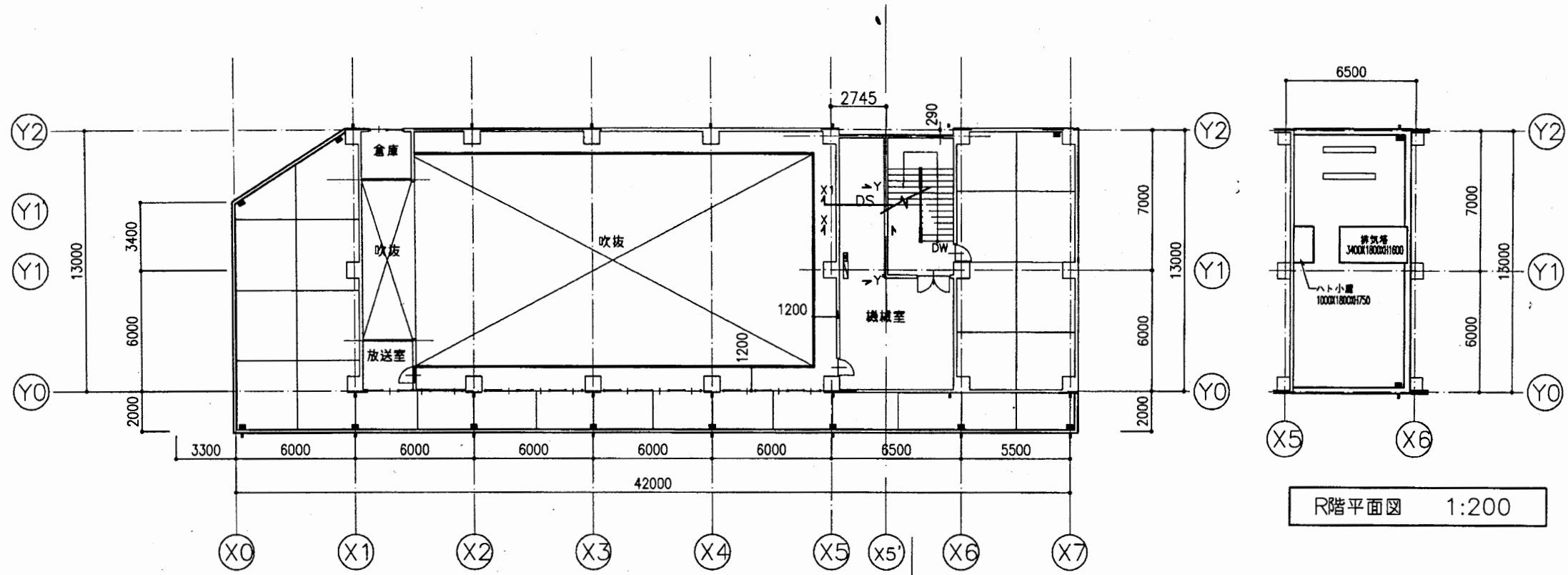
4階平面図 1:200
