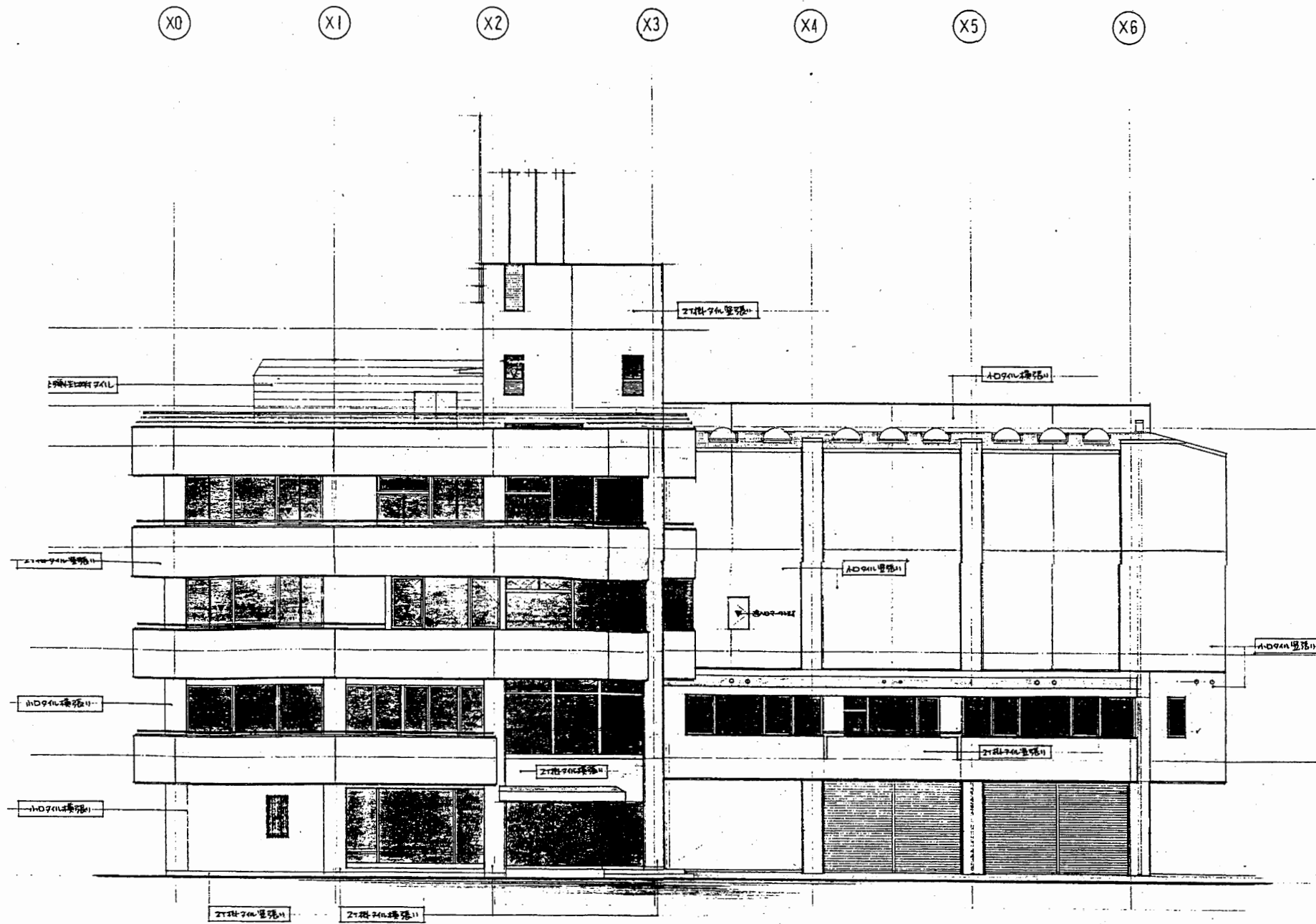
南側立面図 S 1:200
