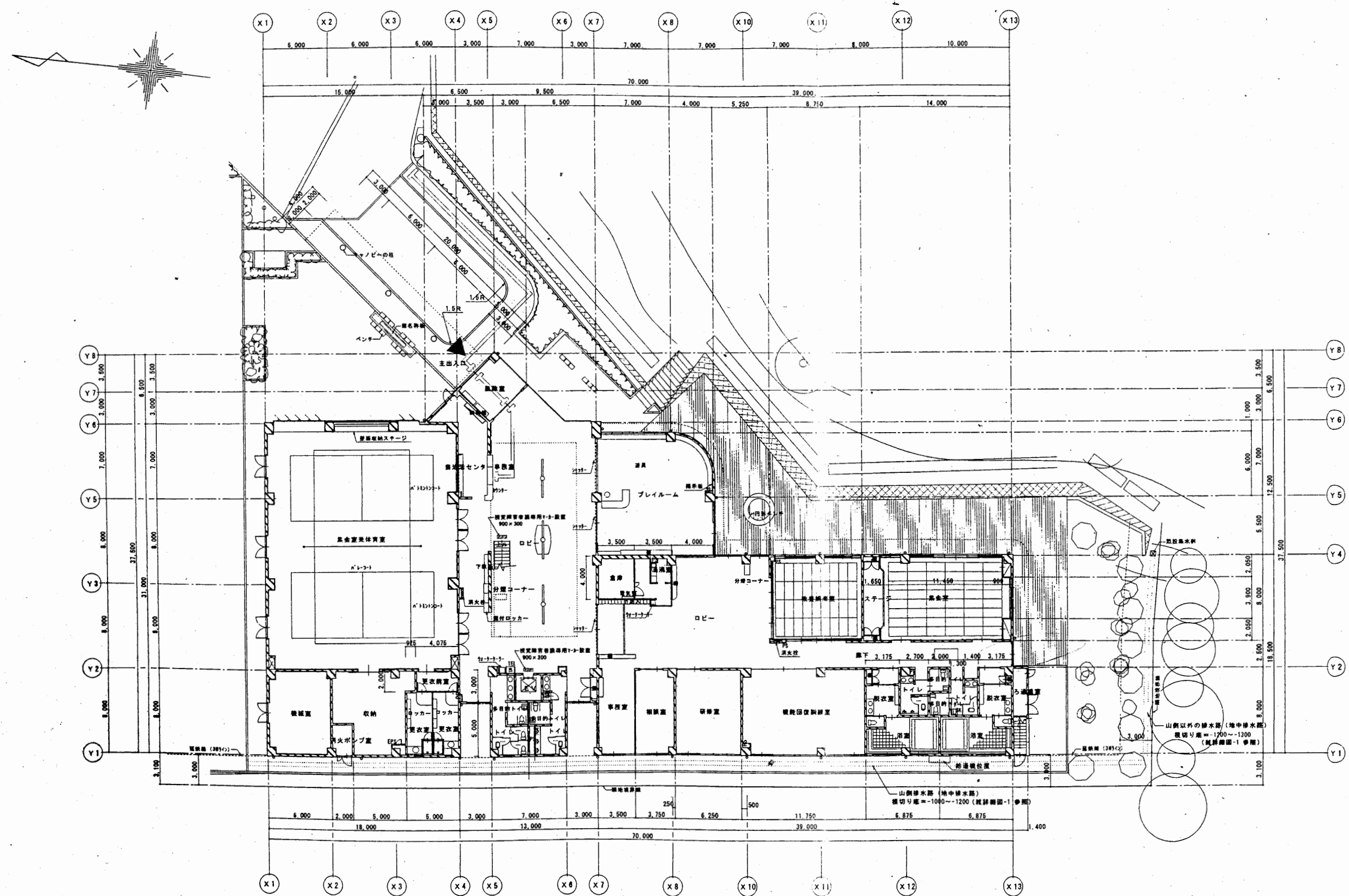
1階平面図
