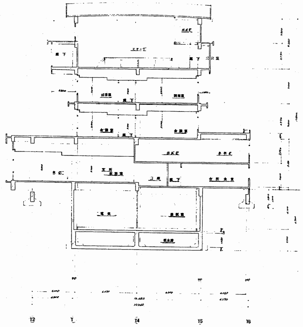
断面図 S 1:200
