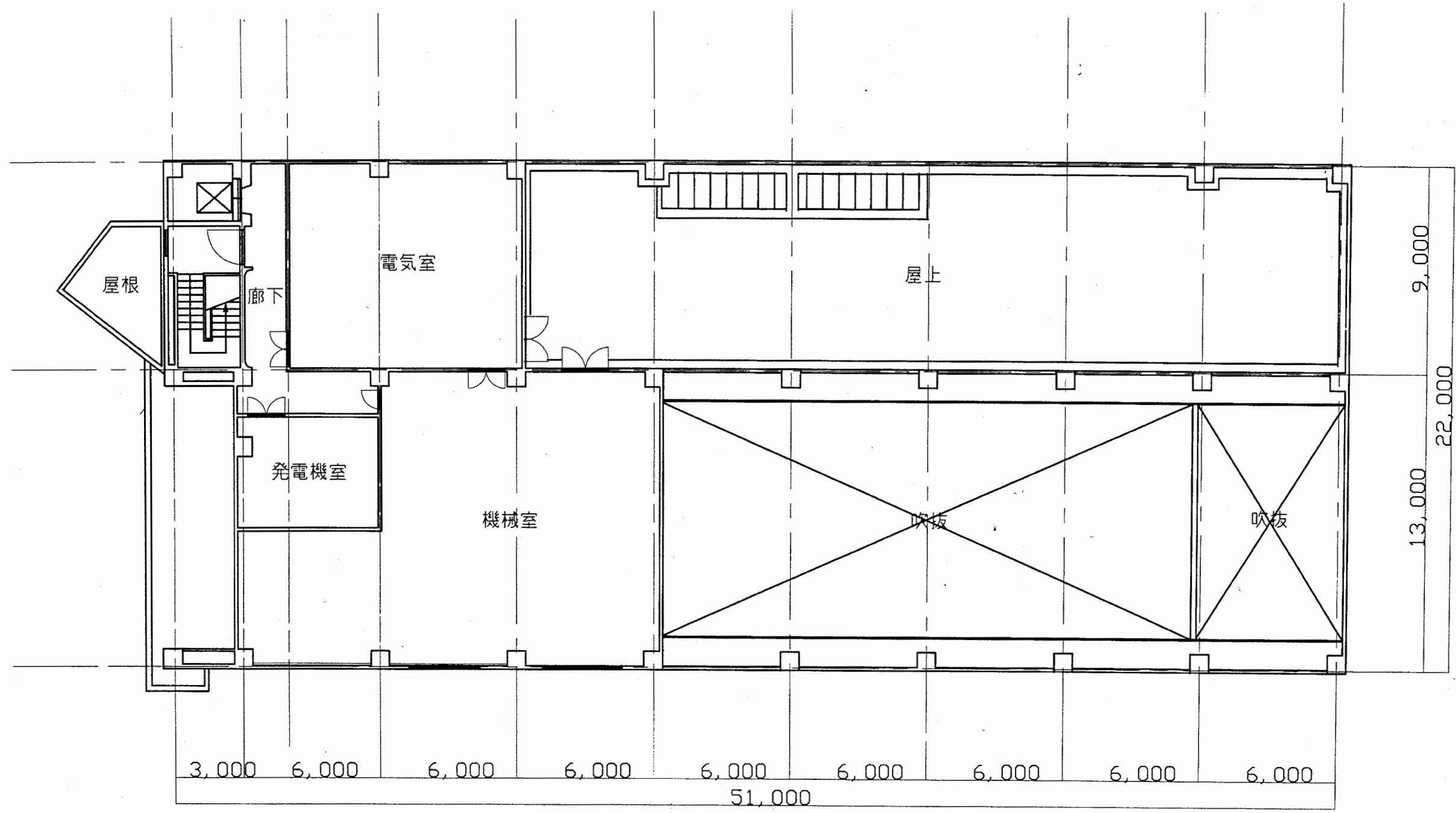
4階平面図 1:200
