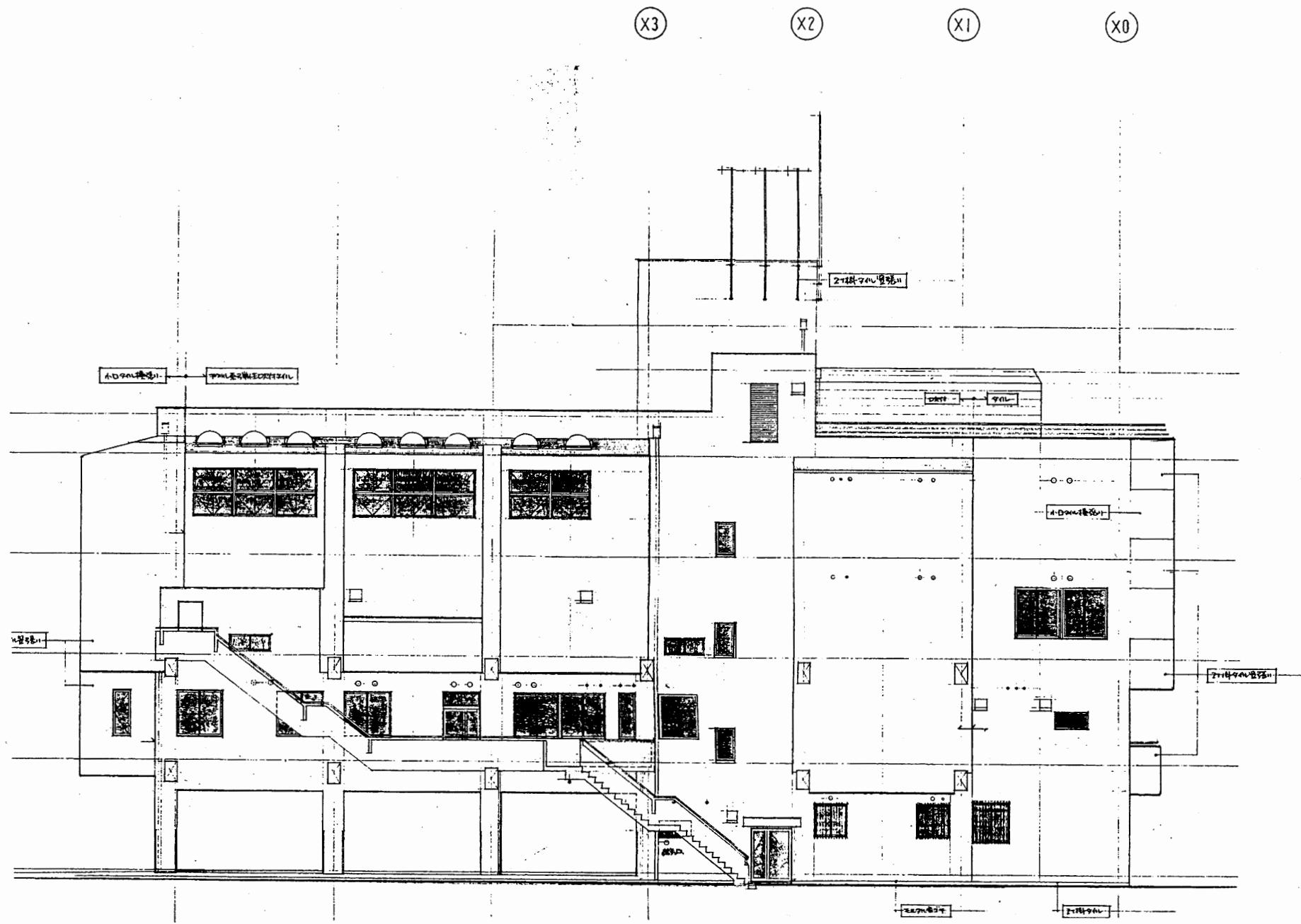
北側立面図 S 1:200
