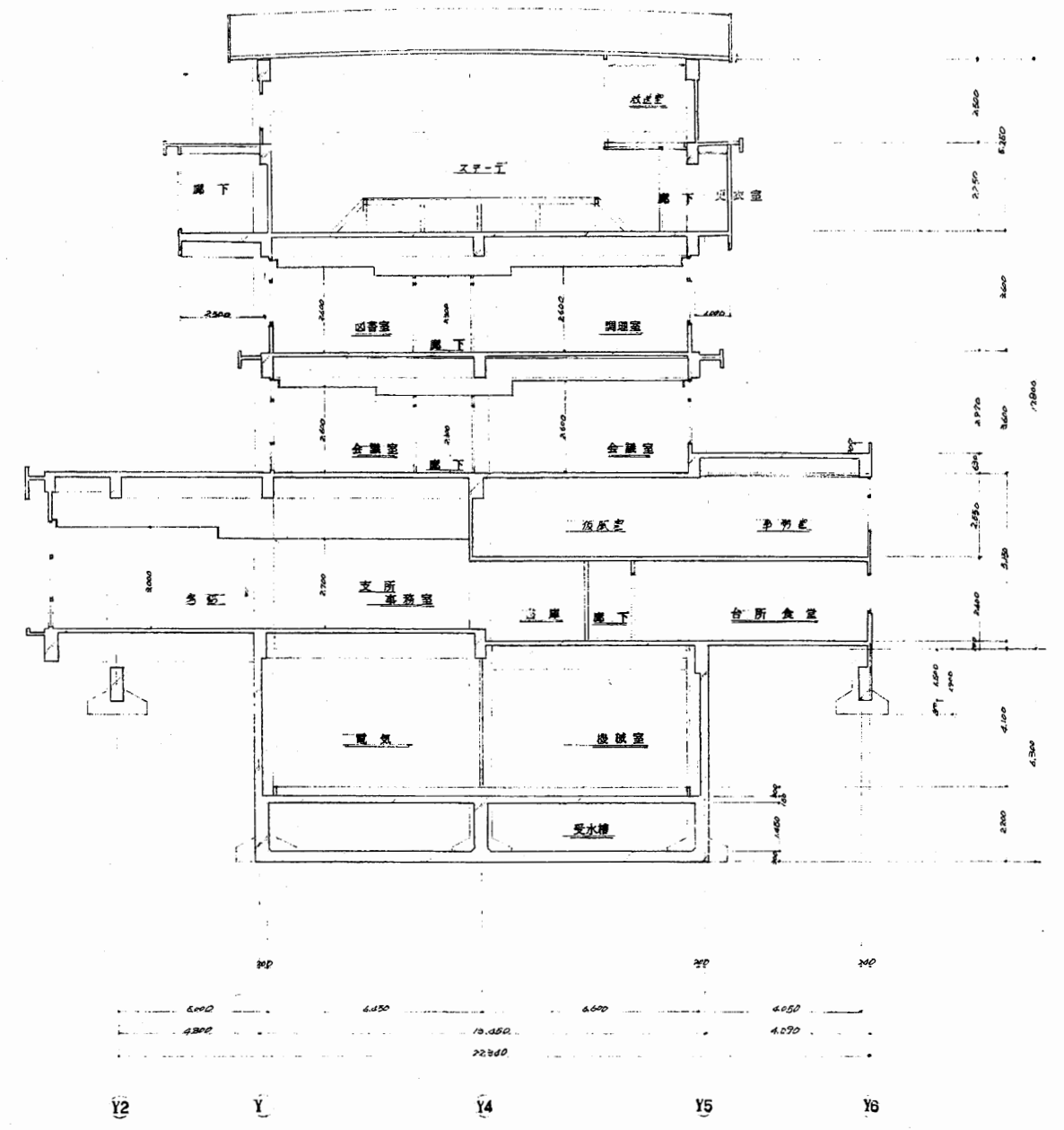
断面図 S 1:200
