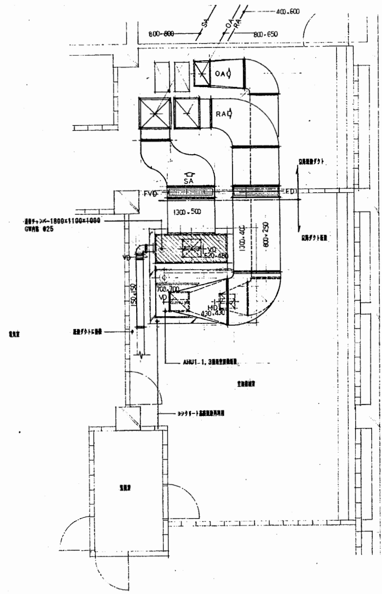
地階空調機ダクト平面図 1:50
