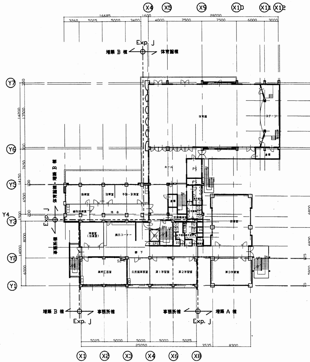
2階平面図 S1:400
