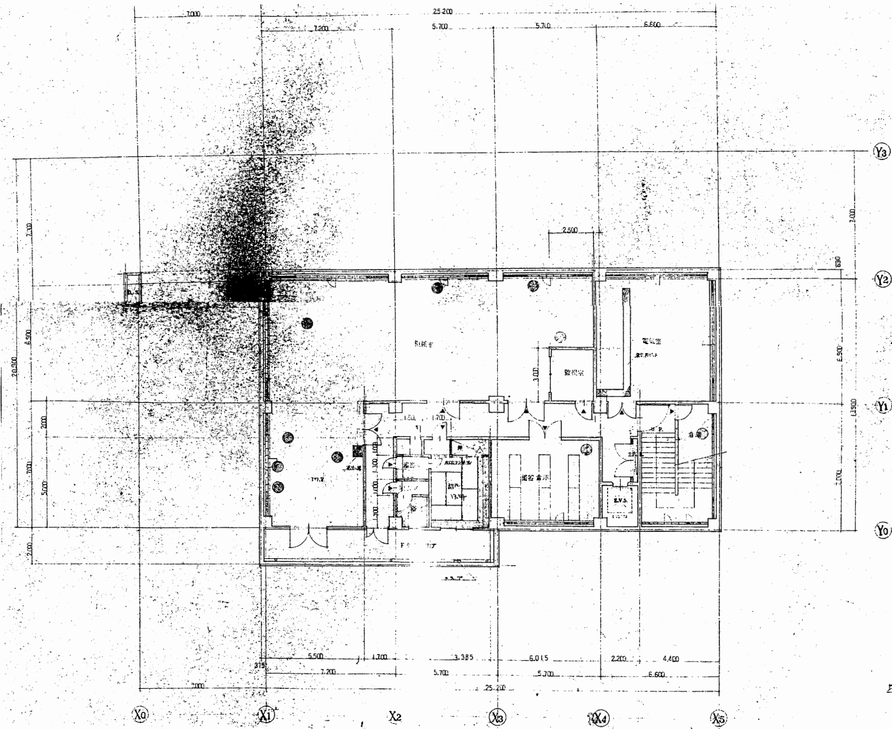
地階平面図 S 1:200
