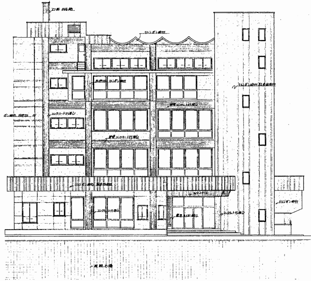
西側立面図 S 1:200
