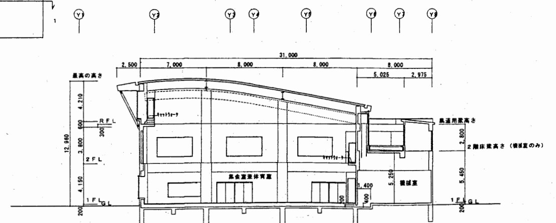
断面図
