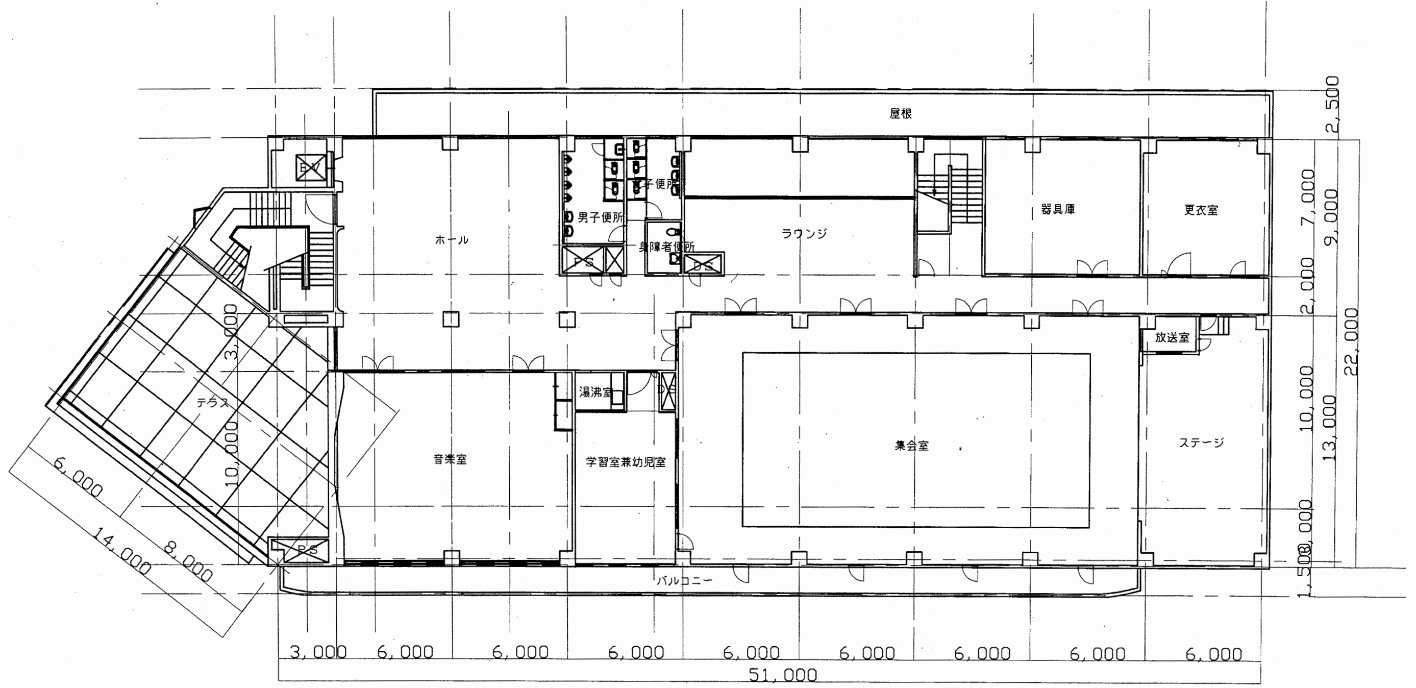
3階平面図 1:200
