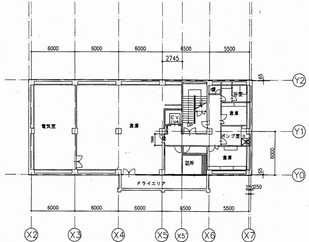
地階平面図 1:200
