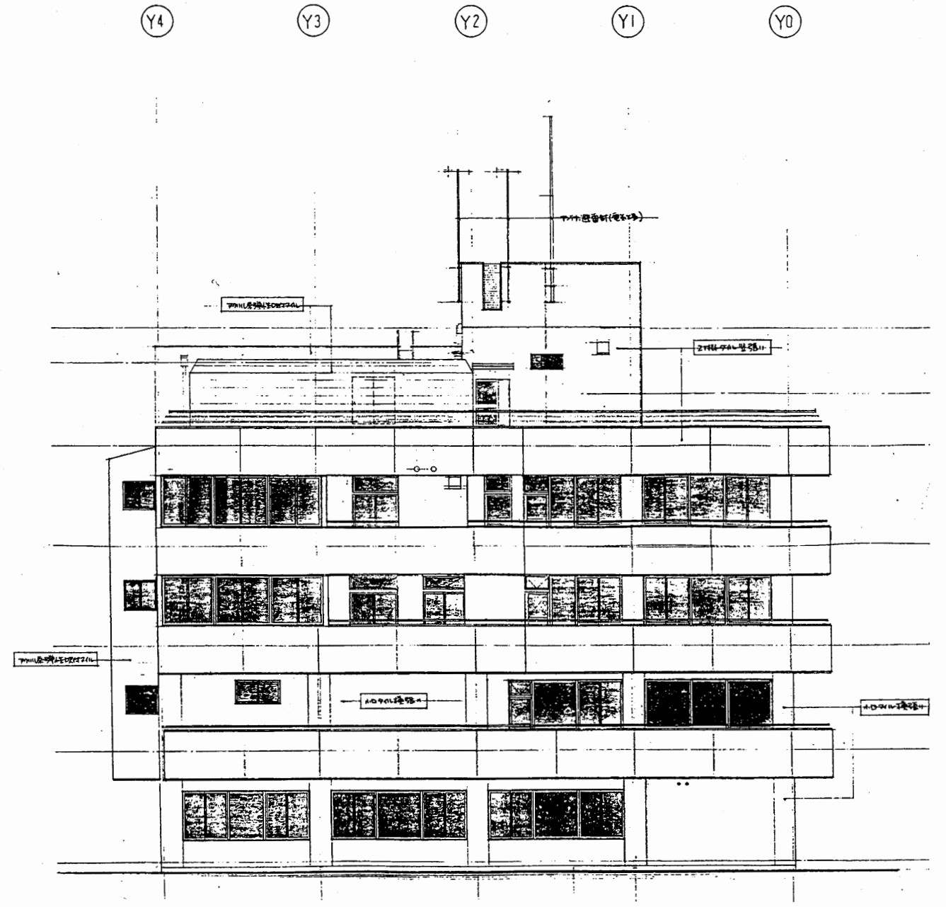
西側立面図 S 1:200
