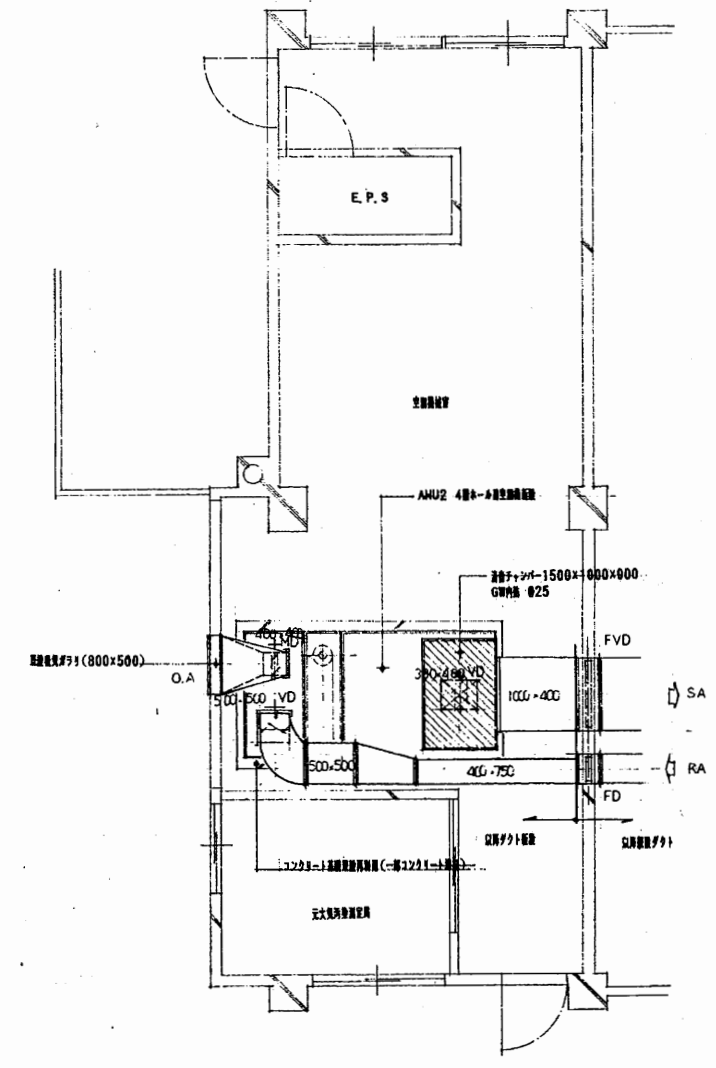
5階空調機ダクト平面図 1:50
