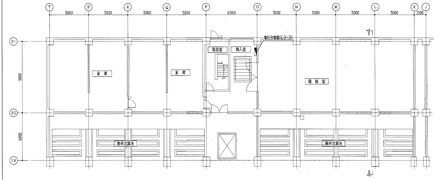
3系機械棟1階平面図 S=1/100
