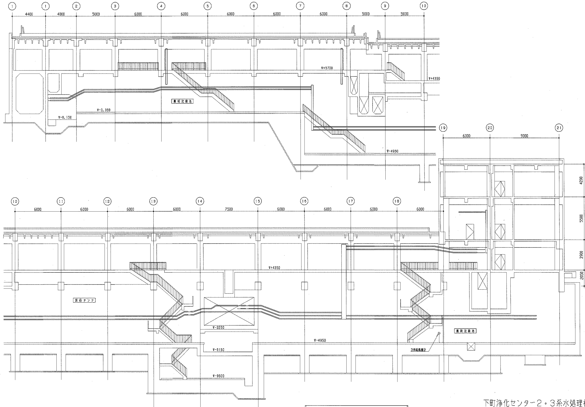
3系水処理棟B-B断面図 S=1/100
