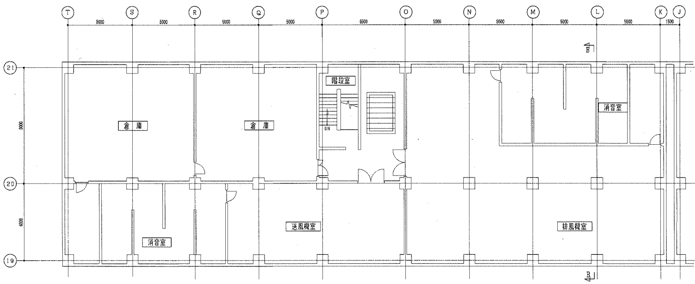
3系機械棟3階平面図 S=1/100
