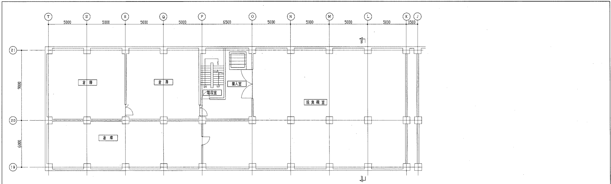
3系機械棟2階平面図 S=1/100
