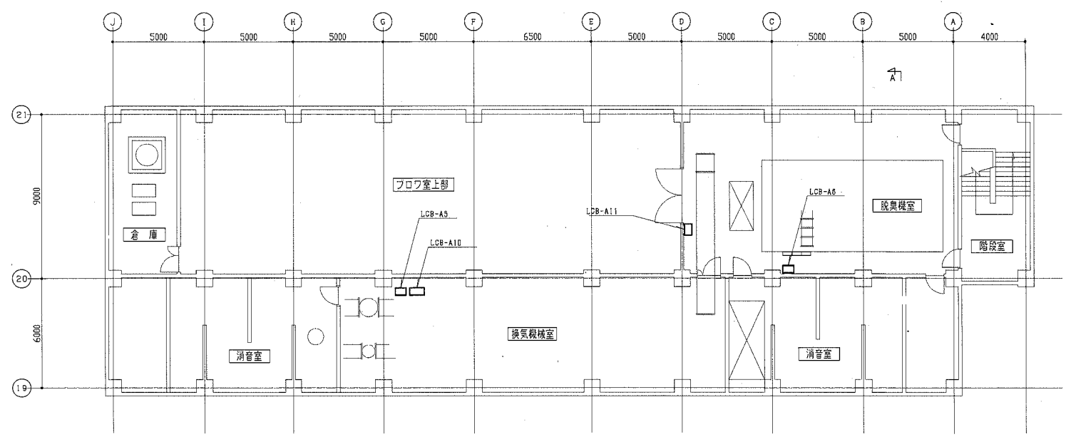
2系ブローア棟3階平面図 S=1/100
