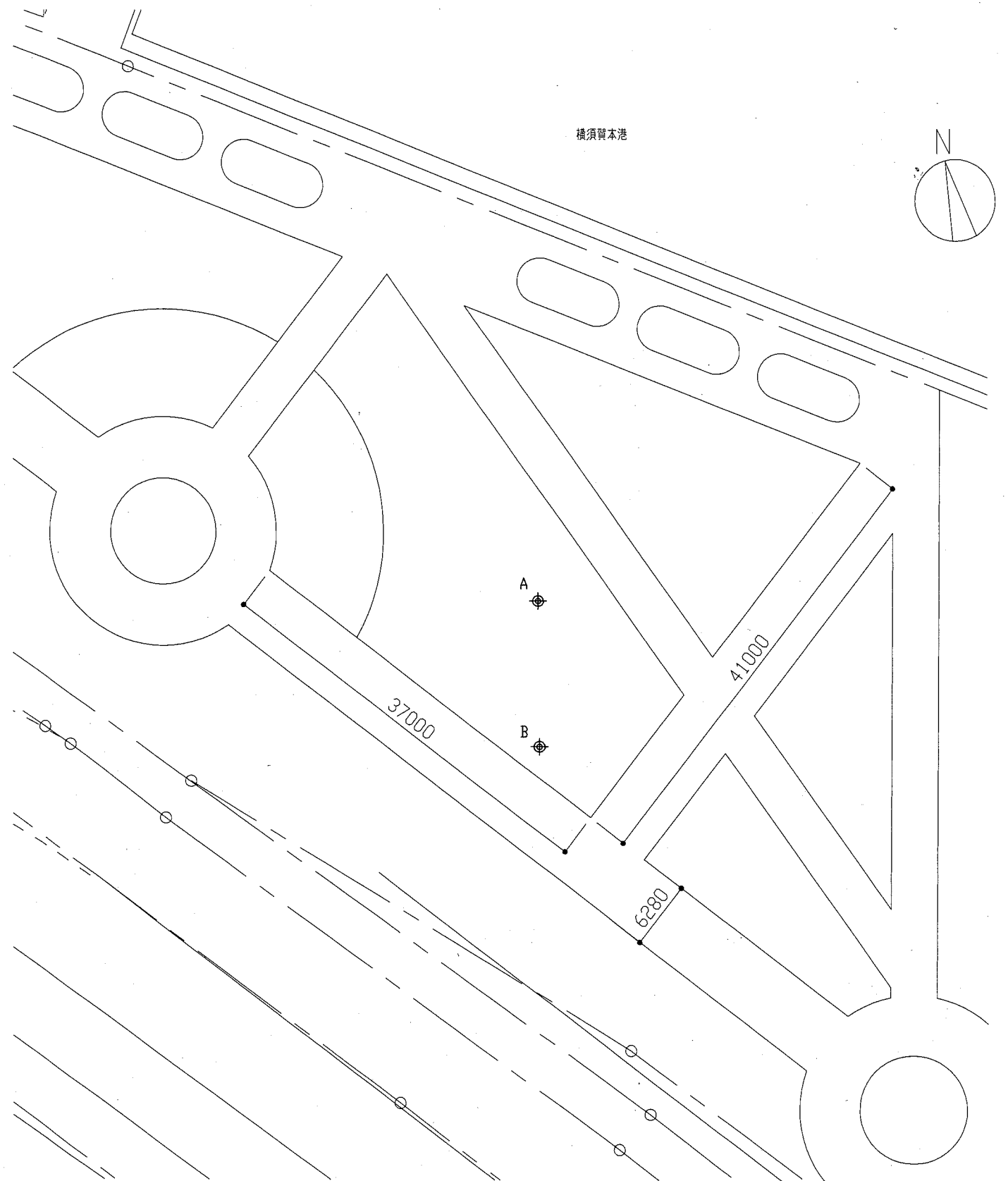
調査位置図 1:500
