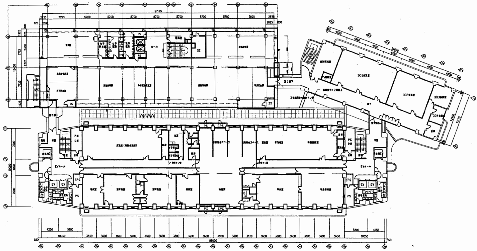
3階平面図 S 1:600
