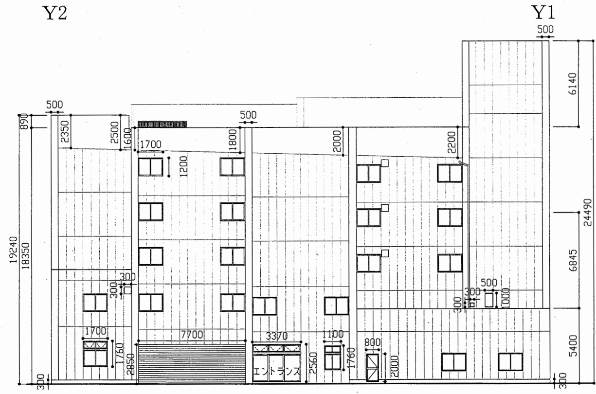
北立面図 1/200
