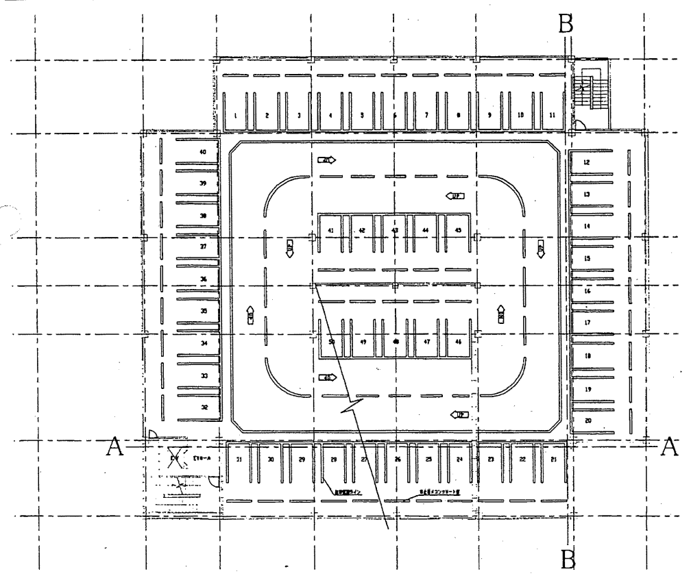
5階平面図 1/300
