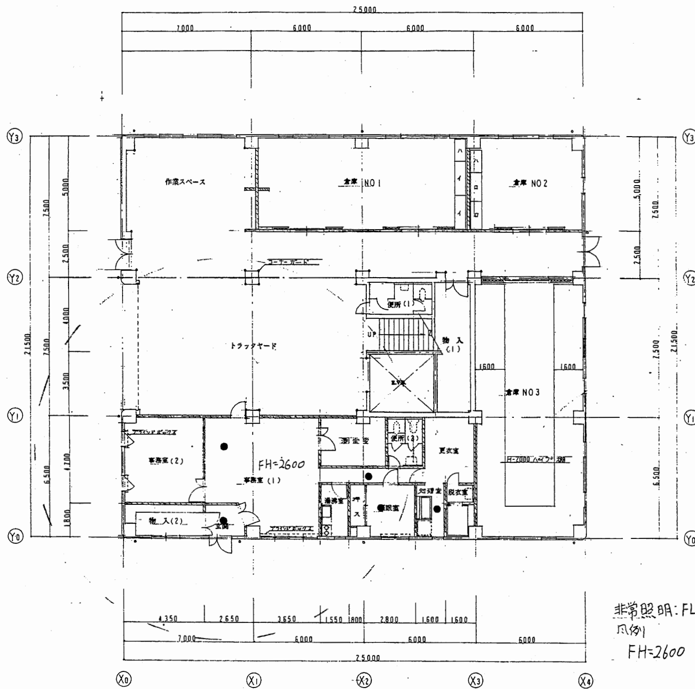
1階平面図 S1:200
