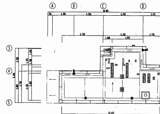
6階屋根伏せ図 S1:300
