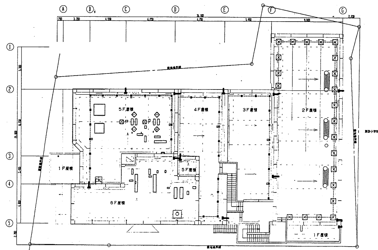
R階平面図 S1:300
