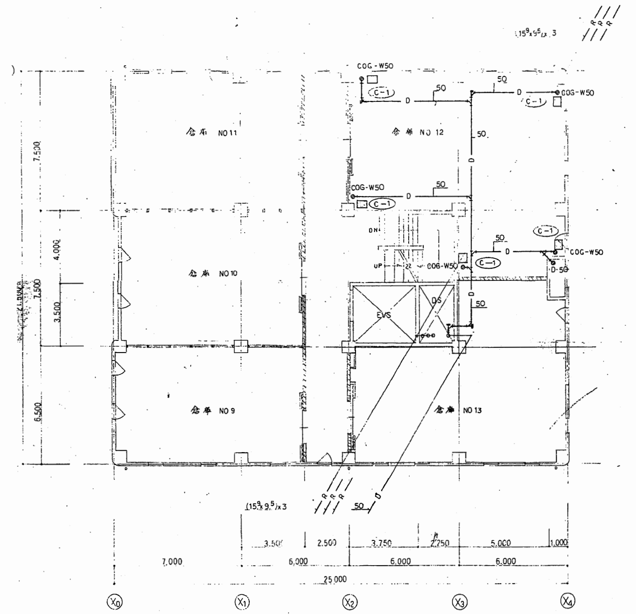
3階平面図 1:100
