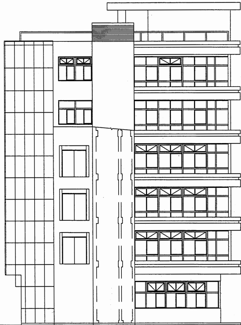
南側立面図
