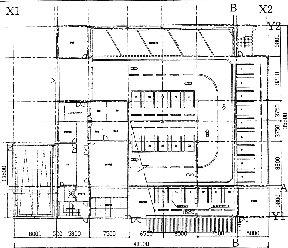
1階平面図 1/300
