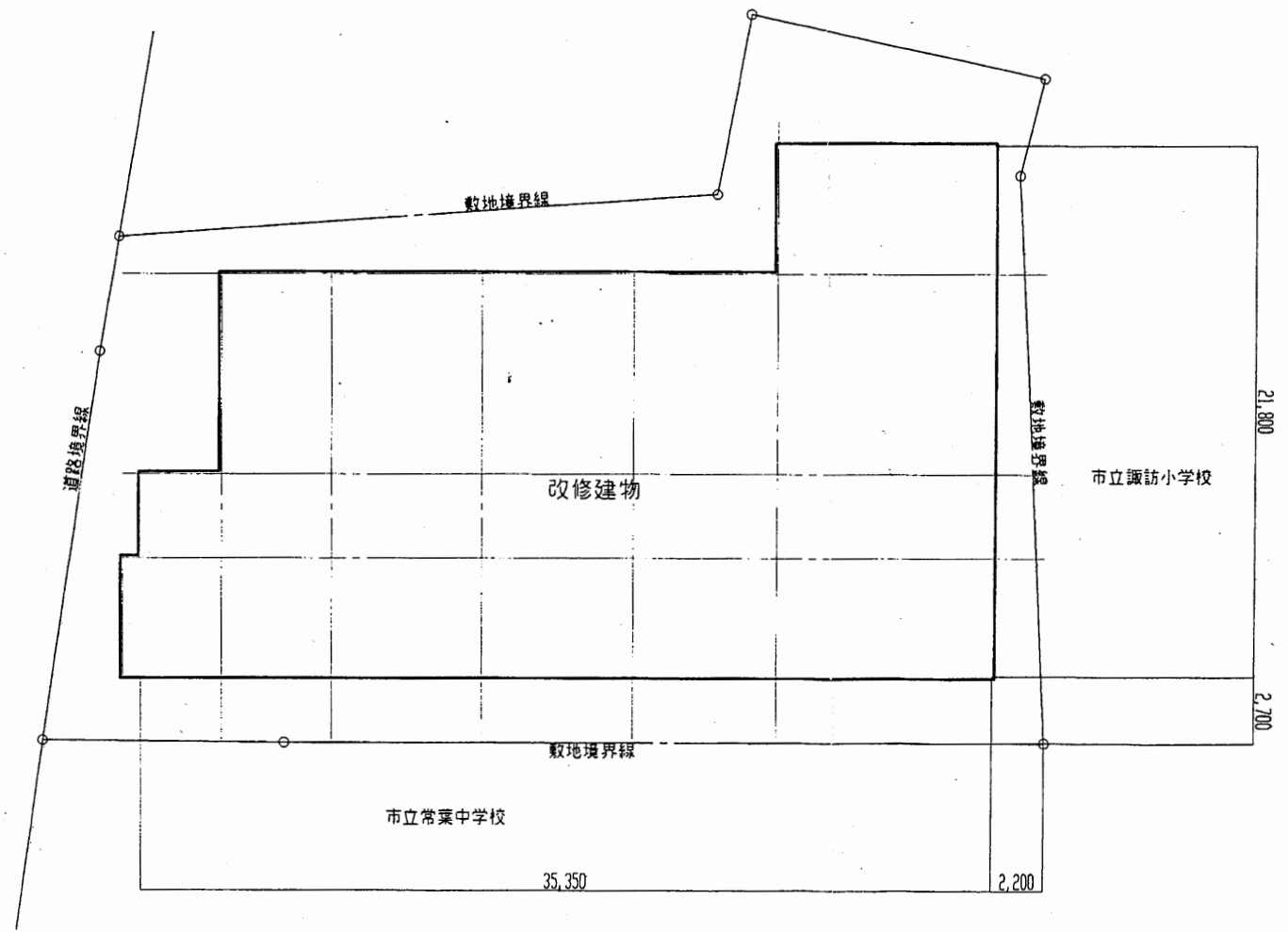
配置図 S=1:300
