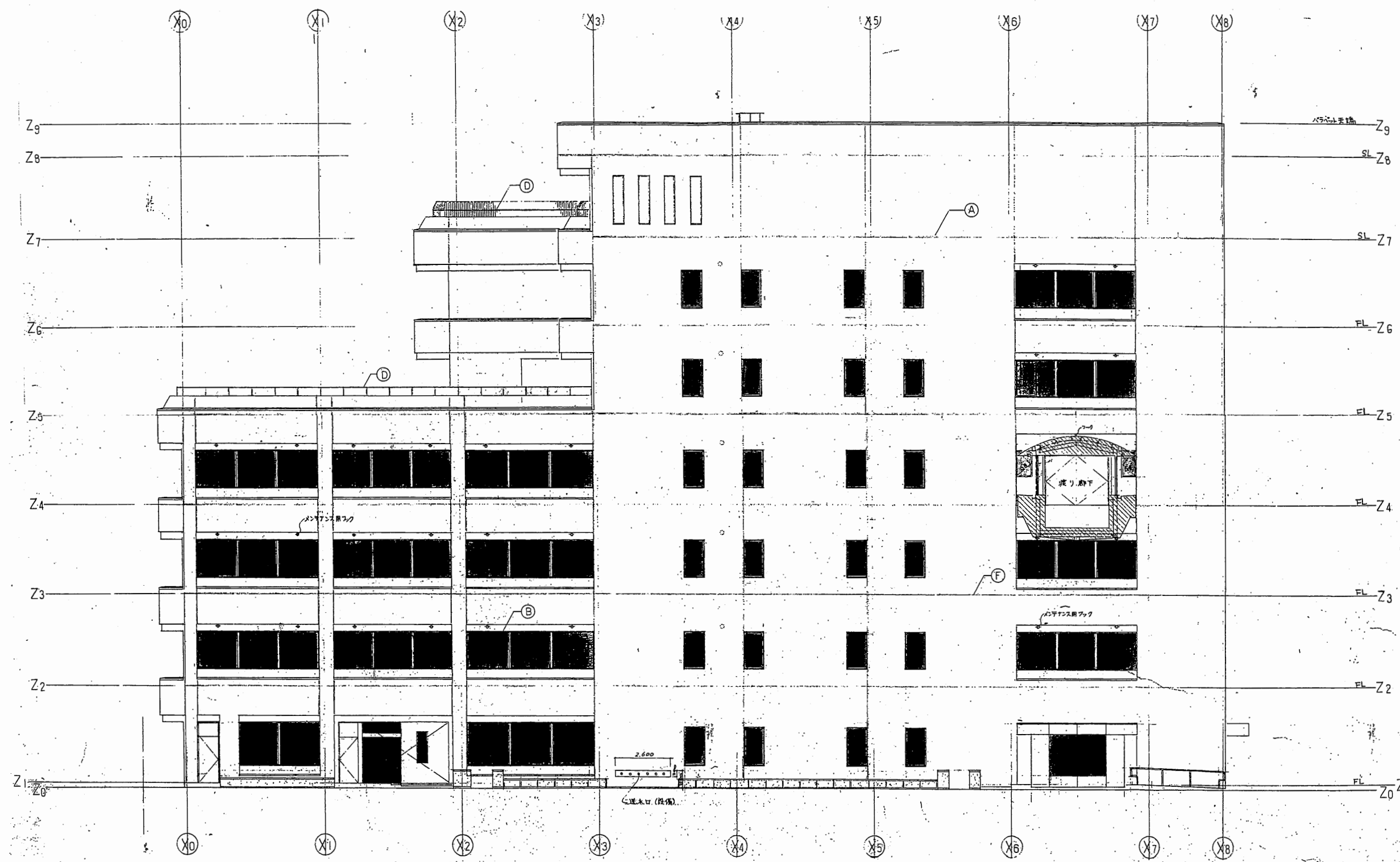
北側立面図 縮尺 1:100
