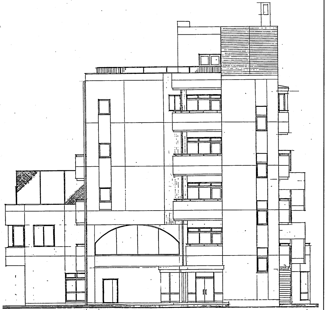
東側立面図
