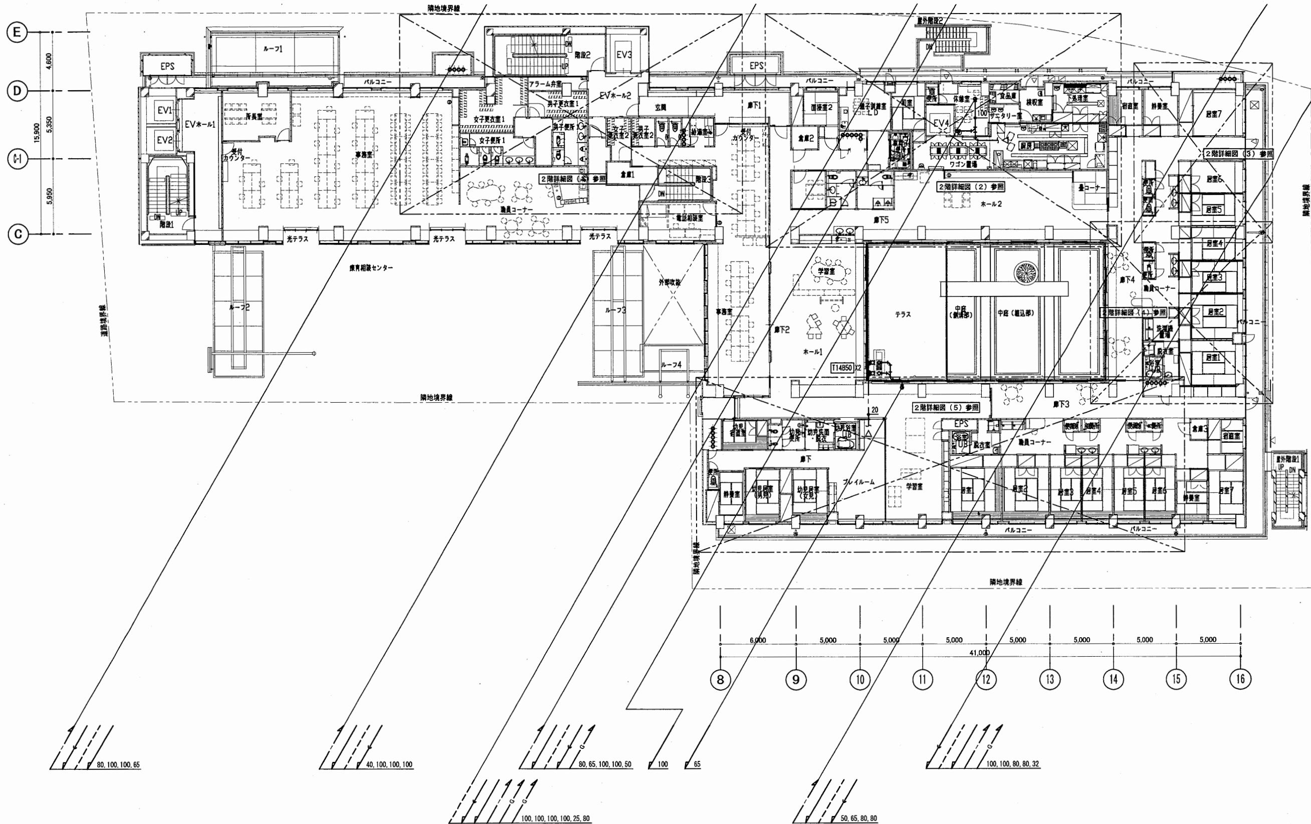
2階平面図
