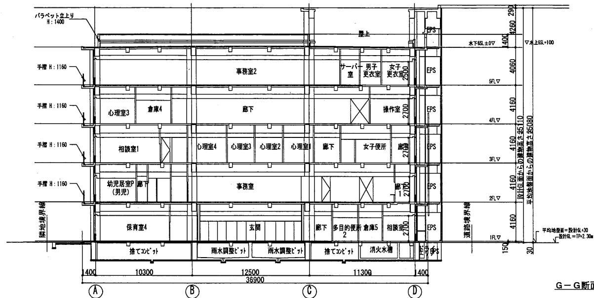
D-D断面
