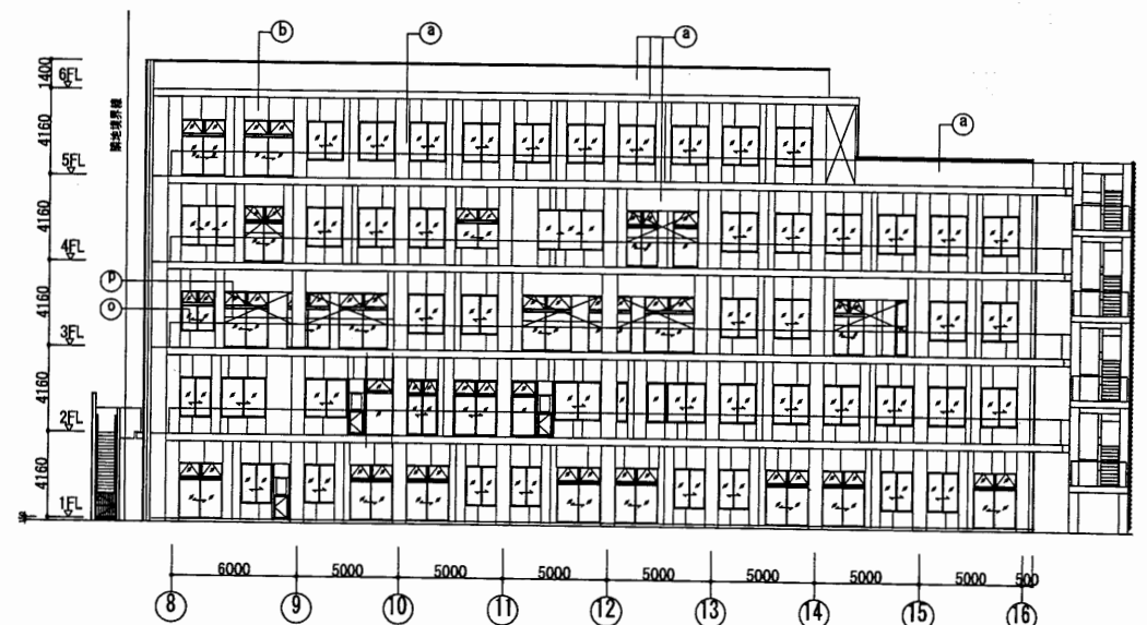
南B立面图
