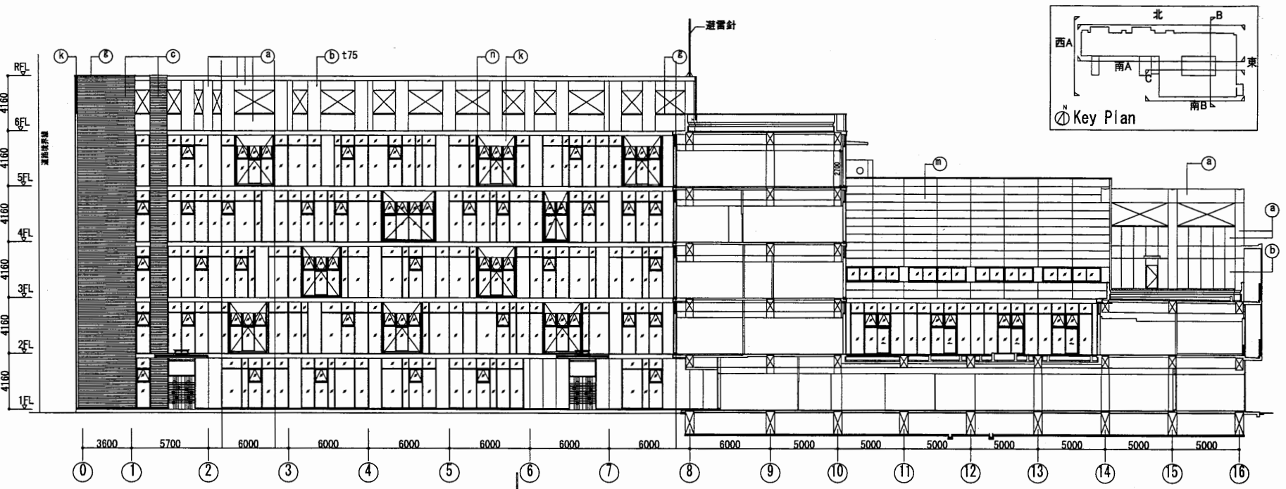
南A立面图
