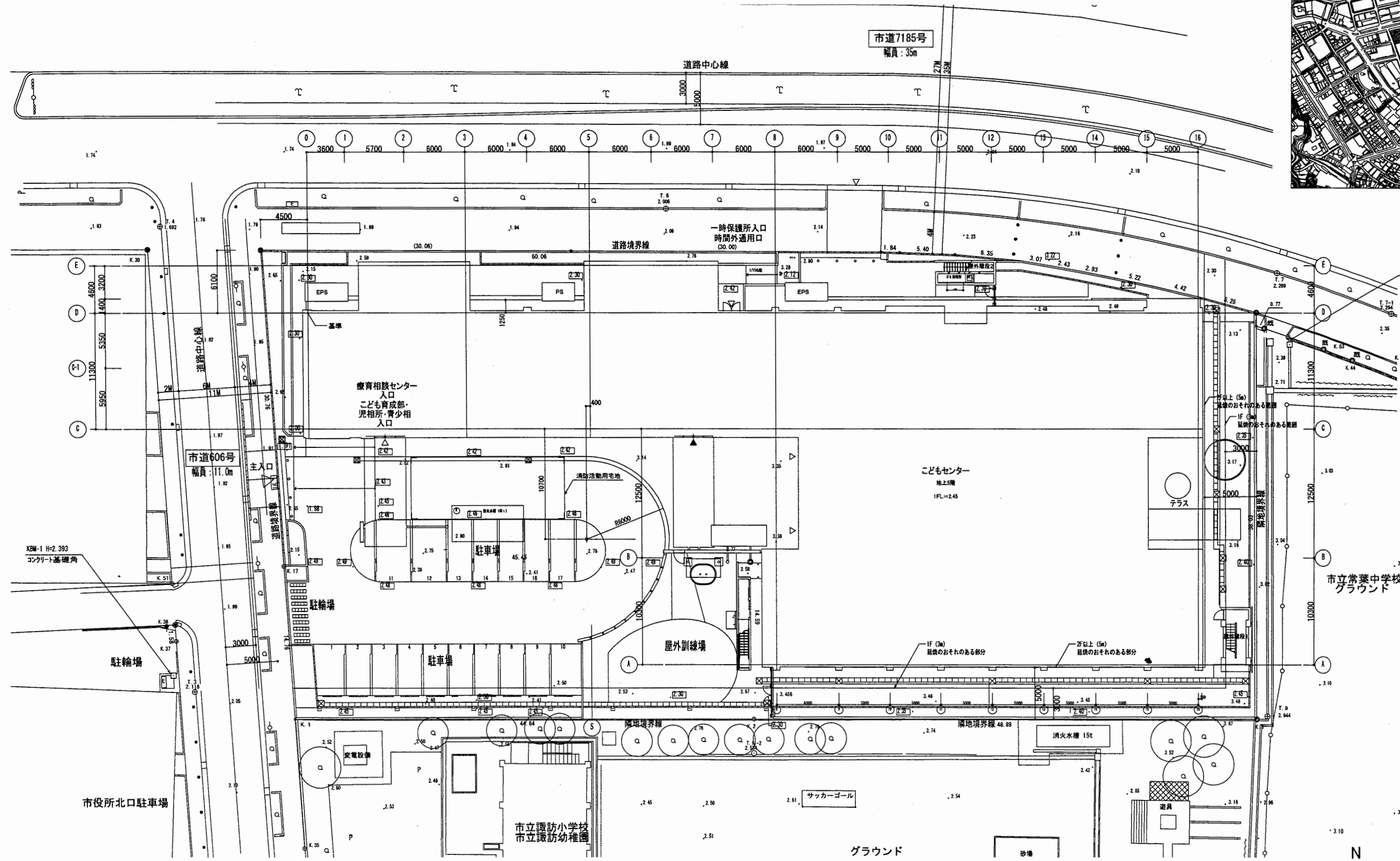
配置図
