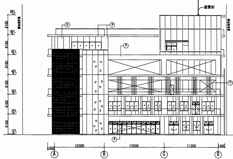
東立面图
