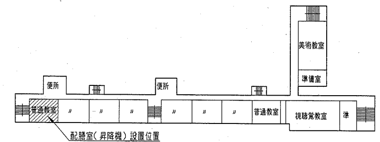
B・C棟3階平面図 1/800
