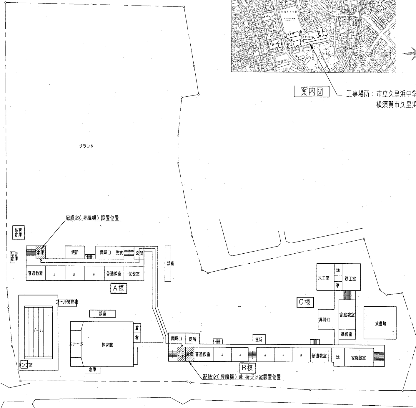
配置図・各棟1階平面図 1/800
