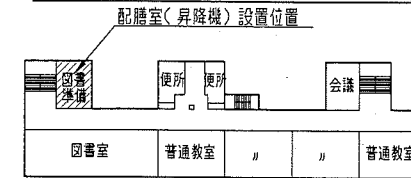
A棟2階平面図 1/800
