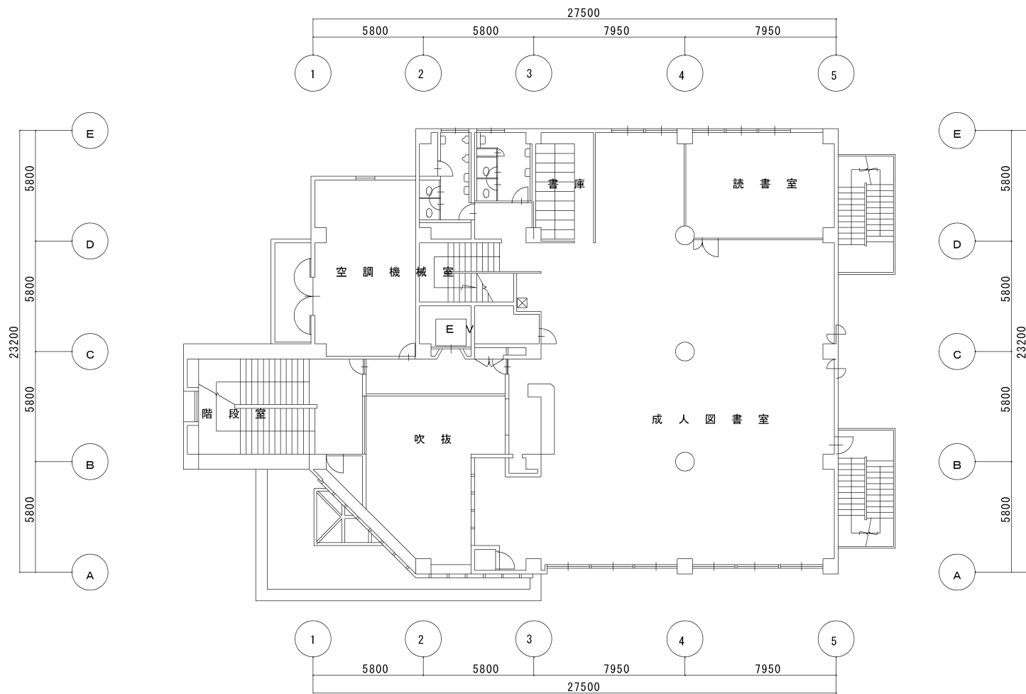
2階平面圖
