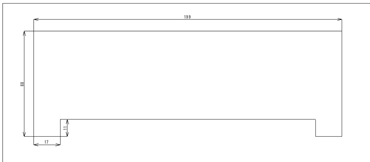
無線機を収納するためのセンターコンソール開口部寸法
